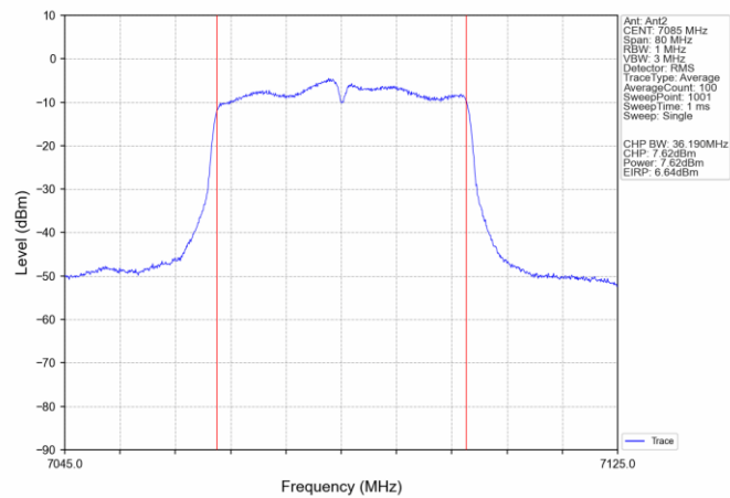
802.11n(HT40) HCH 7085MHz Ant2 NTN
