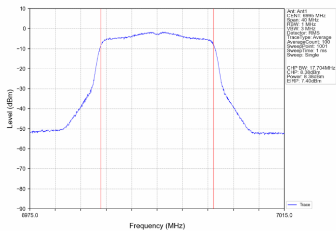
802.11ac(VHT20) MCH_6995MHz_Ant1_NTNV
