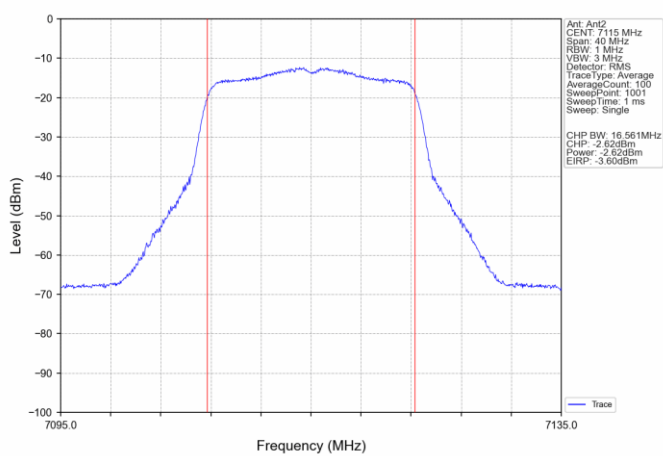
802.11a_HCH_7115MHz_Ant2_NTNV
