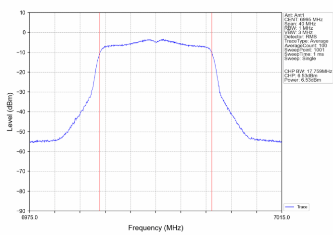
802.11ac(VHT20) MCH_6995MHz_Ant1_NTNV
