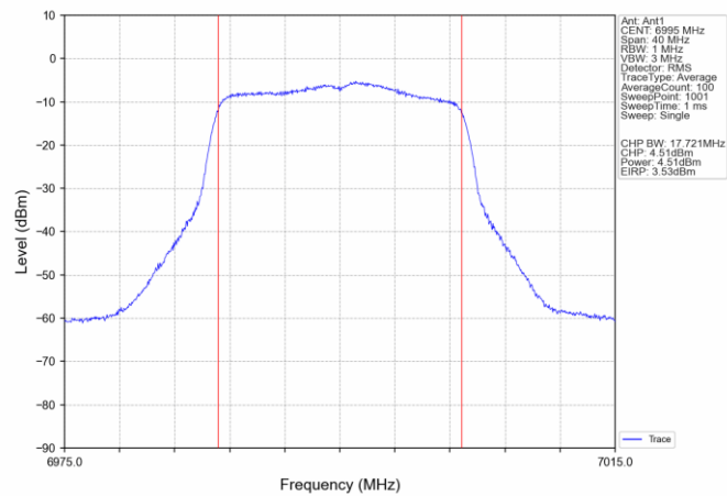
802.11n(HT20)_MCH_6995MHz_Ant1_NTNV
