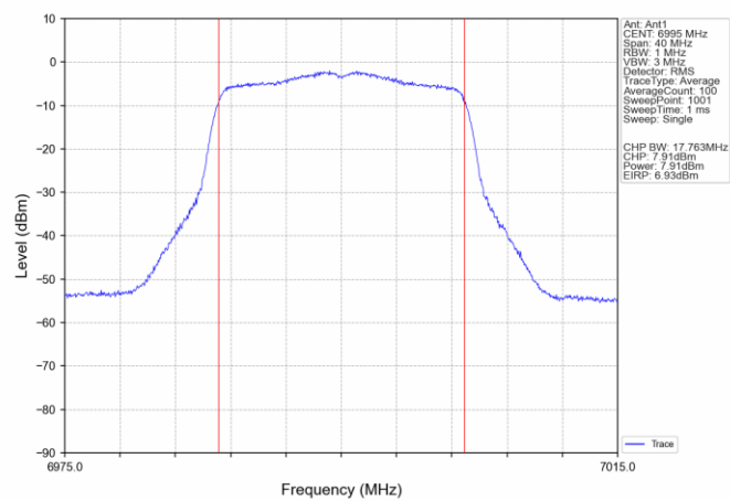
802.11n(HT20)_MCH_6995MHz_Ant1_NTNV
