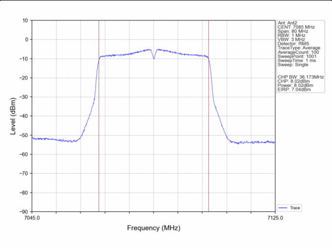
802.11n(HT40) HCH 7085MHz Ant2 NTN
