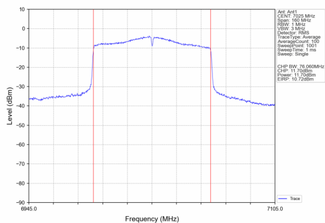
802.11ac(VHT80) HCH_7025MHz_Ant1_NTNV
