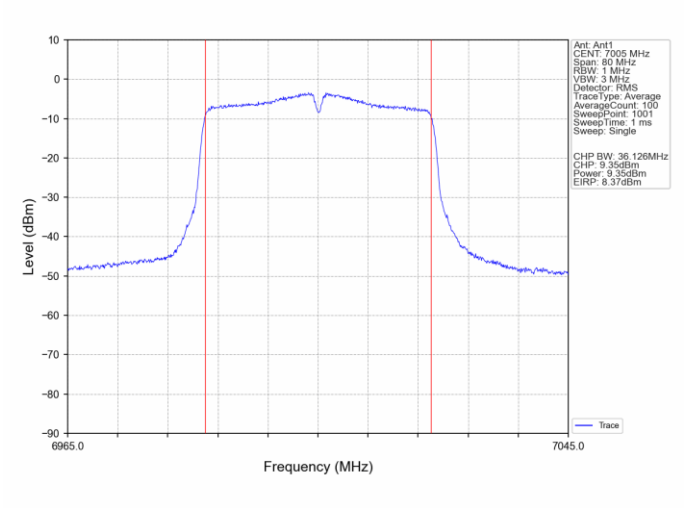
802.11ac(VHT40) MCH_7005MHz_Ant1_NTNV
