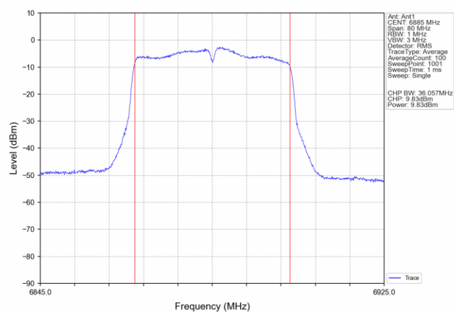
802.11n(HT40)_HCH_6885MHz_Ant1_NTNV
