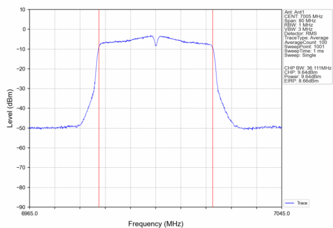
802.11ac(VHT40) MCH_7005MHz_Ant1_NTNV
