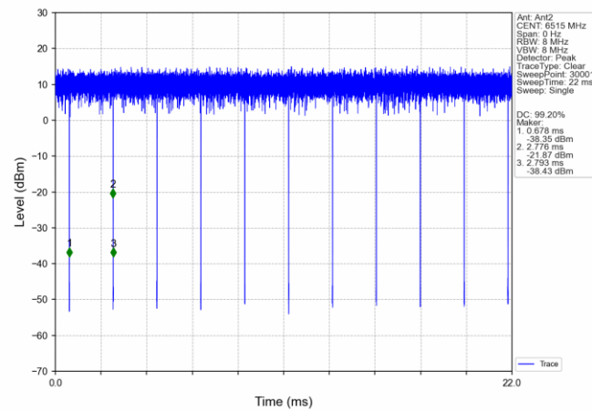
802.11a_HCH_6515MHz_Ant2_NTNV
