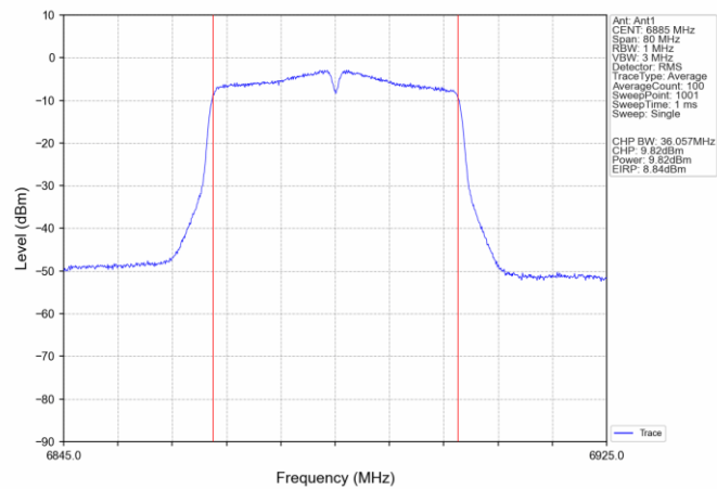
802.11ac(VHT40) HCH 6885MHz Ant1 NTN
