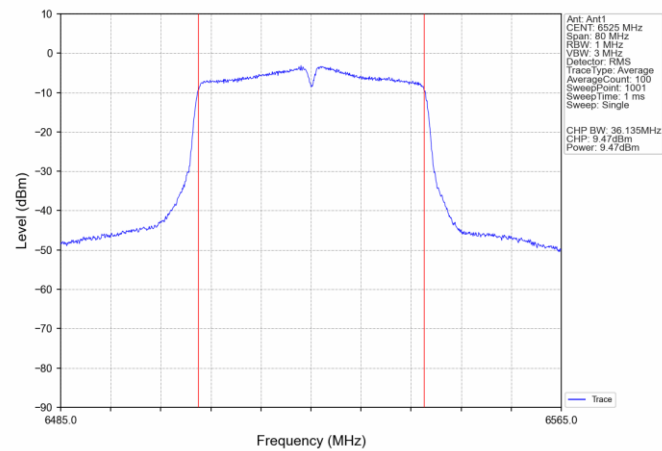
802.11n(HT40) HCH 6525MHz Ant1 NTN
