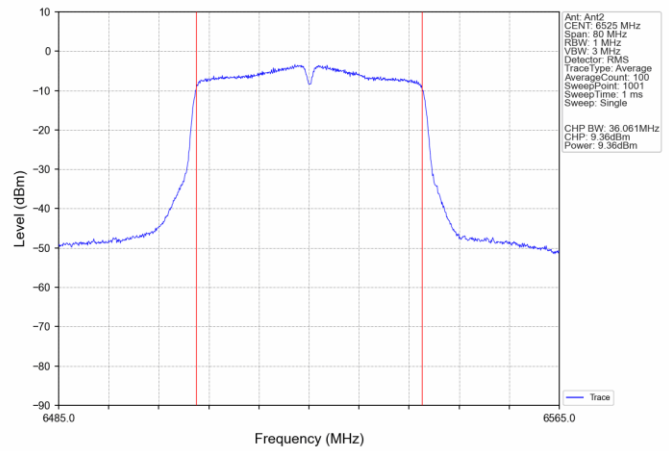
802.11ac(VHT40) HCH 6525MHz Ant2_NTNV
