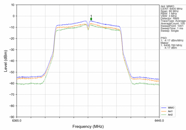
802.11n(HT40) HCH 6405MHz MIMO NTN
