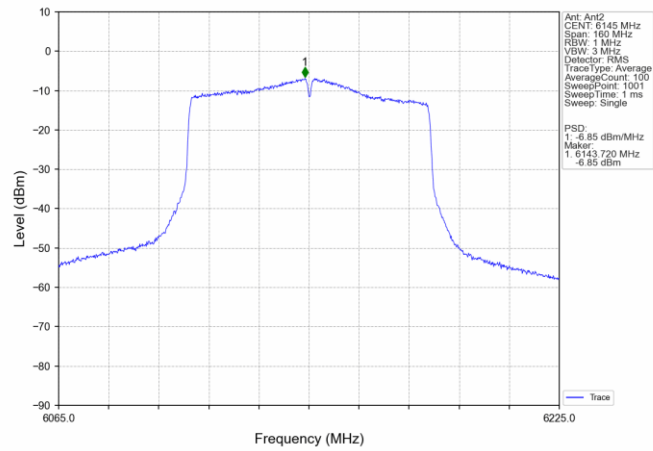
802.11ac(VHT80) MCH 6145MHz MIMO NTN
