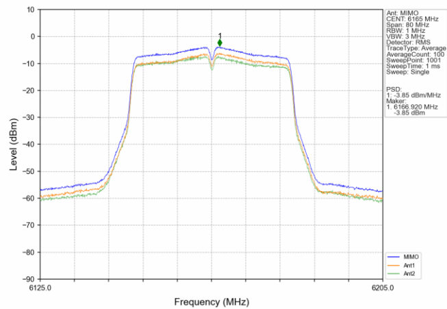
802.11ac(VHT40) MCH 6165MHz MIMO NTN
