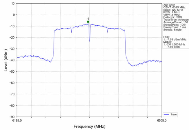
802.11ac(VHT160) HCH 6345MHz MIMO NTN
