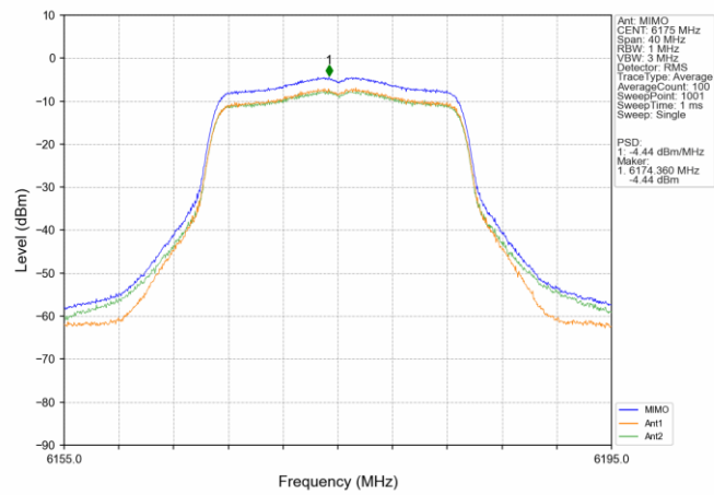
802.11ac(VHT20) MCH 6175MHz MIMO NTN
