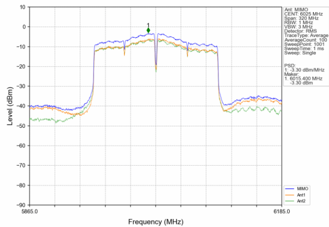
802.11ac(VHT160) LCH 6025MHz MIMO NTN
