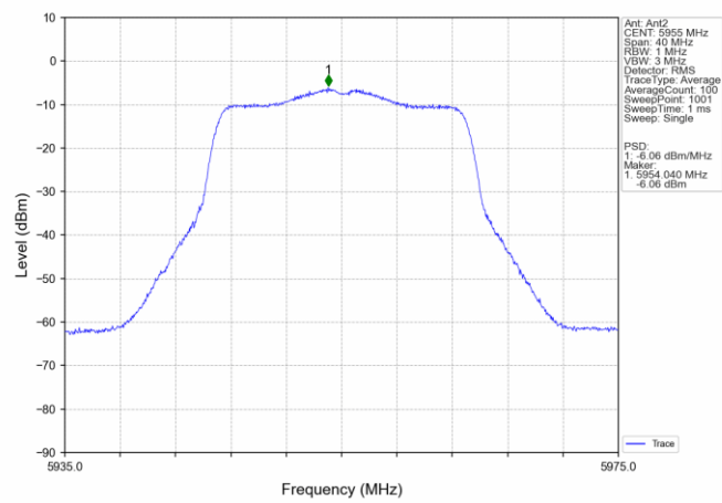
802.11n(HT20) LCH 5955MHz MIMO NTN
