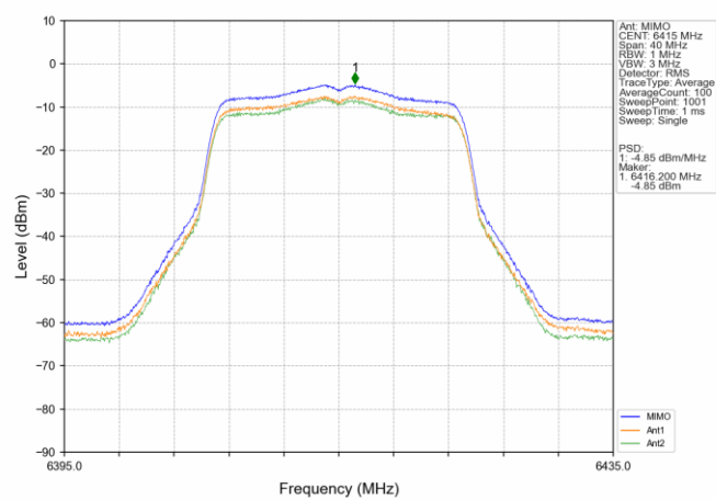
802.11n(HT20) HCH 6415MHz MIMO NTN
