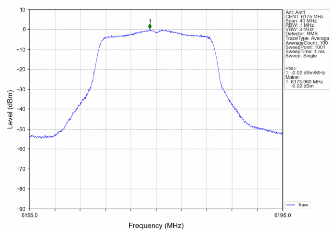
802.11ac(VHT20) MCH_6175MHz_Ant1_NTNV
