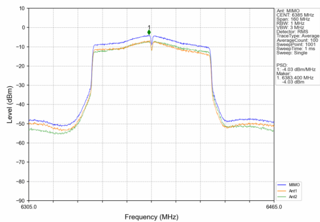
802.11ac(VHT80) HCH 6385MHz MIMO NTN
