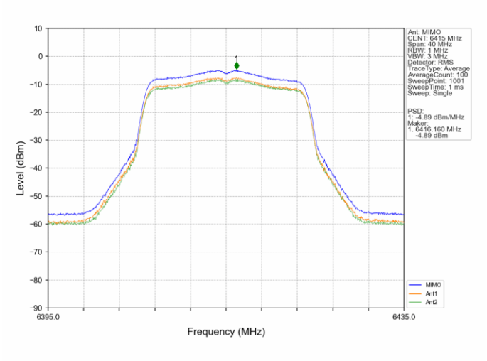
802.11ac(VHT20) HCH 6415MHz MIMO NTN
