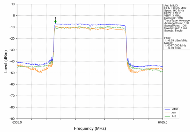
802.11ax(HEW80) HCH_6385MHz_SU / MIMO NTN
