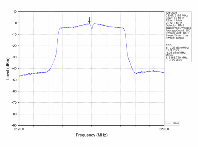
802.11n(HT40) MCH_6165MHz_Ant1_NTNV
