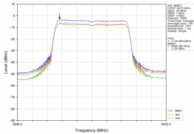
802.11ax(HEW20) HCH 6415MHz SU / MIMO NTN
