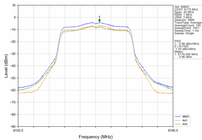
802.11n(HT20) MCH 6175MHz MIMO NTN
