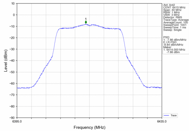
802.11n(HT20)_HCH_6415MHz_MIMO_NTNV
