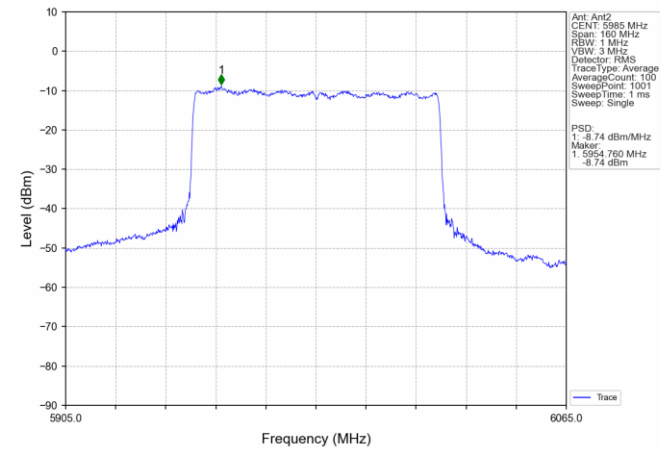
802.11ax(HEW80) LCH_5985MHz_SU / MIMO NTN
