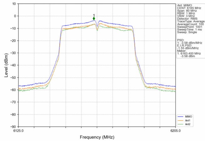
802.11n(HT40) MCH_6165MHz_MIMO_NTNV
