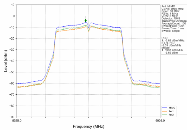
802.11n(HT40) LCH 5965MHz MIMO NTN
