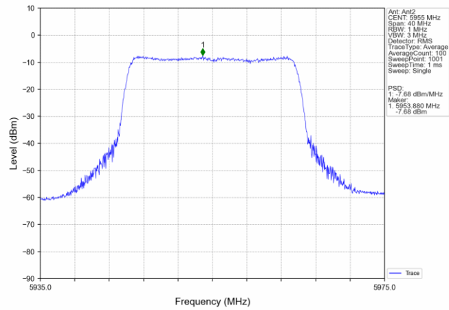
802.11ax(HEW20) LCH_5955MHz_SU / MIMO NTN
