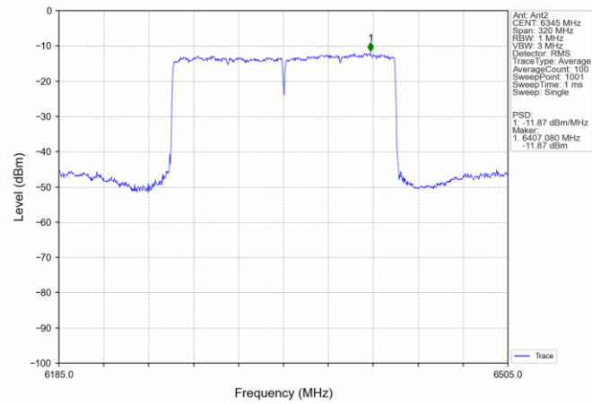
802.11ax(HEW160) HCH 6345MHz SU / MIMO NTN
