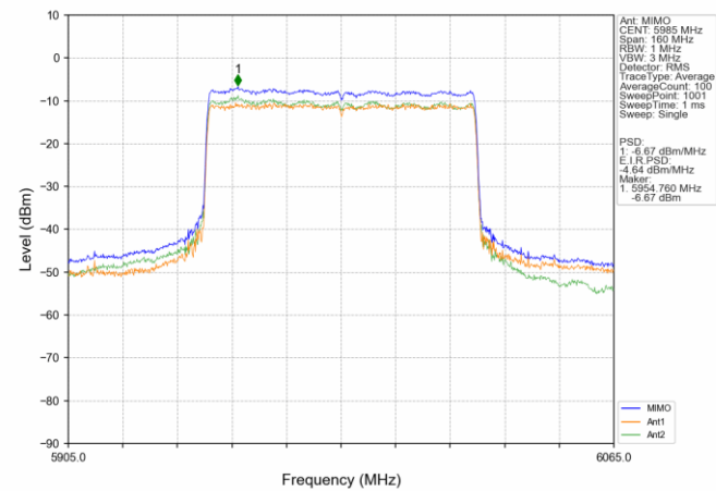
802.11ax(HEW80) LCH_5985MHz_SU / MIMO NTN
