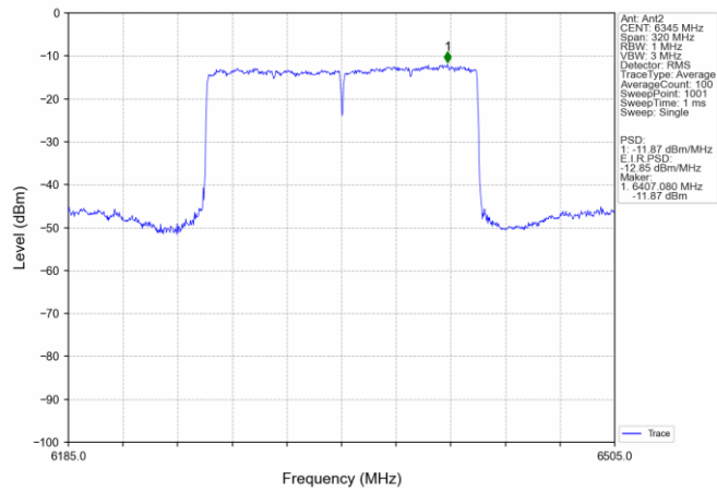
802.11ax(HEW160) HCH 6345MHz SU / MIMO NTN
