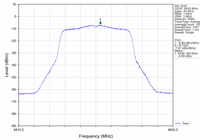
802.11ac(VHT20) LCH 6435MHz Ant2 NTN
