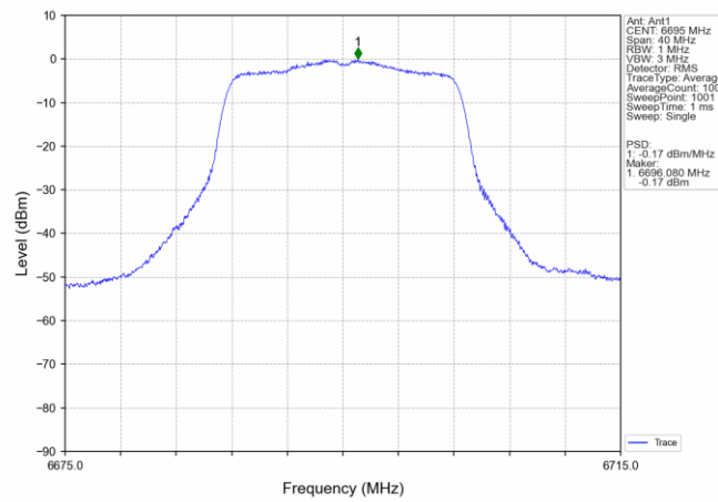
802.11a_MCH_6695MHz_Ant1_NTNV
