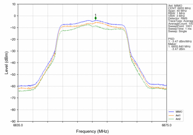
802.11n(HT20) HCH 6855MHz MIMO NTN
