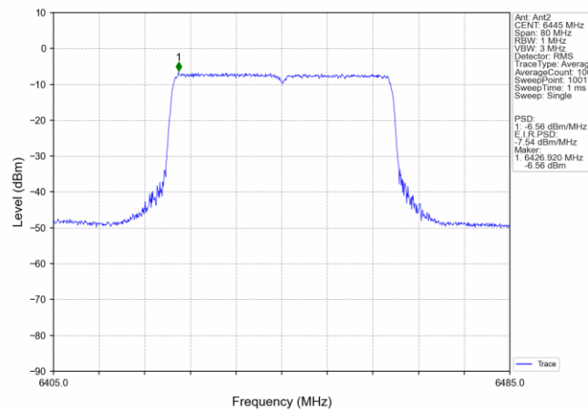
802.11ax(HEW40) LCH 6445MHz SU / Ant2 NTN
