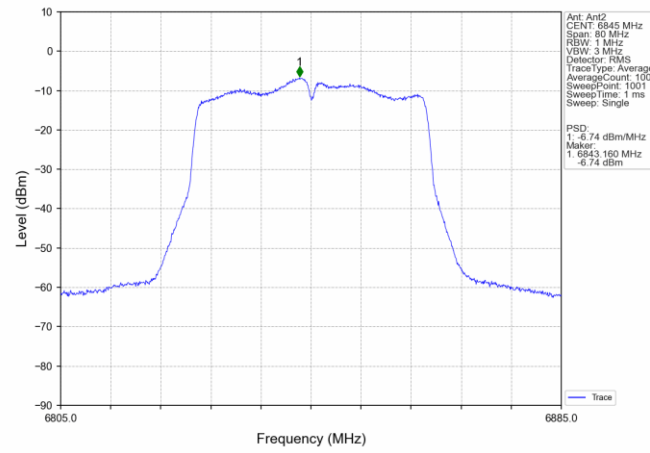
802.11n(HT40) HCH 6845MHz MIMO NTN
