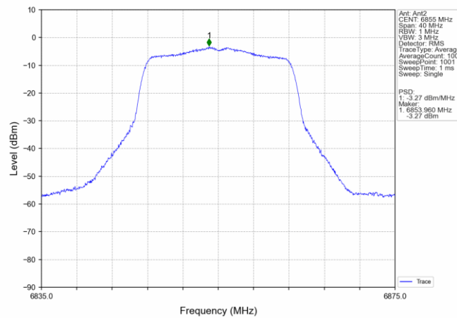
802.11a_HCH_6855MHz_Ant2_NTNV
