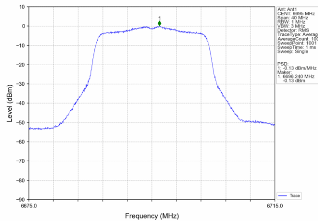
802.11n(HT20) MCH_6695MHz_Ant1_NTNV
