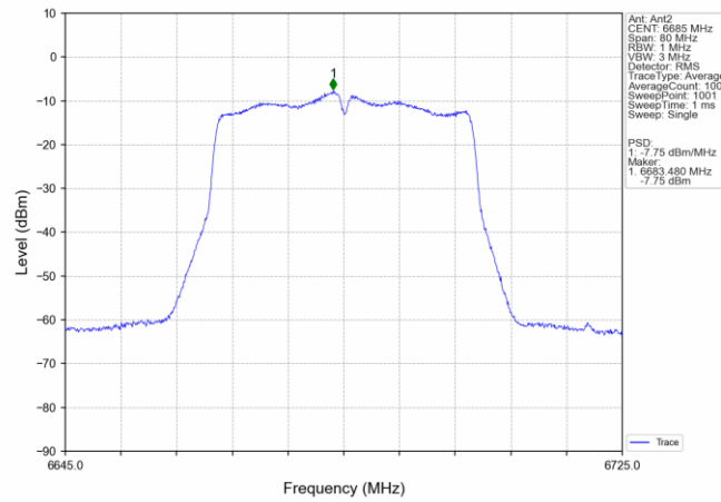
802.11n(HT40) MCH_6685MHz_MIMO_NTNV
