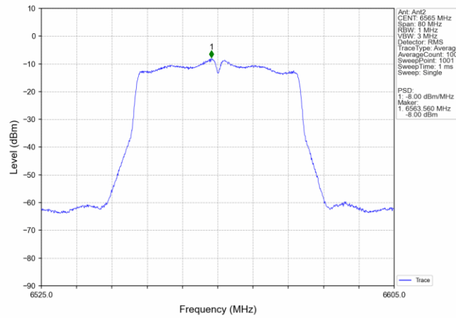
802.11n(HT40) LCH 6565MHz MIMO NTN
