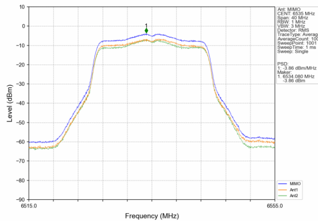
802.11n(HT20) LCH 6535MHz MIMO NTN
