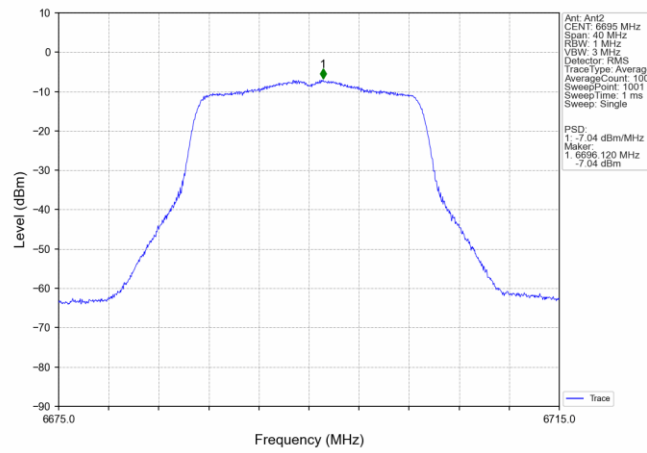
802.11ac(VHT20) MCH 6695MHz MIMO NTN
