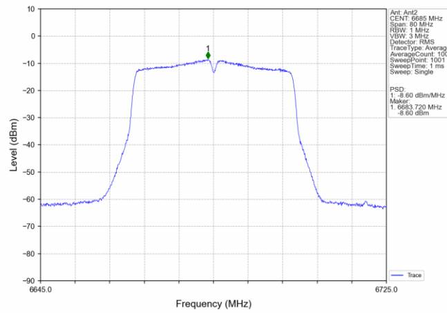
802.11ac(VHT40) MCH 6685MHz MIMO NTN
