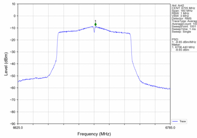
802.11ac(VHT80) MCH 6705MHz MIMO NTN
