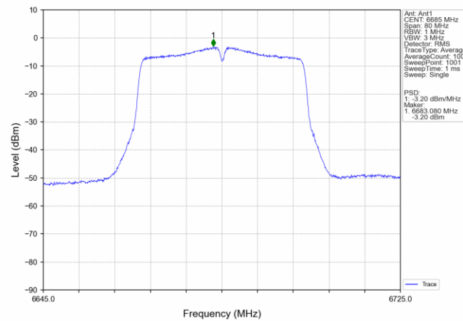
802.11ac(VHT40) MCH_6685MHz_Ant1_NTNV
