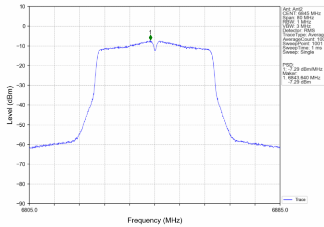
802.11ac(VHT40) HCH 6845MHz MIMO NTN
