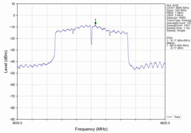
802.11ac(VHT160) MCH_6665MHz_MIMO_NTNV
