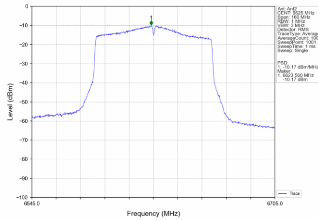
802.11ac(VHT80) LCH 6625MHz MIMO NTN
