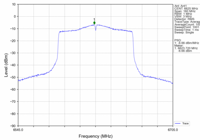
802.11ac(VHT80) LCH 6625MHz Ant1 NTN
