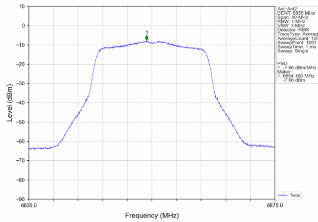
802.11ac(VHT20) HCH 6855MHz MIMO NTN
