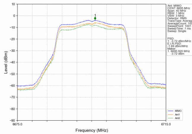
802.11n(HT20) MCH 6695MHz MIMO NTN
