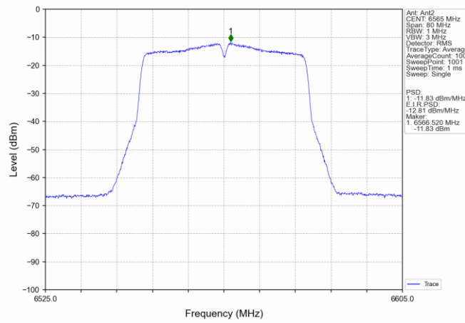
802.11ac(VHT40) LCH_6565MHz_MIMO_NTNV
