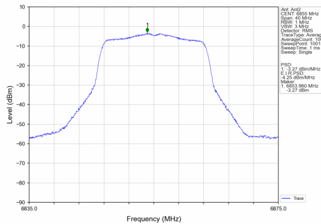
802.11a_HCH_6855MHz_Ant2_NTNV
