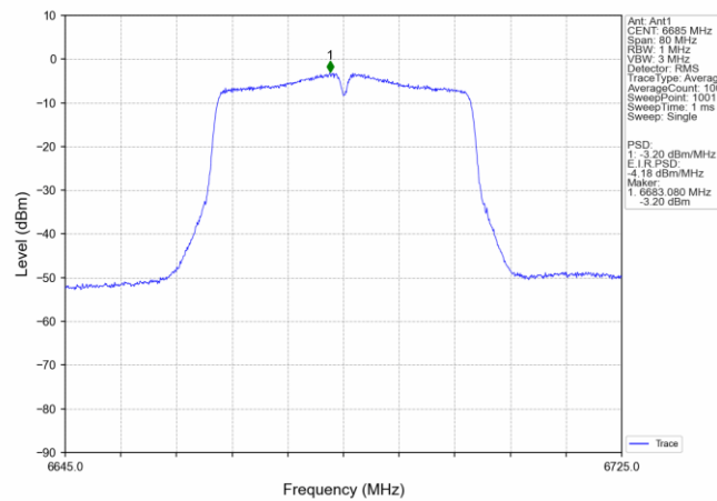
802.11ac(VHT40) MCH_6685MHz_Ant1_NTNV
