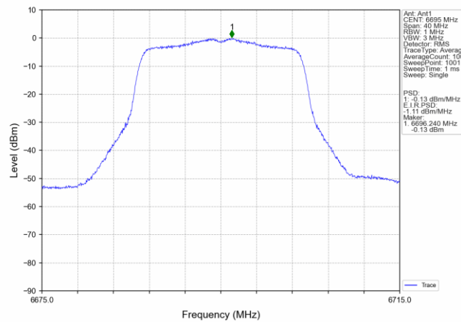
802.11n(HT20) MCH_6695MHz_Ant1_NTNV
