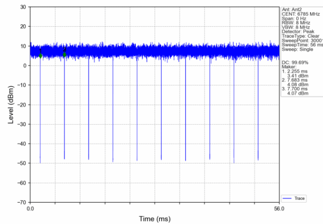
802.11ac(VHT80) HCH_6785MHz_Ant2_NTNV
