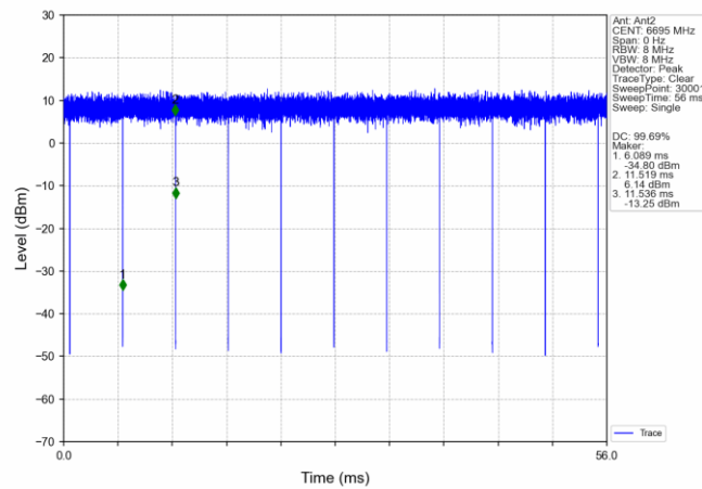
802.11ac(VHT20) MCH_6695MHz_Ant2_NTNV
