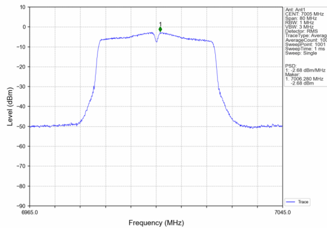
802.11n(HT40) MCH_7005MHz_Ant1_NTNV
