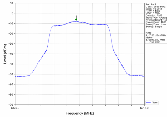
802.11n(HT20) LCH 6895MHz MIMO NTN
