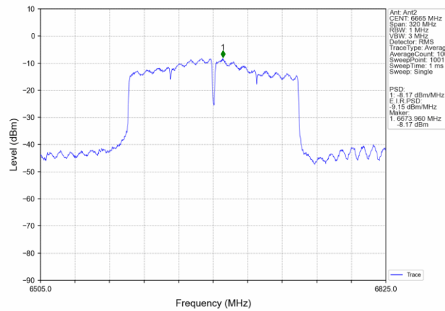
802.11ac(VHT160) MCH_6665MHz_MIMO_NTNV
