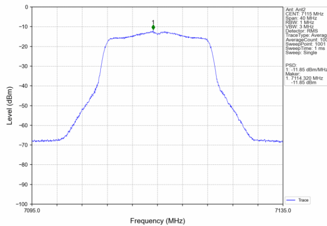
802.11a_HCH_7115MHz_Ant2_NTNV
