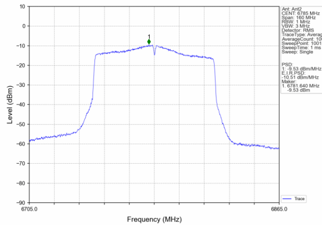
802.11ac(VHT80) HCH 6785MHz MIMO NTN
