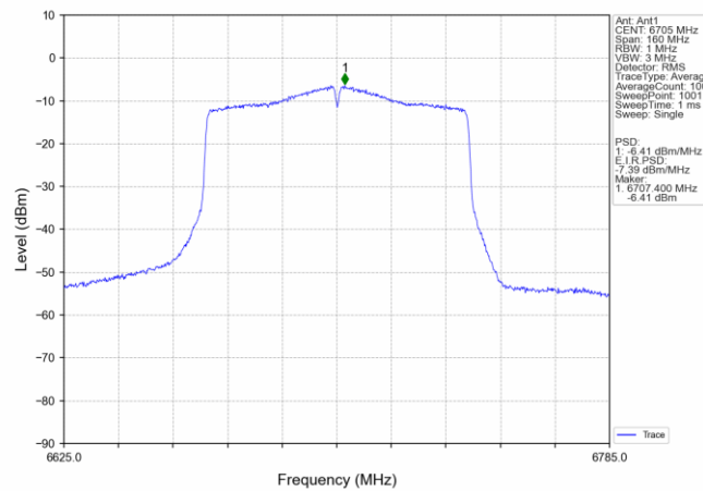
802.11ac(VHT80) MCH_6705MHz_Ant1_NTNV
