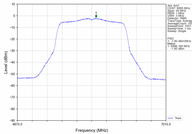
802.11n(HT20) MCH 6995MHz Ant1 NTN
