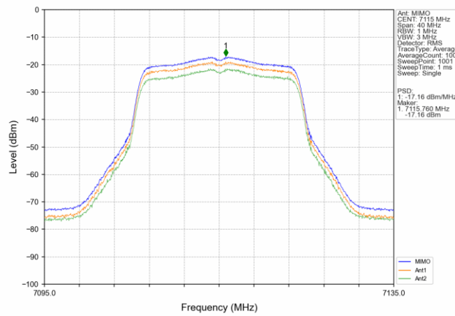
802.11ac(VHT20) HCH 7115MHz MIMO NTN
