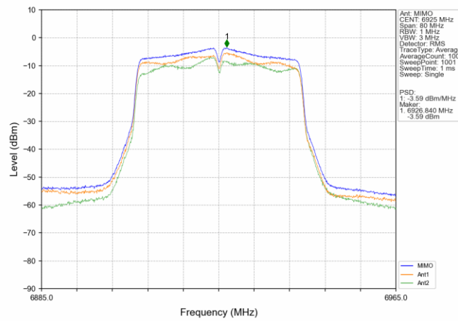
802.11n(HT40) LCH 6925MHz MIMO NTN
