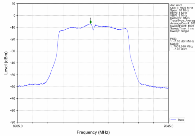
802.11n(HT40) MCH 7005MHz MIMO_NTNV
