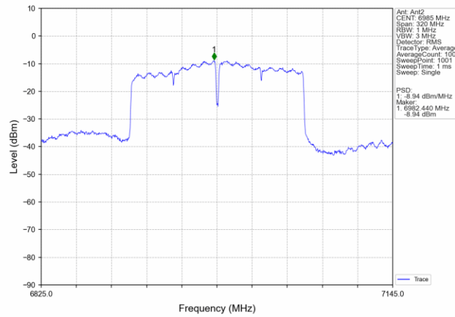
802.11ac(VHT160) MCH_6985MHz_MIMO_NTNV
