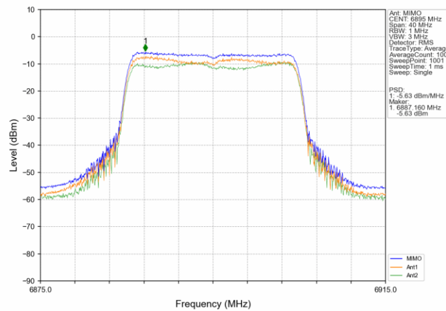
802.11ax(HEW20) LCH 6895MHz SU / MIMO NTN
