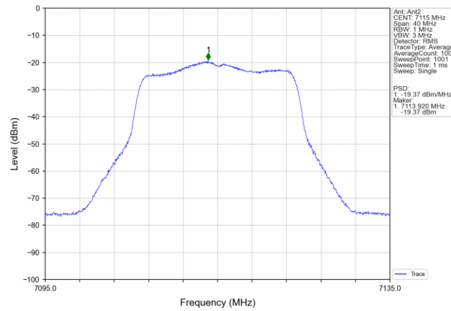
802.11n(HT20) HCH 7115MHz MIMO NTN
