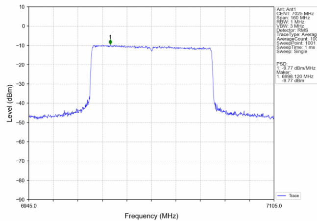
802.11ax(HEW80) HCH 7025MHz SU / Ant1 NTN
