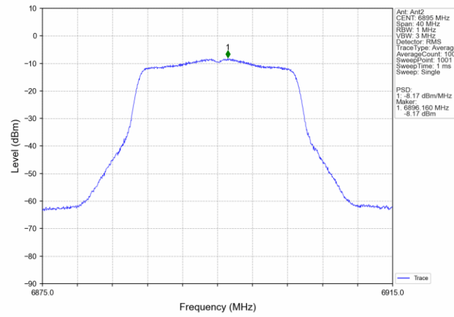
802.11ac(VHT20) LCH_6895MHz_MIMO_NTNV
