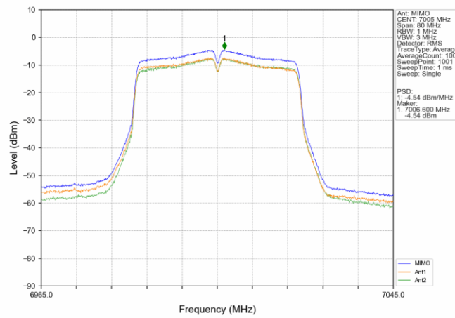
802.11ac(VHT40) MCH 7005MHz MIMO NTN
