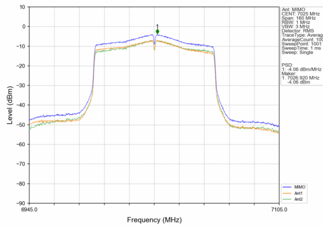
802.11ac(VHT80) HCH 7025MHz MIMO NTN
