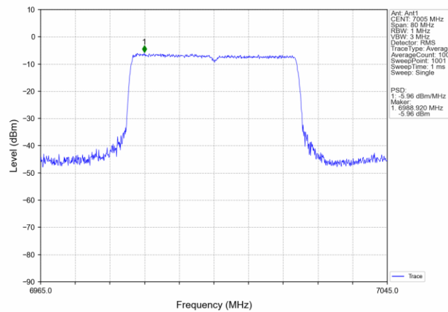
802.11ax(HEW40) MCH 7005MHz SU / Ant1 NTN
