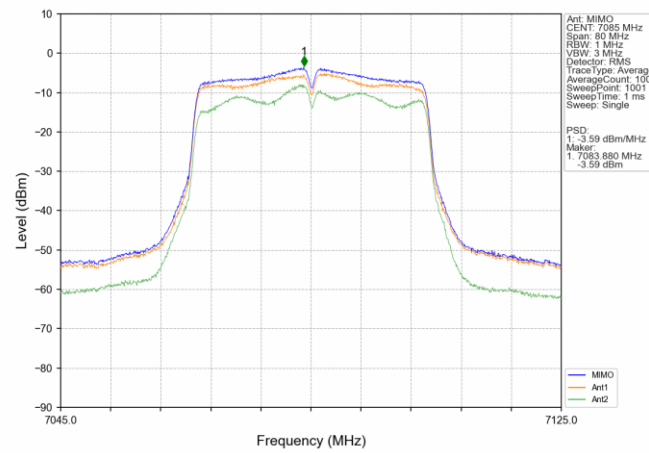
802.11n(HT40) HCH 7085MHz MIMO NTN
