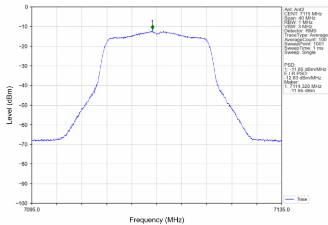
802.11a_HCH_7115MHz_Ant2_NTNV
