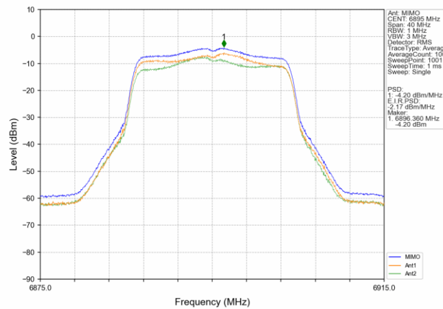
802.11n(HT20)_LCH_6895MHz_MIMO_NTNV
