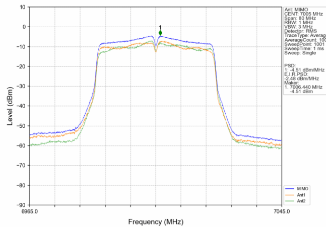
802.11n(HT40) MCH 7005MHz MIMO NTN
