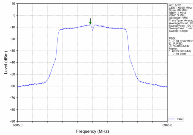
802.11ac(VHT40) LCH_6925MHz_MIMO_NTNV
