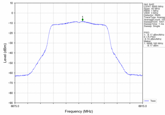
802.11ac(VHT20) LCH 6895MHz MIMO NTN
