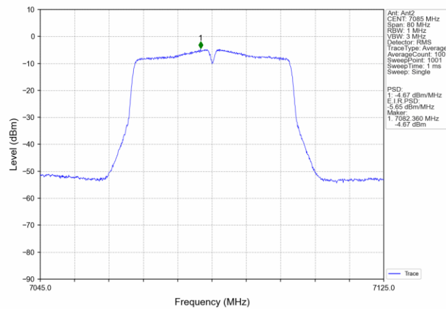
802.11ac(VHT40) HCH_7085MHz_Ant2_NTNV
