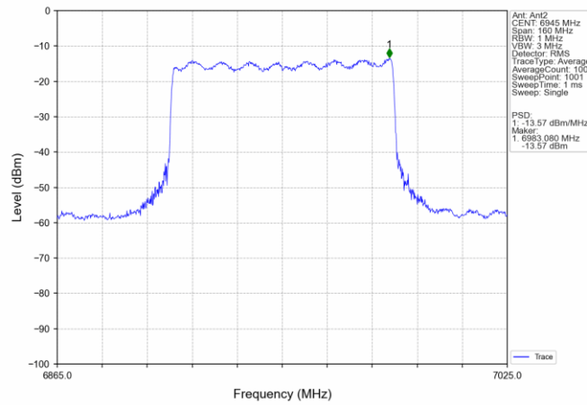
802.11ax(HEW80) LCH 6945MHz SU / MIMO NTN
