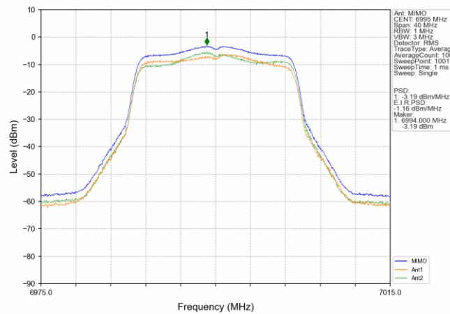
802.11n(HT20) MCH_6995MHz_MIMO_NTNV
