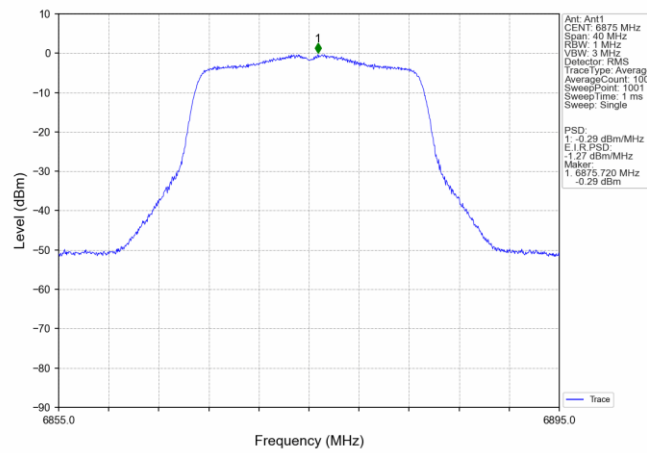
802.11n(HT20)_HCH_6875MHz_Ant1_NTNV
