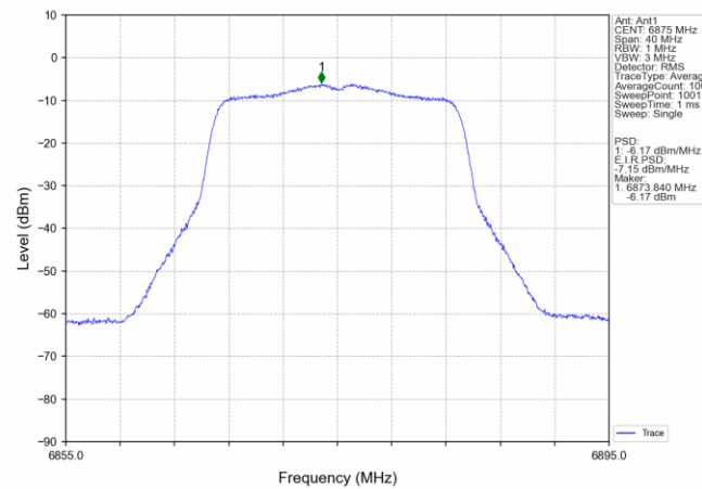
802.11ac(VHT20) HCH 6875MHz Ant1_NTNV
