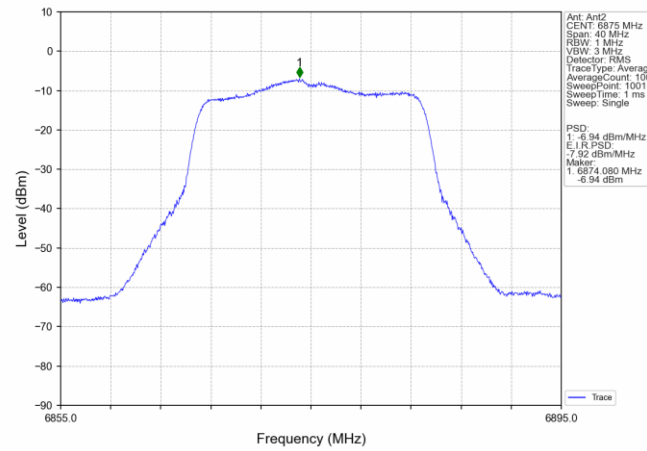
802.11n(HT20)_HCH_6875MHz_MIMO_NTNV
