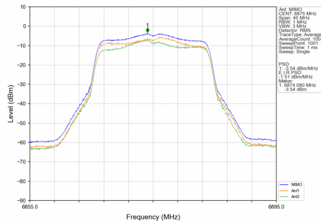
802.11n(HT20)_HCH_6875MHz_MIMO_NTNV
