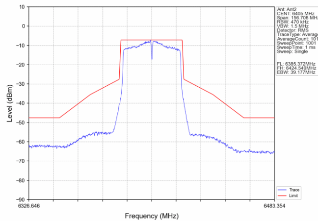
802.11ac(VHT40) HCH 6405MHz Ant2 NTN
