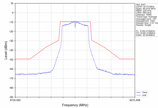
802.11ac(VHT20) MCH_6175MHz_Ant1_NTNV
