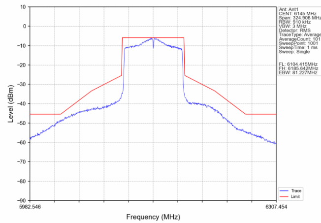
802.11ac(VHT80) MCH_6145MHz_Ant1_NTNV
