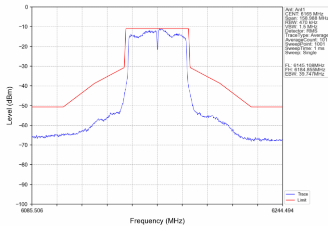
802.11n(HT40)_MCH_6165MHz_Ant1_NTNV
