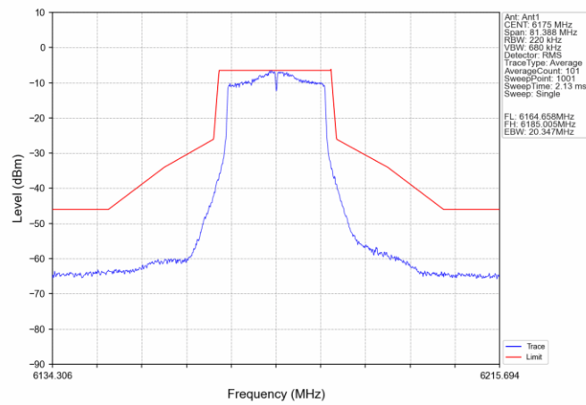
802.11ac(VHT20) MCH_6175MHz_Ant1_NTNV
