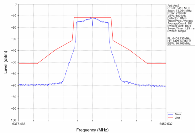
802.11a_HCH_6415MHz_Ant2_NTNV
