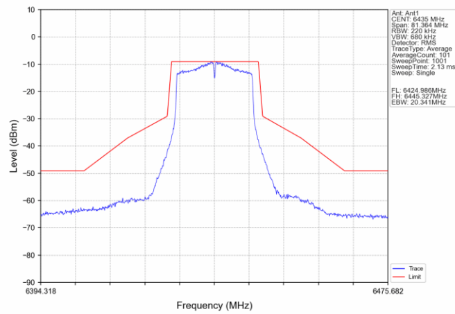
802.11ac(VHT20)_LCH_6435MHz_Ant1_NTNV
