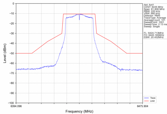
802.11ac(VHT20) LCH_6435MHz_Ant1_NTNV
