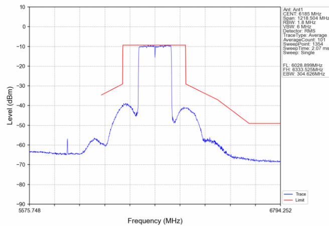
802.11ax(HEW160) MCH 6185MHz_SU / Ant1 NTN
