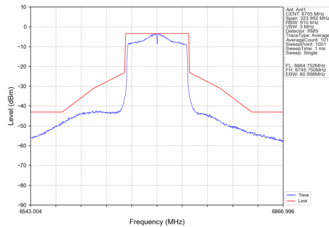
802.11ac(VHT80) MCH_6705MHz_Ant1_NTNV
