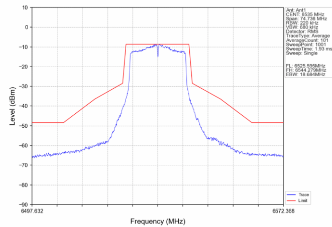
802.11a LCH 6535MHz Ant1 NTN
