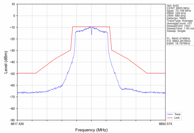
802.11a_HCH_6855MHz_Ant2_NTNV
