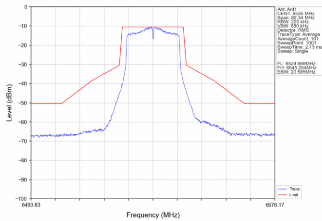
802.11ac(VHT20) LCH_6535MHz_Ant1_NTNV
