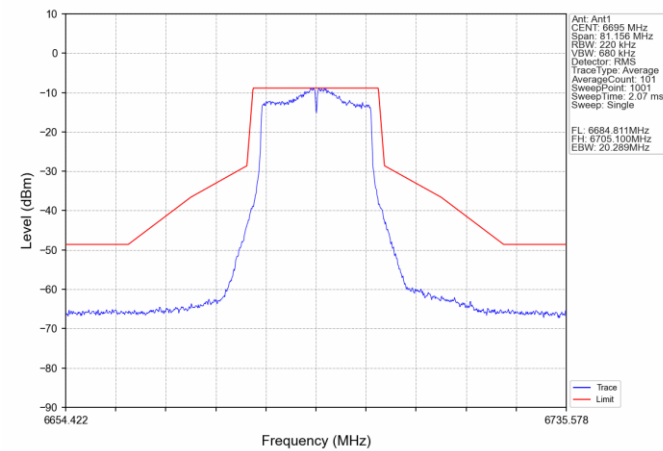
802.11n(HT20) MCH_6695MHz_Ant1_NTNV
