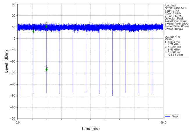
802.11ac(VHT40) HCH_7085MHz_Ant1_NTNV
