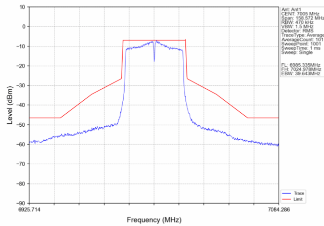
802.11ac(VHT40) MCH_7005MHz_Ant1_NTNV
