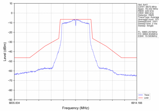
802.11n(HT20)_HCH_6875MHz_Ant1_NTNV
