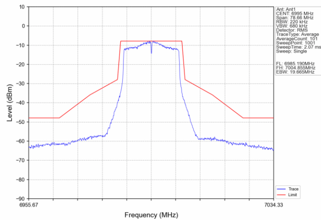
802.11ac(VHT20) MCH_6995MHz_Ant1_NTNV
