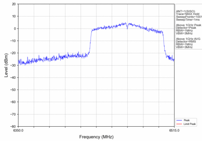
802.11ac(VHT80) LCH_6465MHz_Ant1_NTNV
