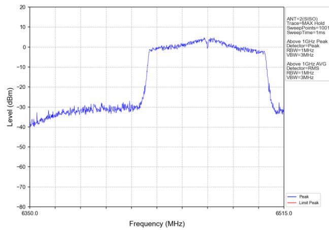
802.11ac(VHT80) LCH_6465MHz_Ant2_NTNV
