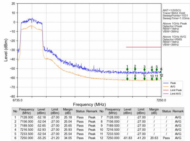
802.11ac(VHT80) HCH_6785MHz_Ant1_NTNV
