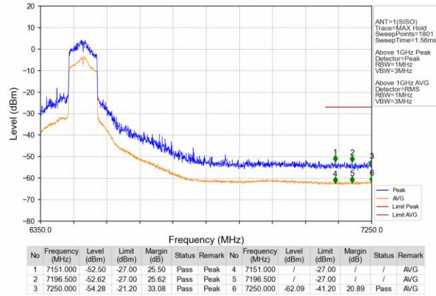
802.11ac(VHT80) LCH_6465MHz_Ant1_NTNV
