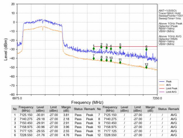
802.11ac(VHT80) HCH_7025MHz_Ant1_NTNV
