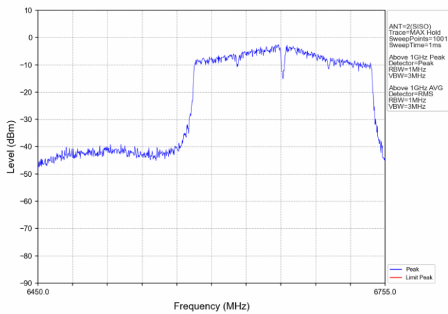
802.11ac(VHT160) MCH_6665MHz_Ant2_NTNV
