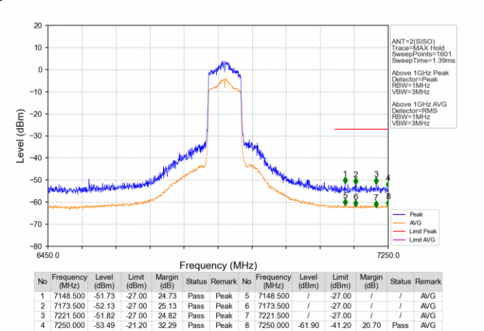
802.11ac(VHT80) HCH 6865MHz Ant2 NTN
