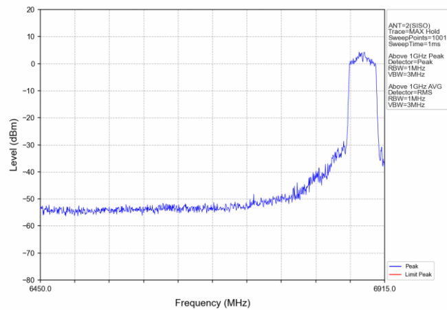
802.11ac(VHT40) HCH_6885MHz_Ant2_NTNV
