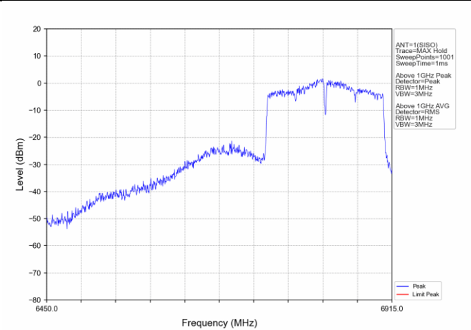
802.11ac(VHT160) HCH 6825MHz Ant1 NTN
