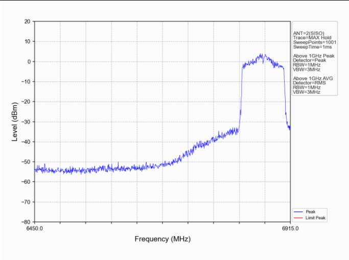
802.11ac(VHT80) HCH 6865MHz Ant2 NTN
