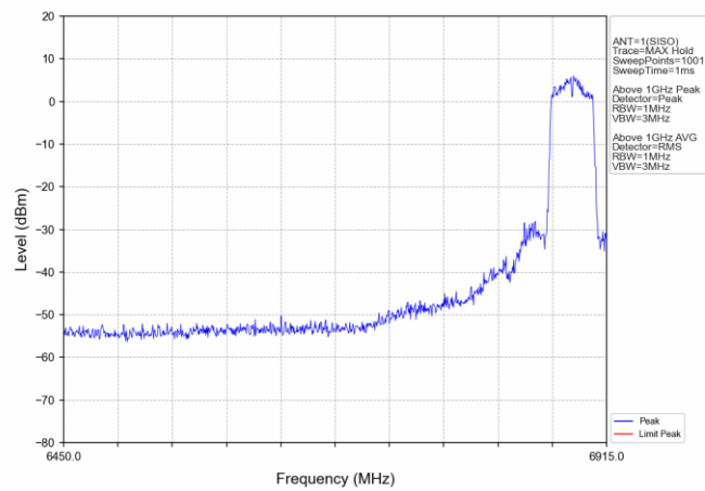
802.11ac(VHT40) HCH_6885MHz_Ant1_NTNV
