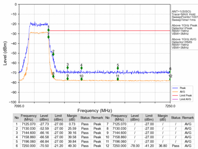
802.11ax(HEW20) HCH 7115MHz SU / Ant1 NTN
