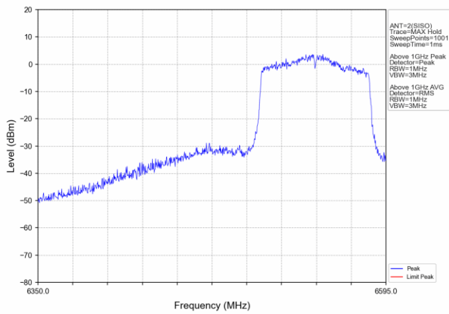
802.11ac(VHT80) HCH_6545MHz_Ant2_NTNV
