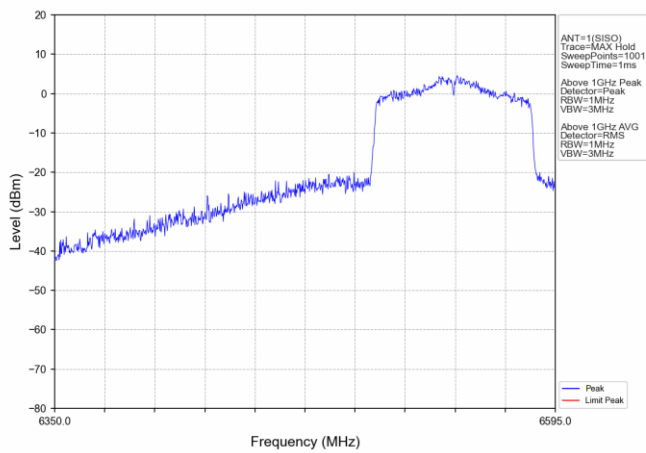
802.11ac(VHT80) HCH_6545MHz_Ant1_NTNV
