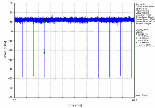
802.11n(HT40) HCH_6525MHz_Ant1_NTNV
