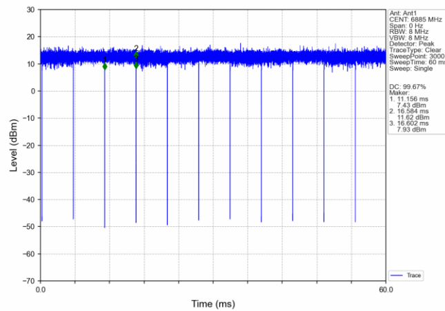
802.11n(HT40)_HCH_6885MHz_Ant1_NTNV
