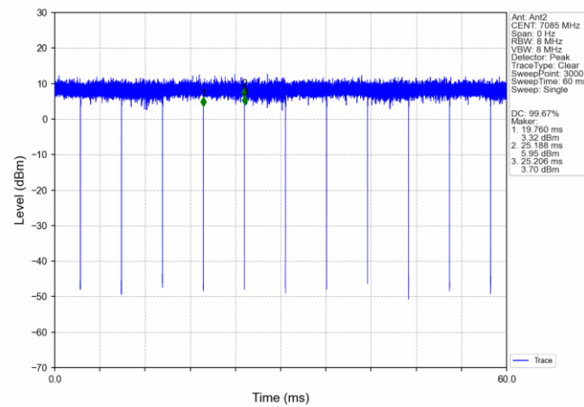
802.11ac(VHT40) HCH 7085MHz Ant2_NTNV
