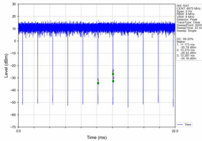
802.11n(HT20)_HCH_6875MHz_Ant1_NTNV
