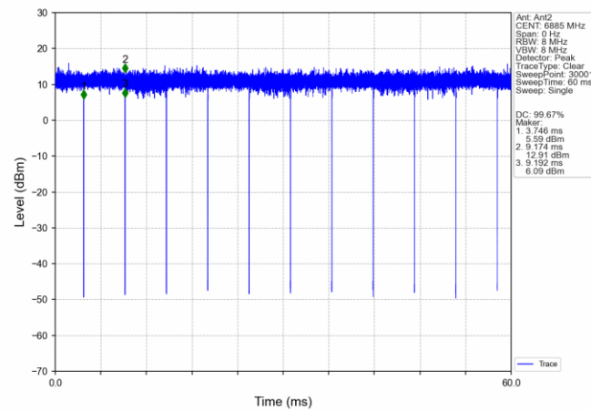
802.11n(HT40)_HCH_6885MHz_Ant2_NTNV
