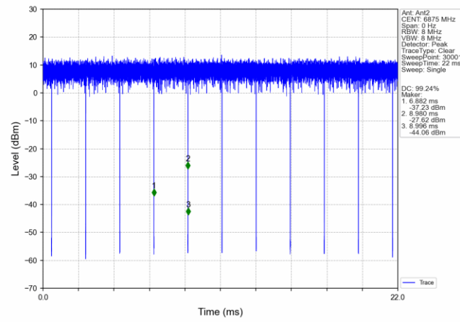
802.11n(HT20)_HCH_6875MHz_Ant2_NTNV
