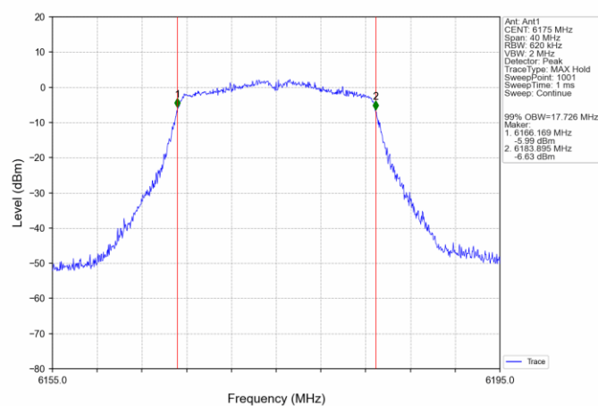
802.11ac(VHT20) MCH_6175MHz_Ant1_NTNV
