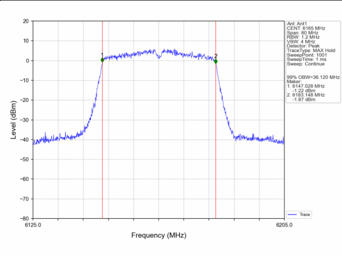
802.11ac(VHT40) MCH_6165MHz_Ant1_NTNV
