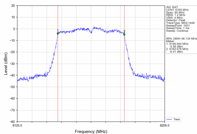
802.11n(HT40) MCH_6165MHz_Ant1_NTNV
