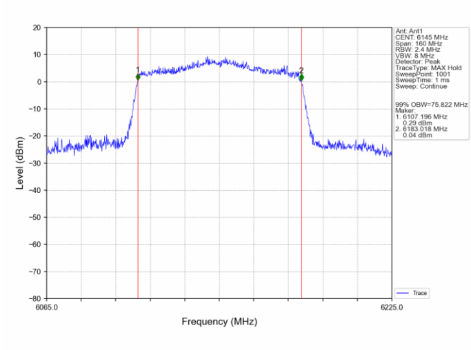
802.11ac(VHT80) MCH_6145MHz_Ant1_NTNV
