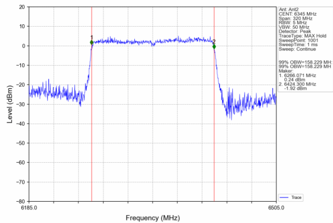
802.11ax(HEW160) HCH 6345MHz SU / Ant2 NTV
