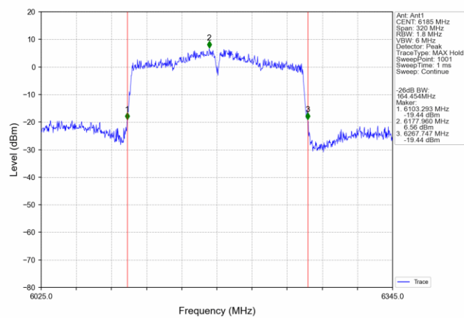
802.11ac(VHT160) MCH 6185MHz Ant1 NTN
