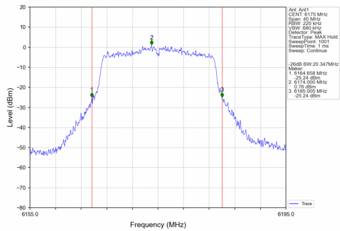
802.11ac(VHT20) MCH_6175MHz_Ant1_NTNV
