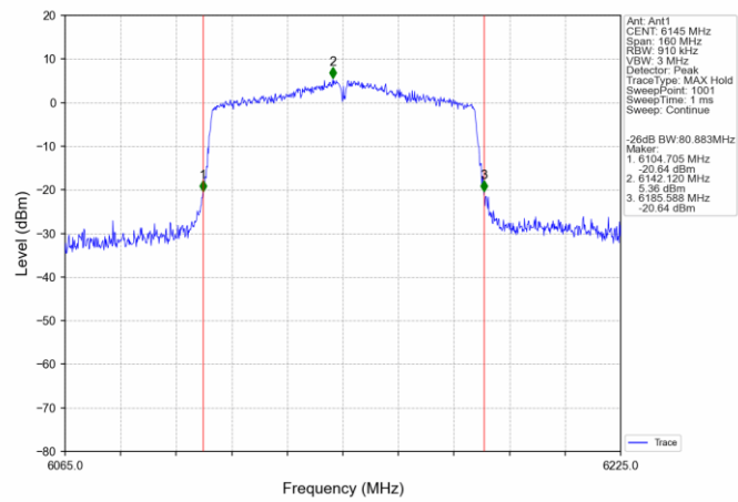
802.11ac(VHT80) MCH_6145MHz_Ant1_NTNV
