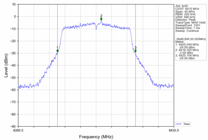
802.11n(HT20) HCH 6415MHz Ant2 NTN
