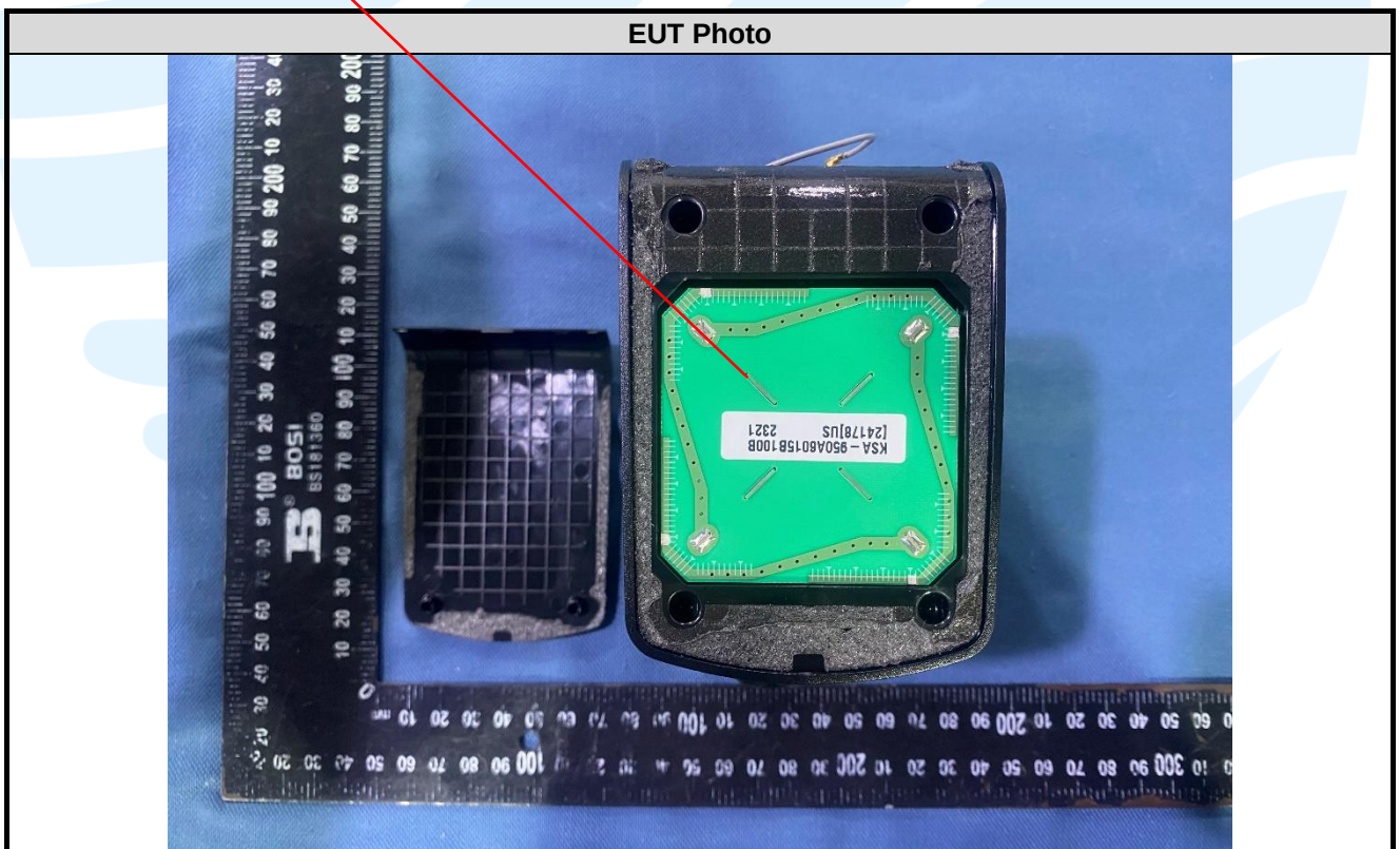
RFID Antenna
