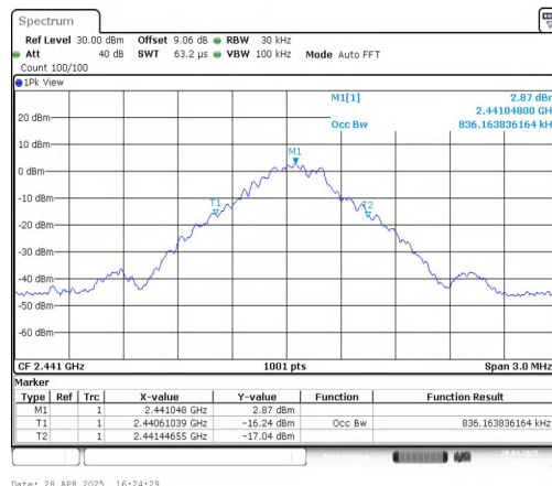
DH5-Ant1-2441
