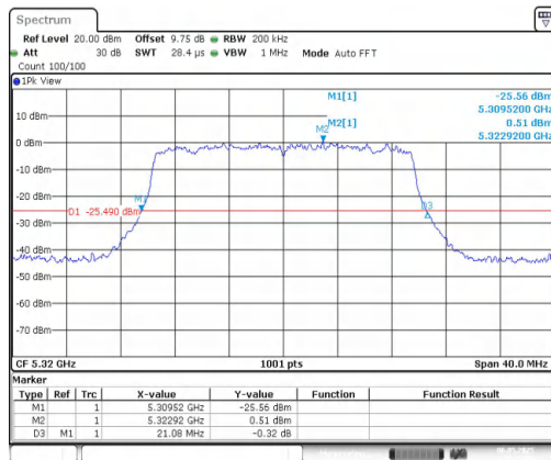
11AX20MIMO-Ant1-5320
