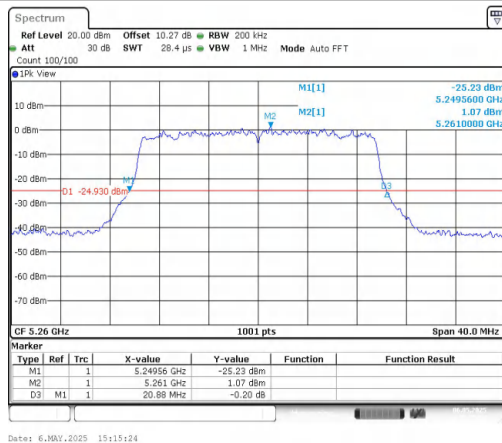
11AX20MIMO-Ant1-5260
