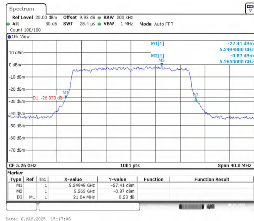
11AX20MIMO-Ant2-5260
