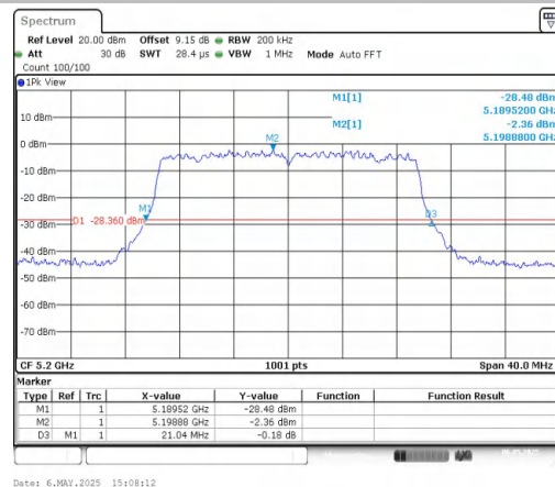
11AX20MIMO-Ant2-5200
