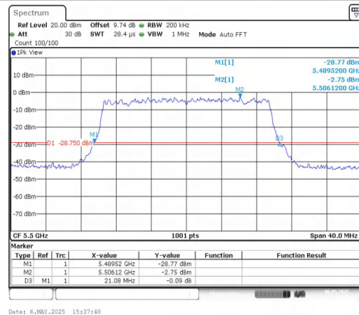
11AX20MIMO-Ant2-5500
