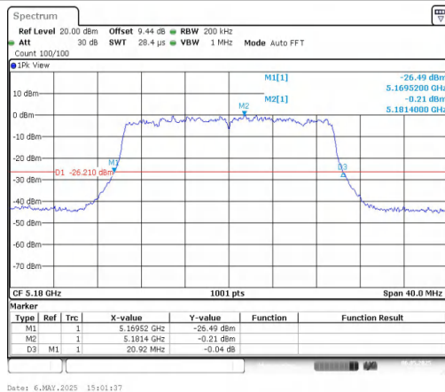
11AX20MIMO-Ant1-5180
