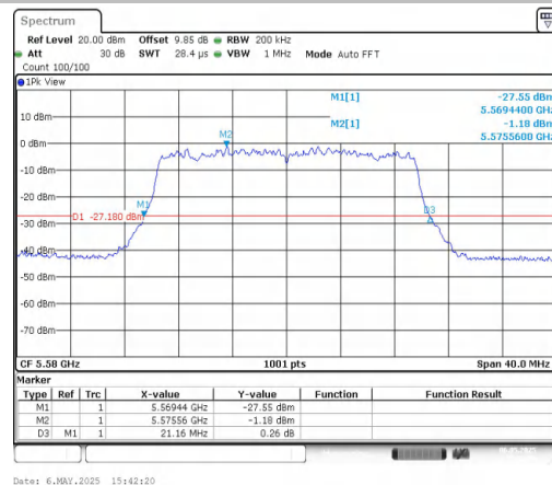
11AX20MIMO-Ant2-5580
