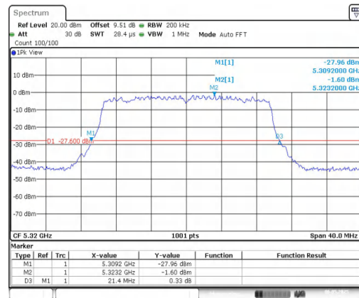
11AX20MIMO-Ant2-5320
