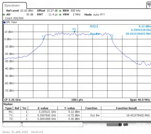
11AC20MIMO-Ant1-5260
