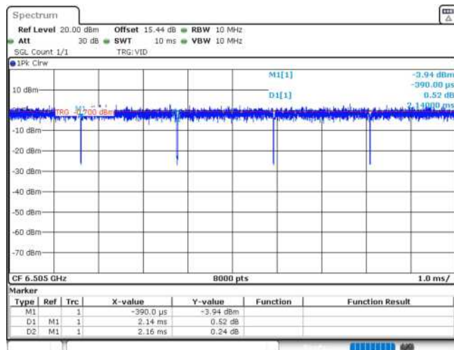
11AX160MIMO_Ant1_6505
