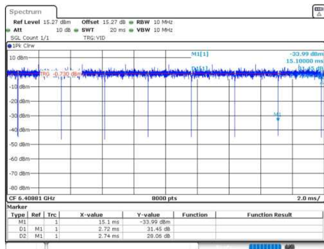
11AX20MIMO_Ant1_6415_106Tone_RU53
