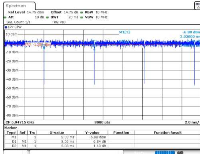
11AX20MIMO_Ant1_5955_52Tone_RU37
