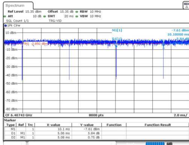
11AX20MIMO_Ant2_6415_52Tone_RU37
