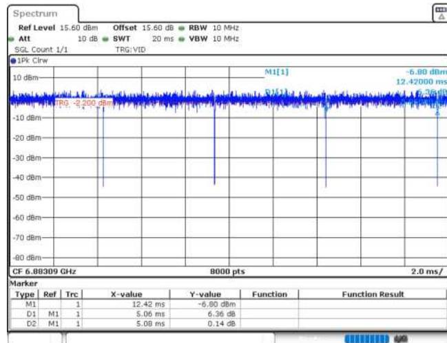
11AX20MIMO_Ant2_6875_52Tone_RU40
