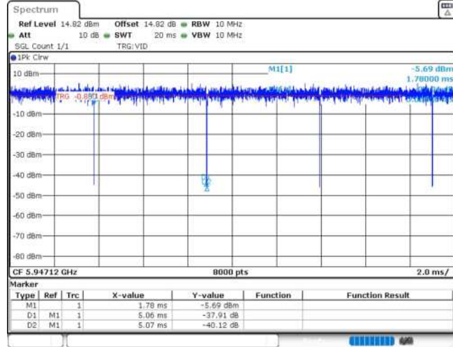
11AX20MIMO_Ant2_5955_52Tone_RU37
