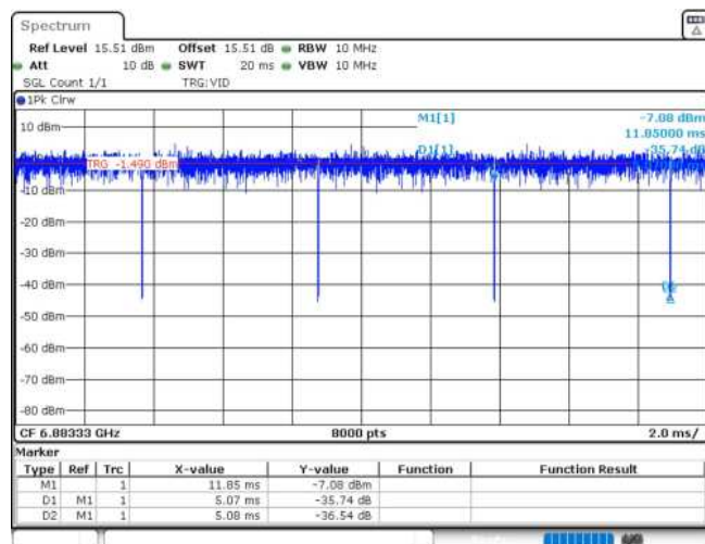
11AX20MIMO_Ant1_6875_26Tone_RU0
