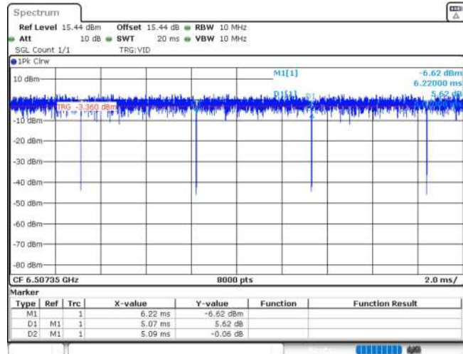
11AX20MIMO_Ant1_6515_26Tone_RU0
