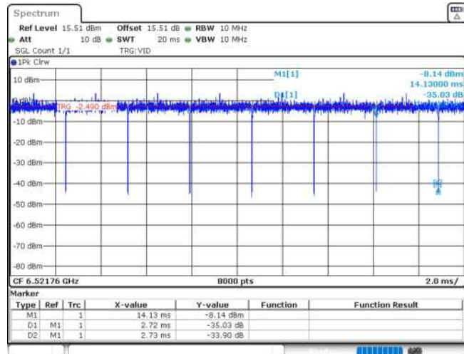
11AX20MIMO_Ant2_6515_106Tone_RU54
