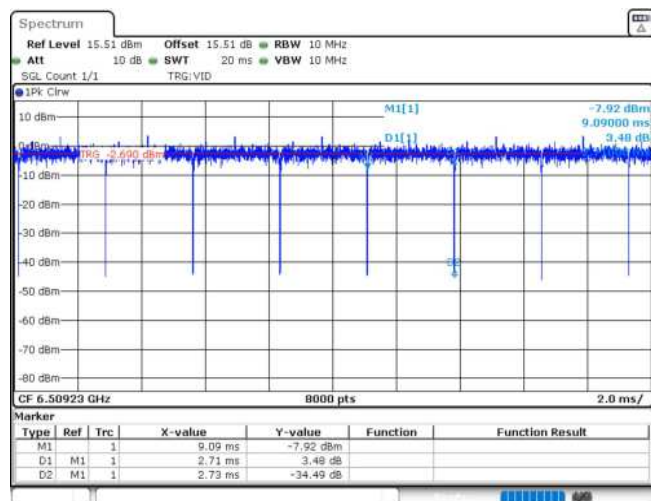
11AX20MIMO_Ant2_6515_106Tone_RU53
