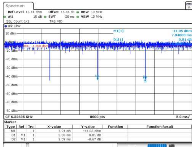
11AX20MIMO_Ant1_6535_26Tone_RU0
