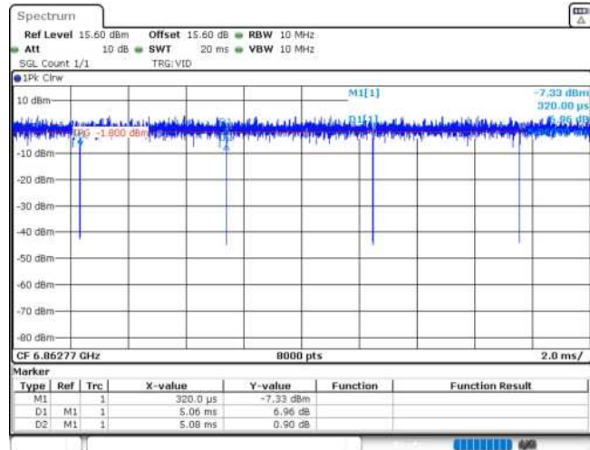
11AX20MIMO_Ant2_6855_52Tone_RU40
