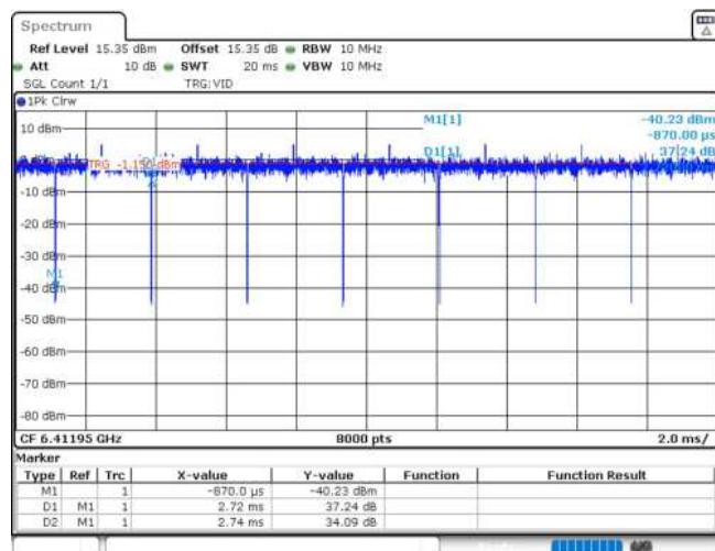
11AX20MIMO_Ant2_6415_106Tone_RU53
