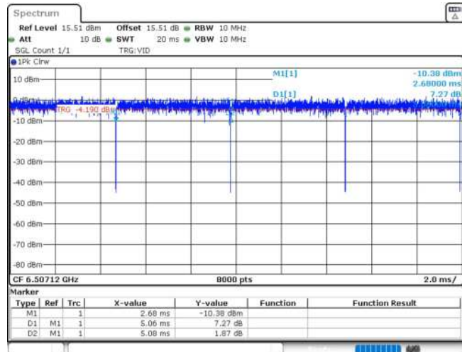
11AX20MIMO_Ant2_6515_52Tone_RU37
