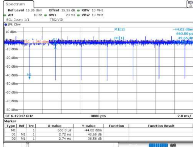
11AX20MIMO_Ant2_6415_106Tone_RU54
