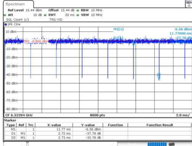
11AX20MIMO_Ant1_6515_106Tone_RU54
