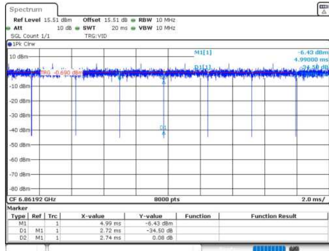
11AX20MIMO_Ant1_6855_106Tone_RU54
