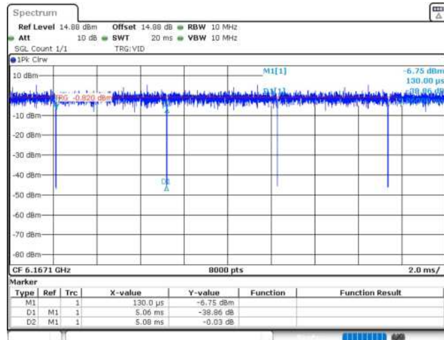
11AX20MIMO_Ant1_6175_52Tone_RU37
