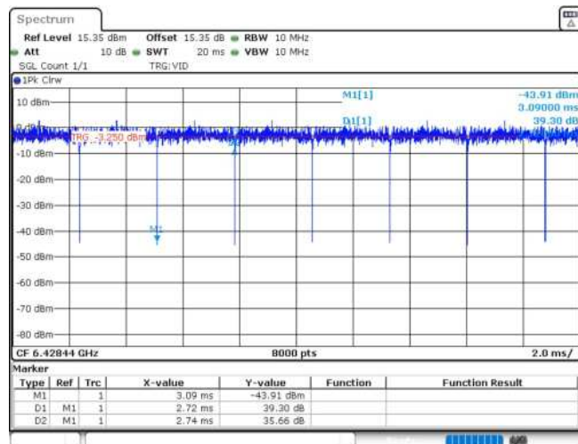
11AX20MIMO_Ant2_6435_106Tone_RU53
