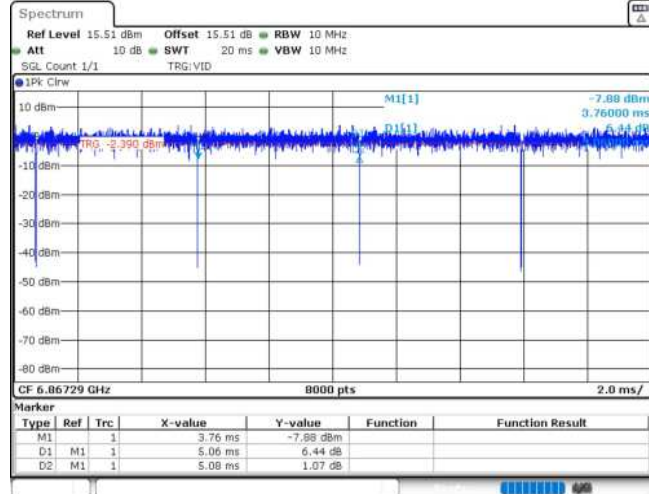
11AX20MIMO_Ant1_6875_52Tone_RU37
