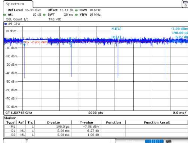
11AX20MIMO_Ant1_6535_52Tone_RU37
