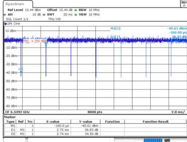
11AX20MIMO_Ant1_6535_106Tone_RU54
