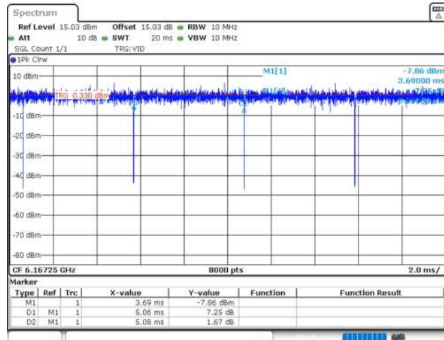
11AX20MIMO_Ant2_6175_52Tone_RU37
