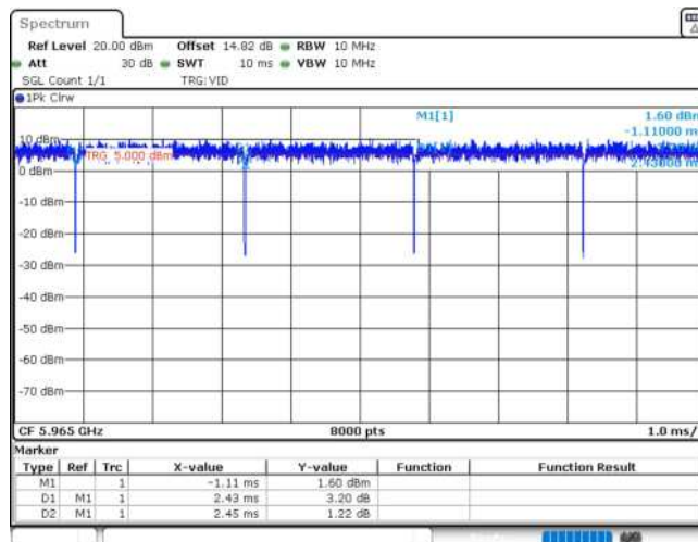
11AX40MIMO_Ant2_5965
