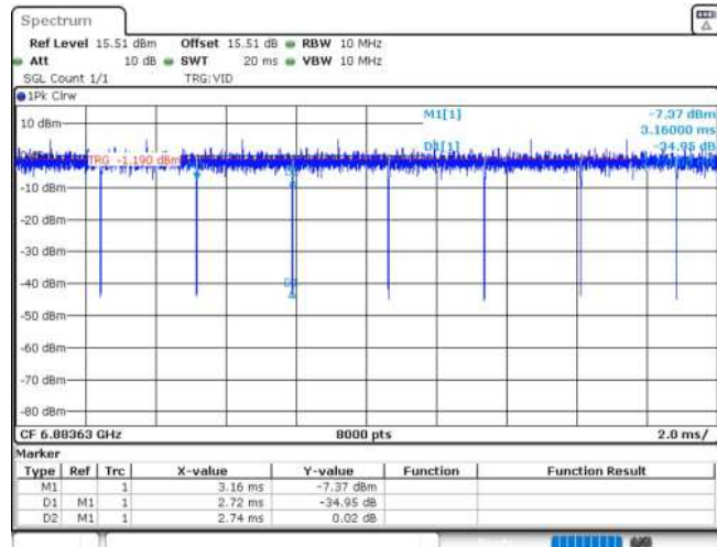
11AX20MIMO_Ant1_6875_106Tone_RU54
