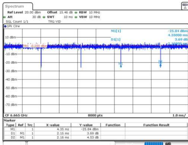
11AX160MIMO_Ant2_6665
