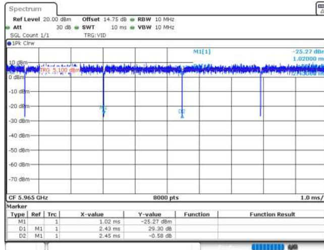
11AX40MIMO_Ant1_5965
