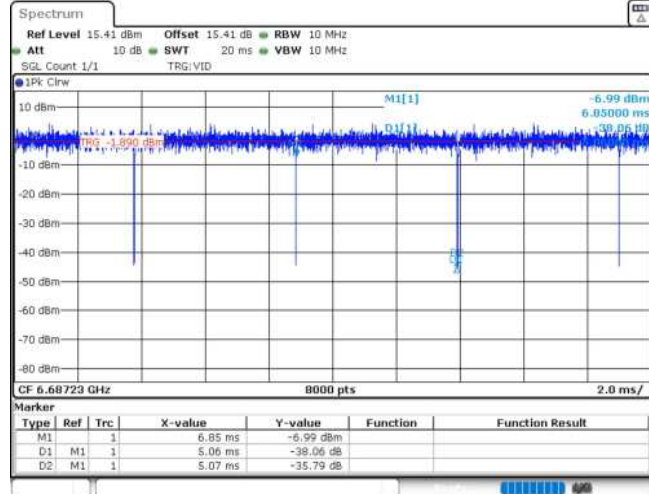
11AX20MIMO_Ant1_6695_52Tone_RU37
