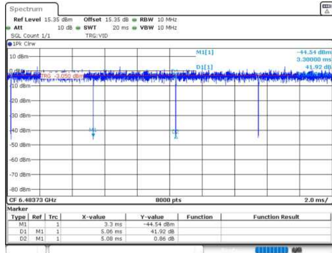
11AX20MIMO_Ant2_6475_52Tone_RU40
