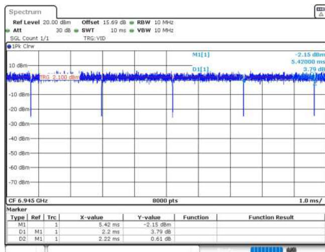
11AX80MIMO_Ant2_6945
