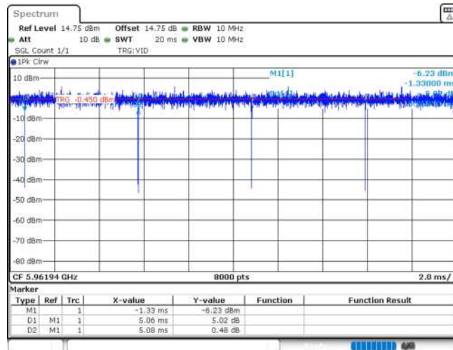
11AX20MIMO_Ant1_5955_52Tone_RU40
