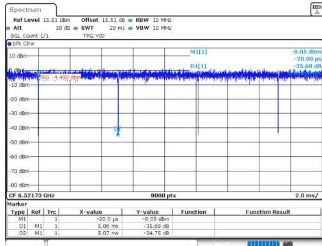
11AX20MIMO_Ant2_6515_52Tone_RU40
