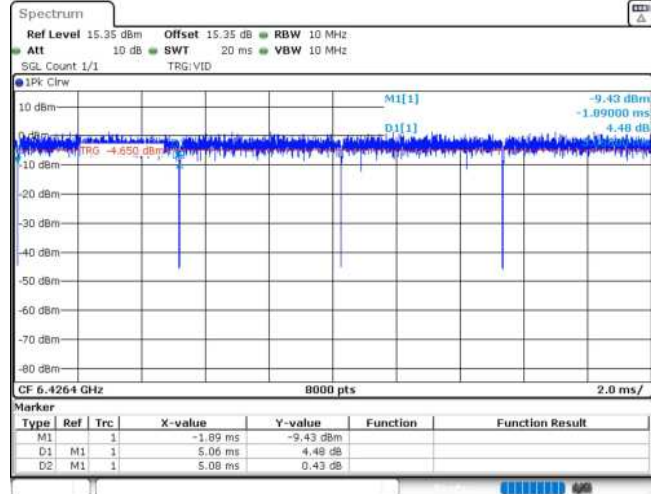
11AX20MIMO_Ant2_6435_52Tone_RU37
