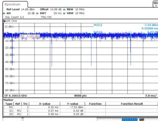
11AX20MIMO_Ant1_6175_26Tone_RU0
