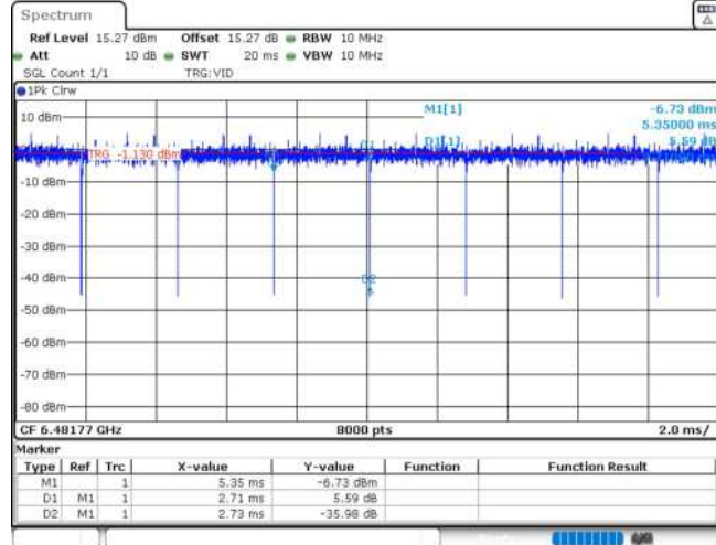
11AX20MIMO_Ant1_6475_106Tone_RU54
