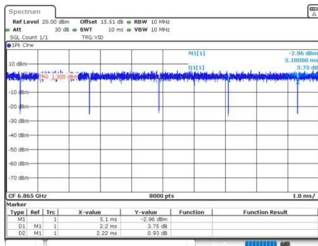
11AX80MIMO_Ant1_6865
