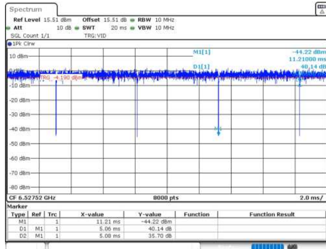
11AX20MIMO_Ant2_6535_52Tone_RU37
