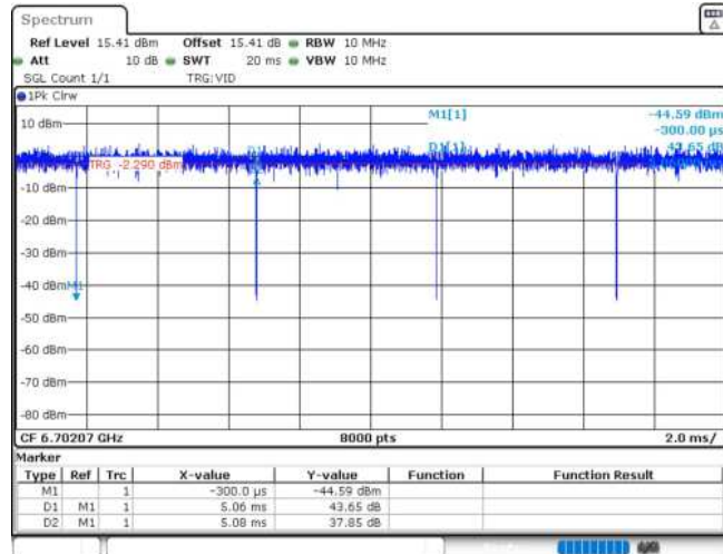
11AX20MIMO_Ant1_6695_52Tone_RU40
