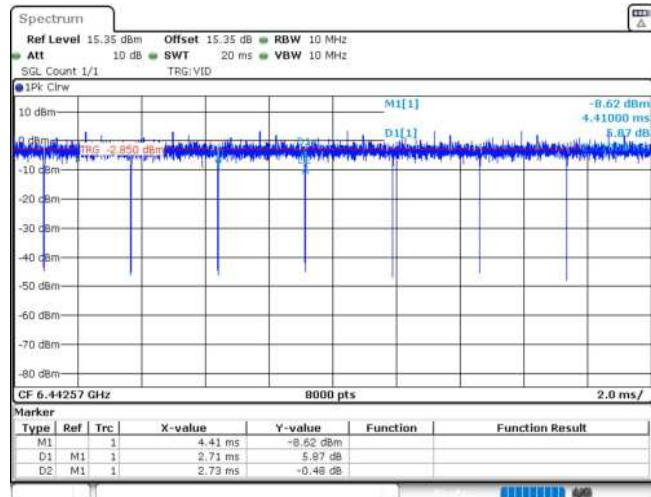
11AX20MIMO_Ant2_6435_106Tone_RU54
