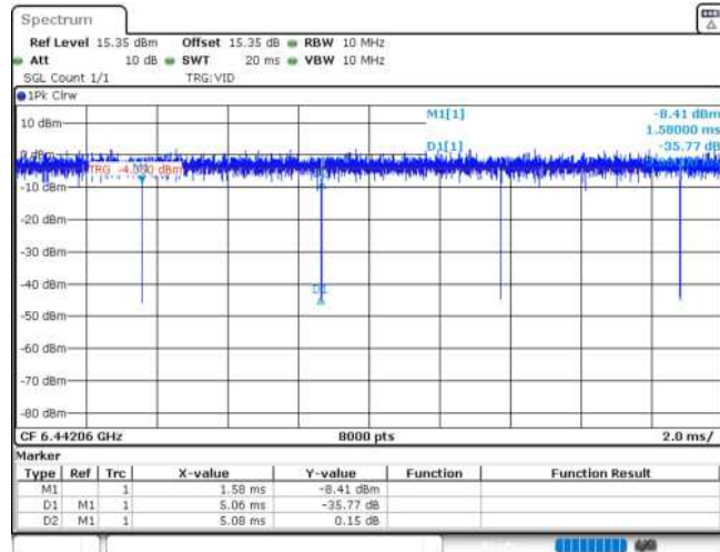
11AX20MIMO_Ant2_6435_52Tone_RU40
