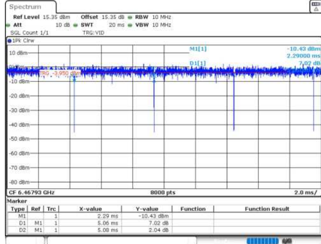
11AX20MIMO_Ant2_6475_52Tone_RU37
