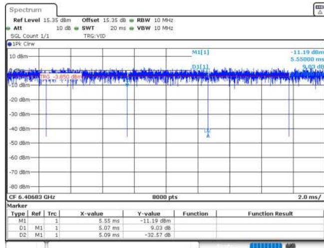
11AX20MIMO_Ant2_6415_26Tone_RU0
