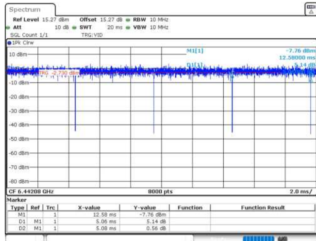
11AX20MIMO_Ant1_6435_52Tone_RU40
