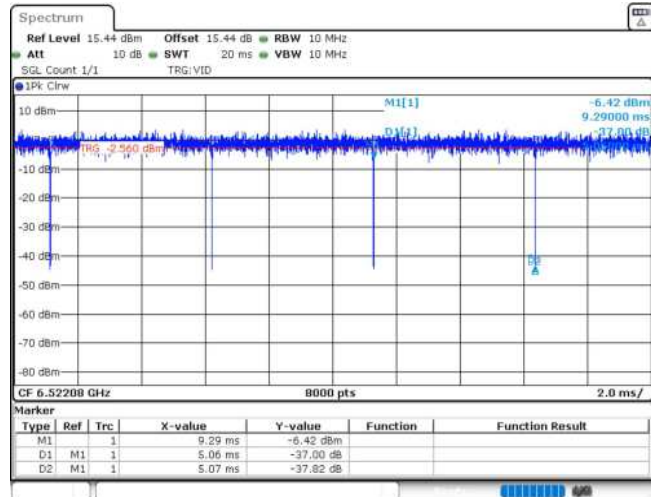
11AX20MIMO_Ant1_6515_52Tone_RU40
