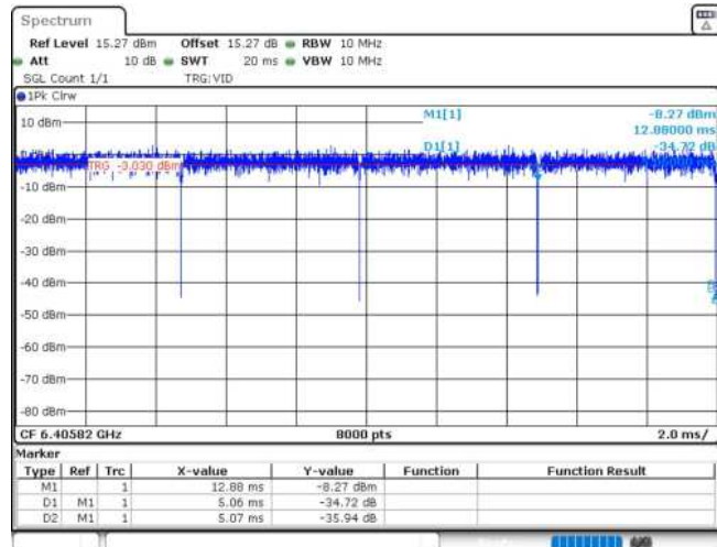
11AX20MIMO_Ant1_6415_52Tone_RU37
