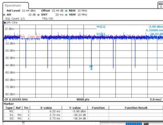
11AX20MIMO_Ant1_6535_106Tone_RU53
