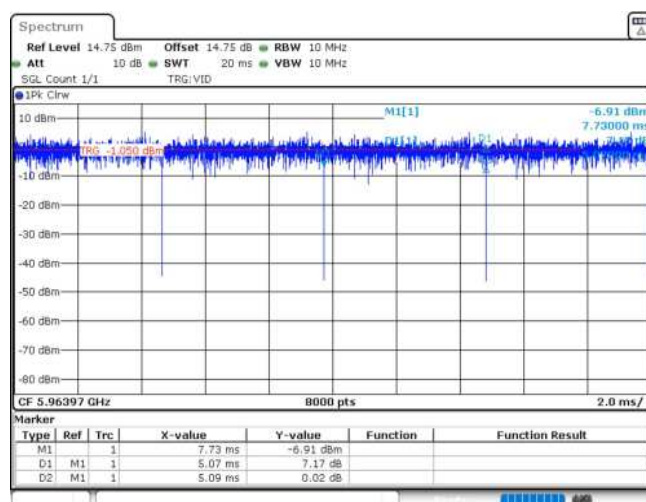
11AX20MIMO_Ant1_5955_26Tone_RU0
