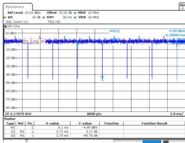
11AX20MIMO_Ant2_6175_106Tone_RU53
