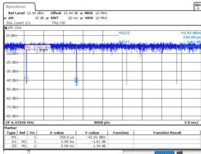
11AX20MIMO_Ant1_6515_26Tone_RU0
