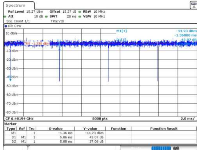
11AX20MIMO_Ant1_6475_52Tone_RU40
