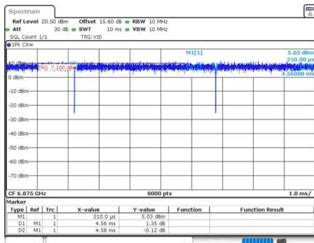
11AX20MIMO_Ant2_6875
