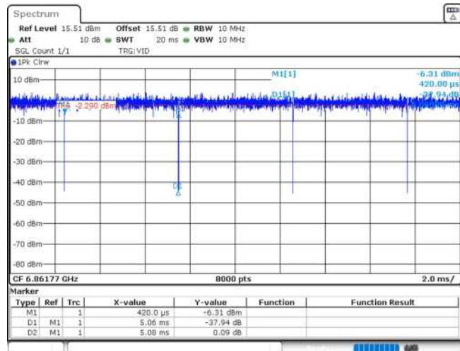
11AX20MIMO_Ant1_6855_52Tone_RU40
