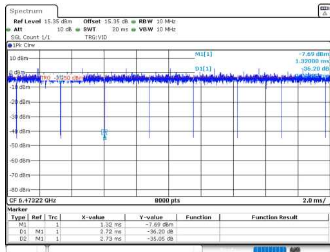
11AX20MIMO_Ant2_6475_106Tone_RU53
