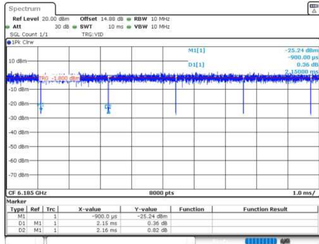
11AX160MIMO_Ant1_6185
