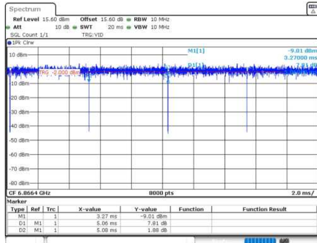
11AX20MIMO_Ant2_6875_52Tone_RU37
