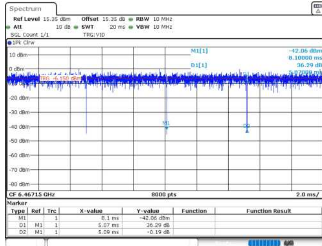
11AX20MIMO_Ant2_6475_26Tone_RU0
