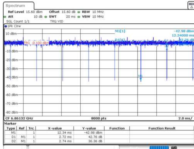
11AX20MIMO_Ant2_6855_106Tone_RU54
