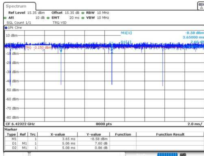
11AX20MIMO_Ant2_6415_52Tone_RU40
