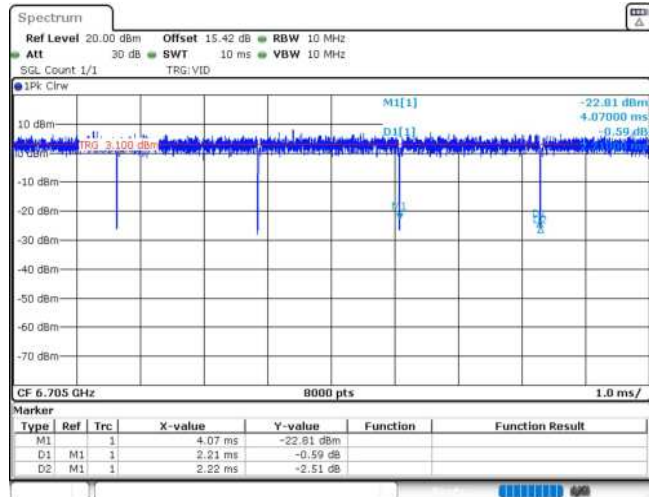
11AX80MIMO_Ant1_6705
