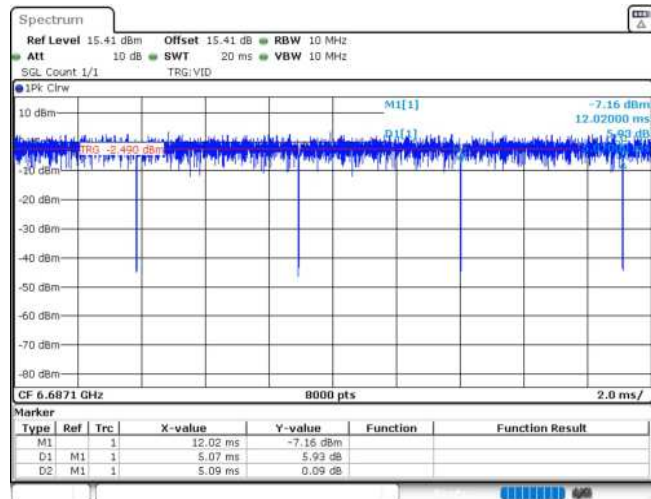
11AX20MIMO_Ant1_6695_26Tone_RU0
