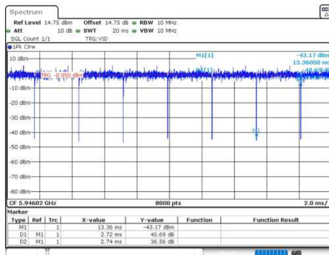
11AX20MIMO_Ant1_5955_106Tone_RU53
