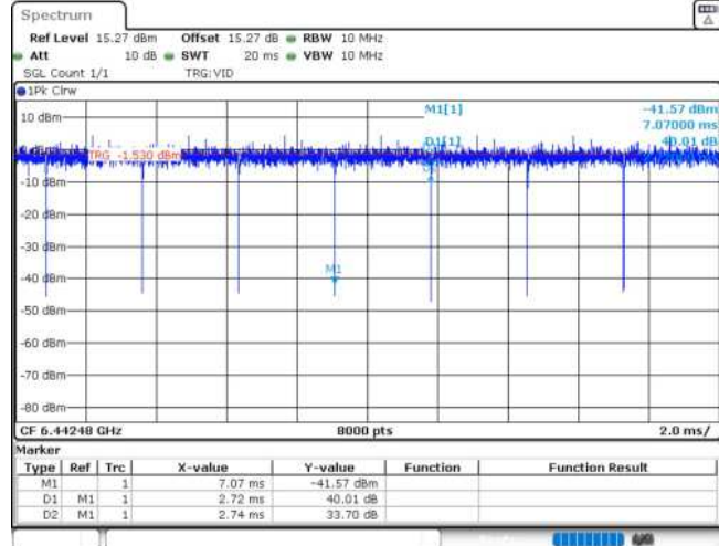
11AX20MIMO_Ant1_6435_106Tone_RU54
