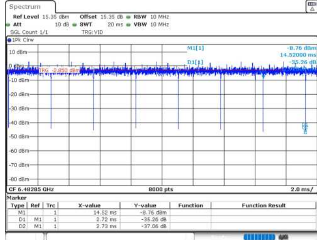
11AX20MIMO_Ant2_6475_106Tone_RU54
