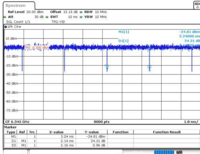
11AX160MIMO_Ant2_6345
