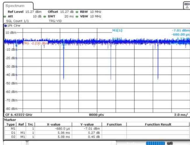
11AX20MIMO_Ant1_6415_52Tone_RU40
