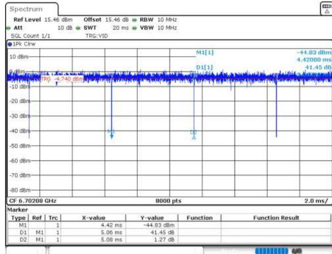
11AX20MIMO_Ant2_6695_52Tone_RU40
