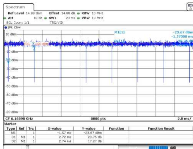
11AX20MIMO_Ant1_6175_106Tone_RU53
