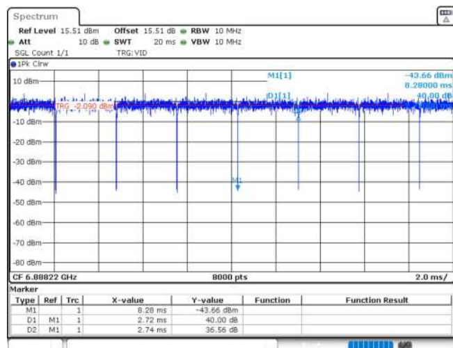
11AX20MIMO_Ant1_6895_106Tone_RU53
