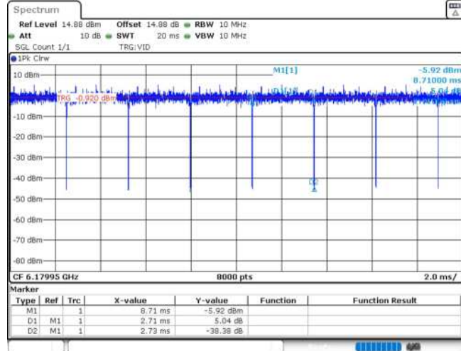
11AX20MIMO_Ant1_6175_106Tone_RU54
