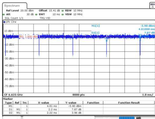
11AX80MIMO_Ant1_6625
