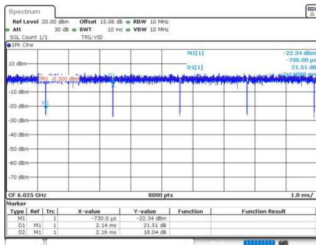
11AX160MIMO_Ant1_6025
