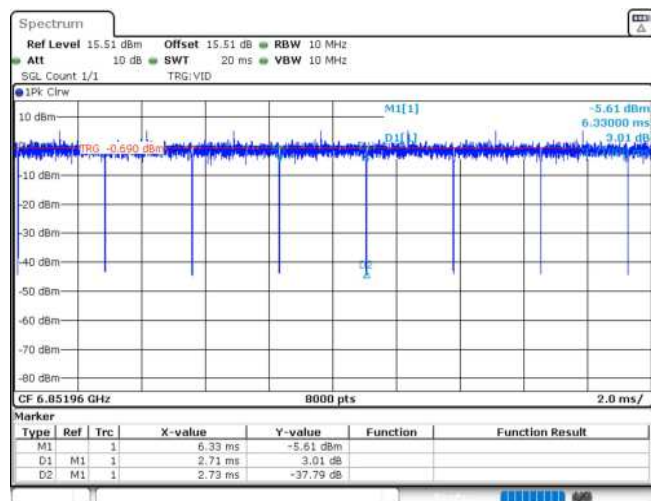
11AX20MIMO_Ant1_6855_106Tone_RU53
