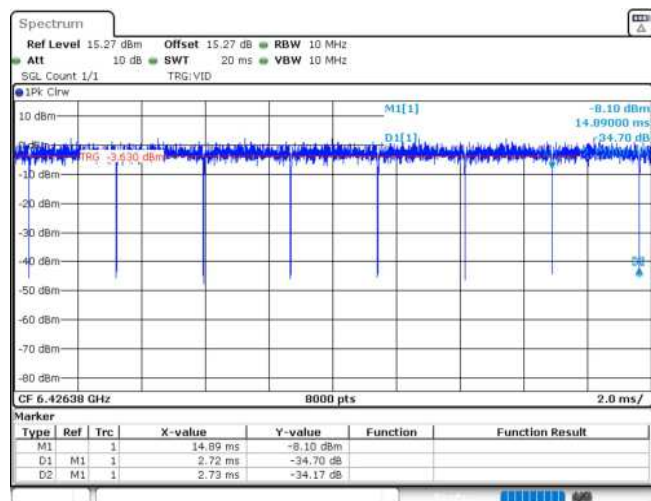
11AX20MIMO_Ant1_6435_106Tone_RU53
