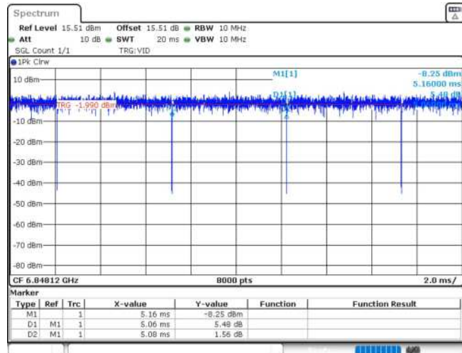
11AX20MIMO_Ant1_6855_52Tone_RU37
