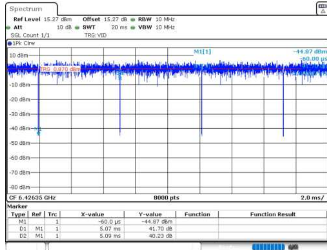
11AX20MIMO_Ant1_6435_26Tone_RU0
