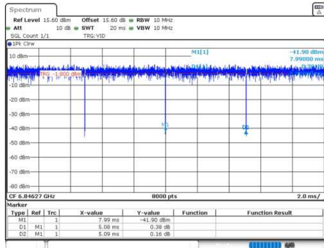
11AX20MIMO_Ant2_6855_26Tone_RU0
