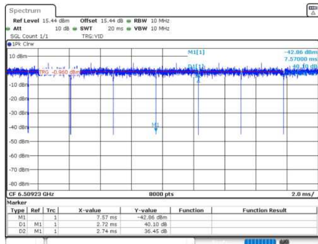
11AX20MIMO_Ant1_6515_106Tone_RU53
