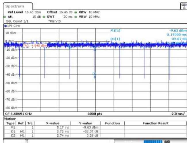
11AX20MIMO_Ant2_6695_106Tone_RU53
