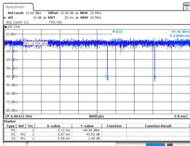
11AX20MIMO_Ant2_6855_26Tone_RU8
