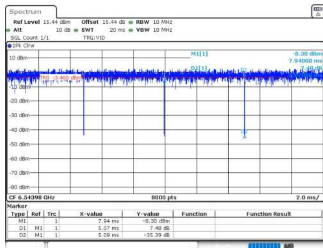
11AX20MIMO_Ant1_6535_26Tone_RU8
