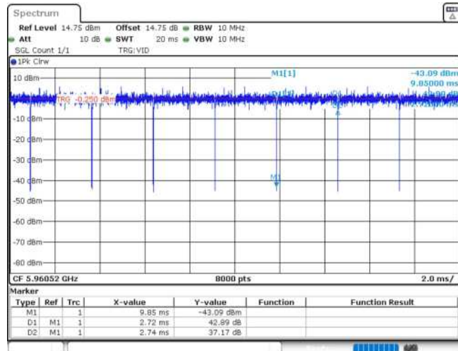
11AX20MIMO_Ant1_5955_106Tone_RU54
