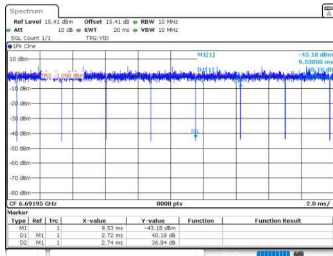
11AX20MIMO_Ant1_6695_106Tone_RU53
