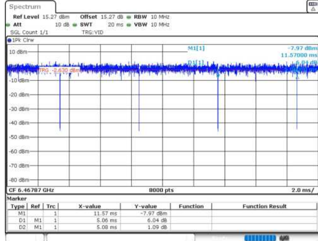
11AX20MIMO_Ant1_6475_52Tone_RU37
