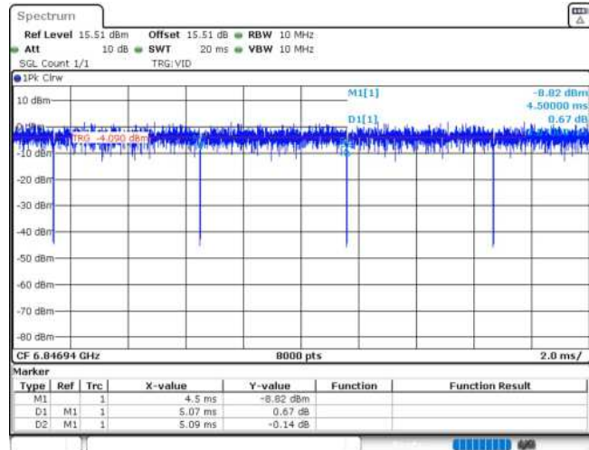
11AX20MIMO_Ant1_6855_26Tone_RU0
