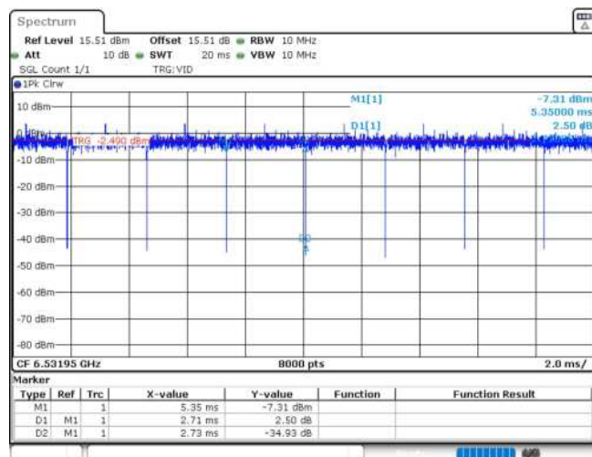
11AX20MIMO_Ant2_6535_106Tone_RU53
