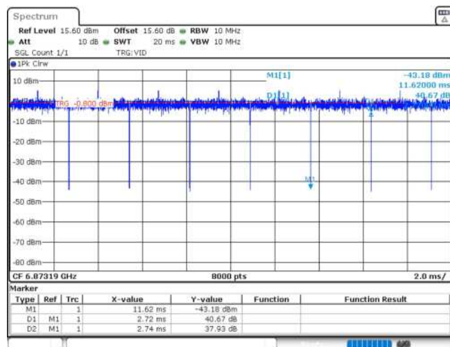
11AX20MIMO_Ant2_6875_106Tone_RU53
