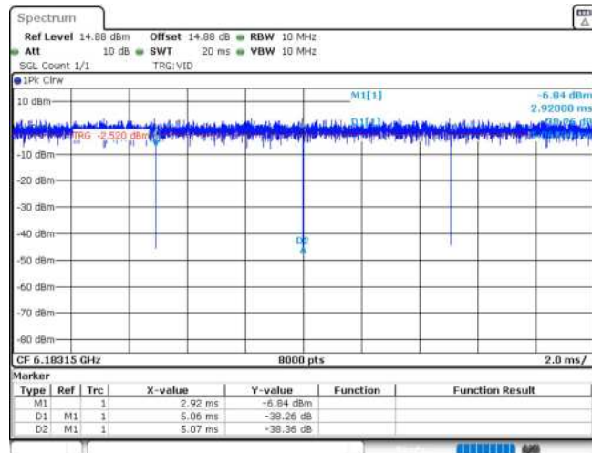
11AX20MIMO_Ant1_6175_52Tone_RU40
