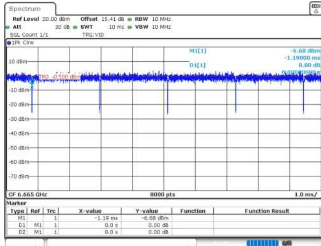
11AX160MIMO_Ant1_6665
