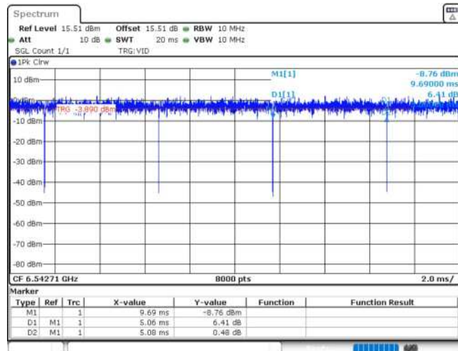
11AX20MIMO_Ant2_6535_52Tone_RU40
