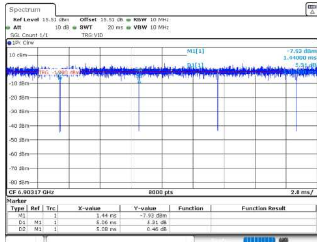
11AX20MIMO_Ant1_6895_52Tone_RU40
