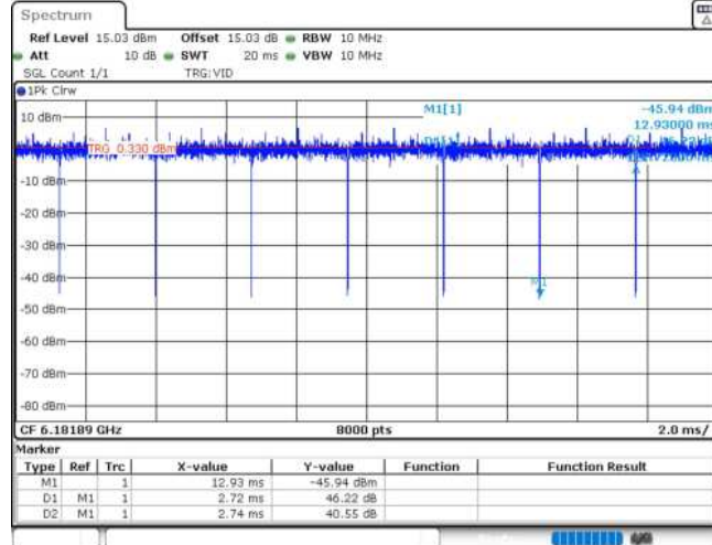
11AX20MIMO_Ant2_6175_106Tone_RU54
