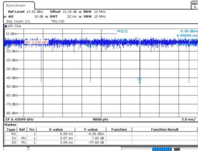
11AX20MIMO_Ant2_6435_26Tone_RU0
