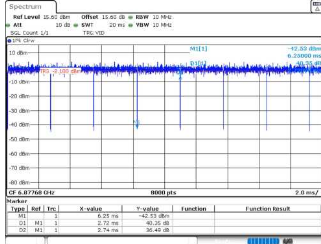
11AX20MIMO_Ant2_6875_106Tone_RU54
