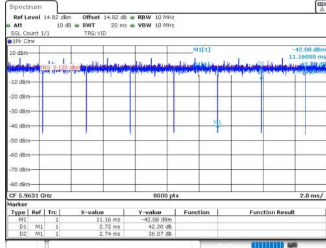
11AX20MIMO_Ant2_5955_106Tone_RU54
