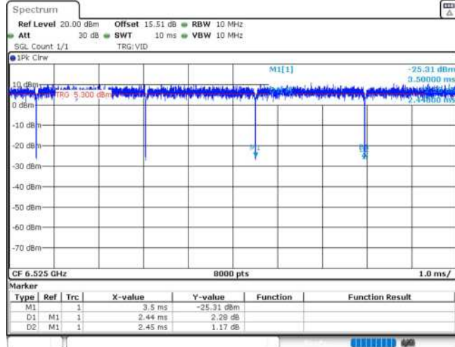
11AX40MIMO_Ant2_6525
