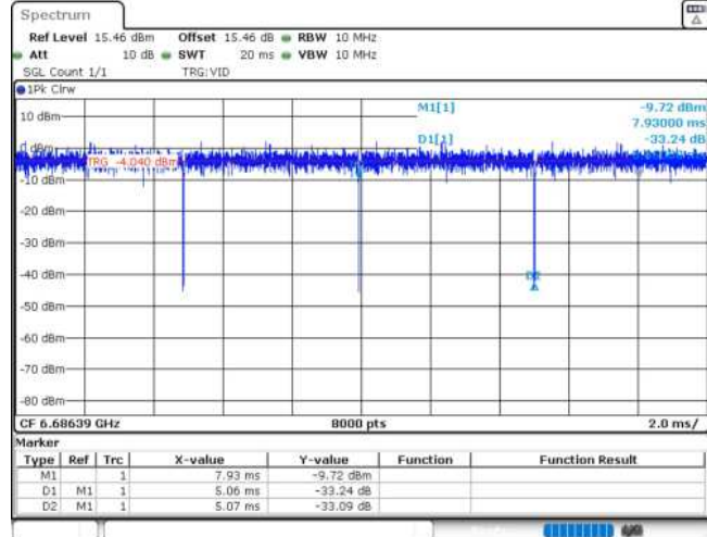
11AX20MIMO_Ant2_6695_52Tone_RU37
