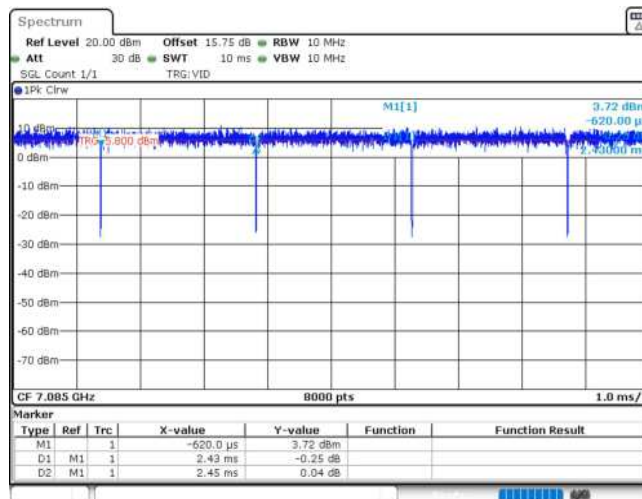
11AX40MIMO_Ant1_7085
