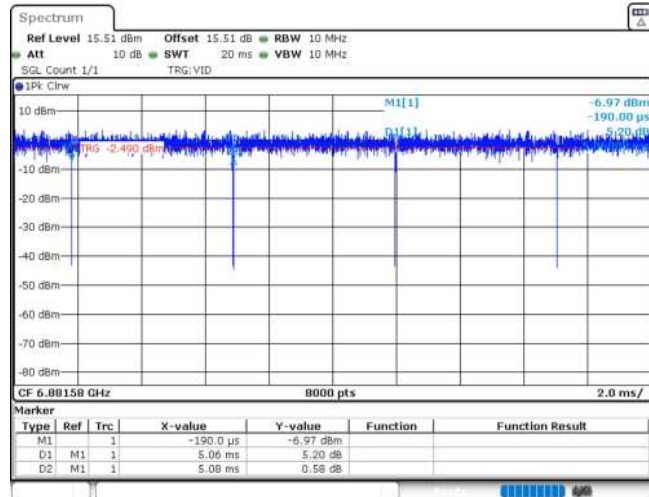
11AX20MIMO_Ant1_6875_52Tone_RU40
