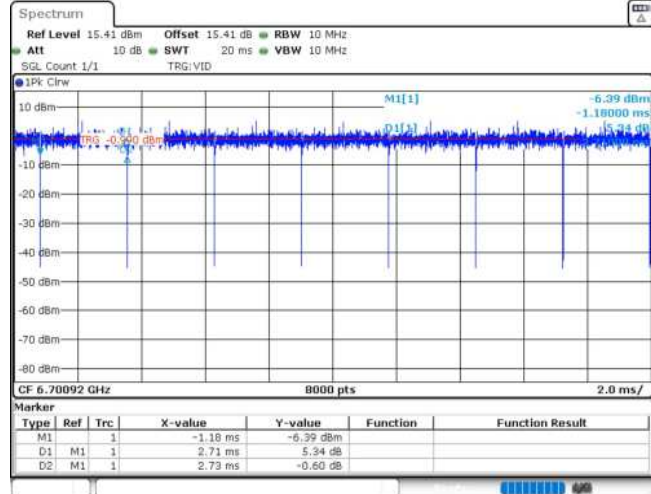
11AX20MIMO_Ant1_6695_106Tone_RU54
