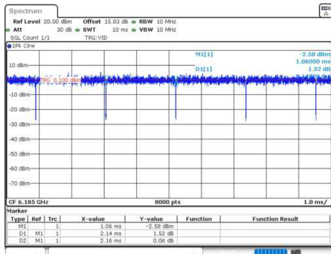
11AX160MIMO_Ant2_6185
