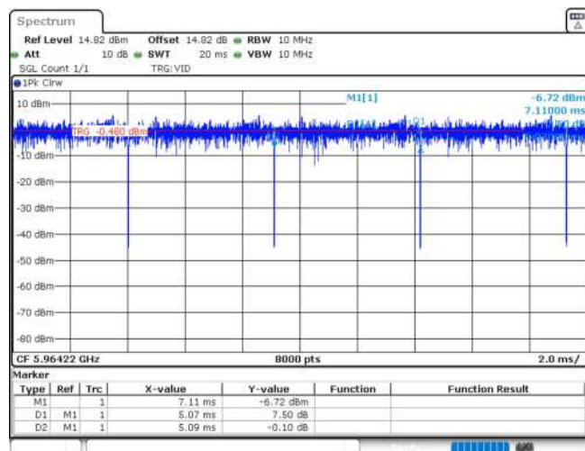
11AX20MIMO_Ant2_5955_26Tone_RU8
