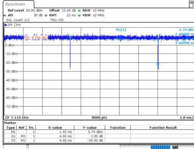
11AX20MIMO_Ant2_7115
