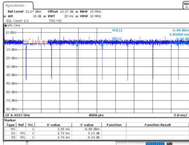
11AX20MIMO_Ant1_6415_106Tone_RU54
