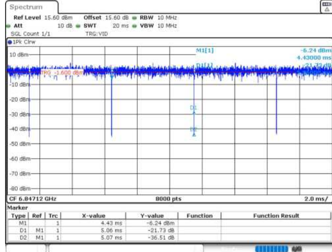
11AX20MIMO_Ant2_6855_52Tone_RU37
