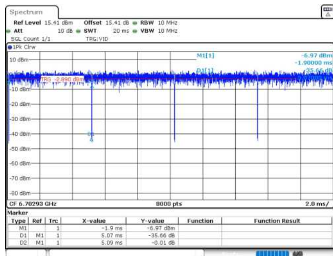
11AX20MIMO_Ant1_6695_26Tone_RU8
