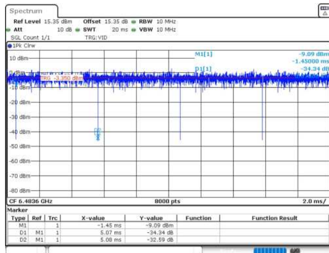
11AX20MIMO_Ant2_6475_26Tone_RU0
