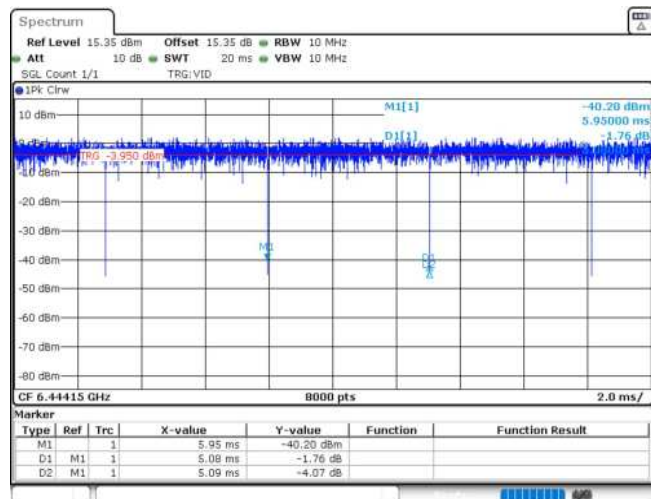
11AX20MIMO_Ant2_6435_26Tone_RU8
