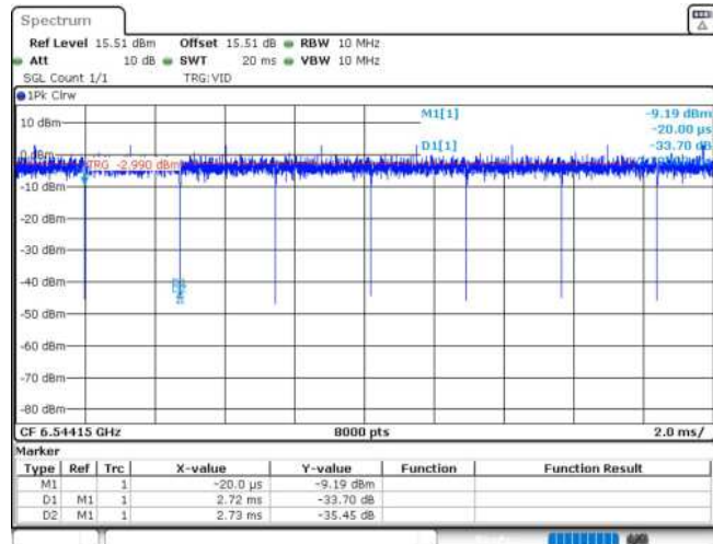
11AX20MIMO_Ant2_6535_106Tone_RU54
