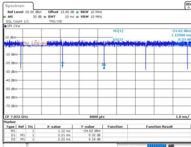
11AX80MIMO_Ant2_7025
