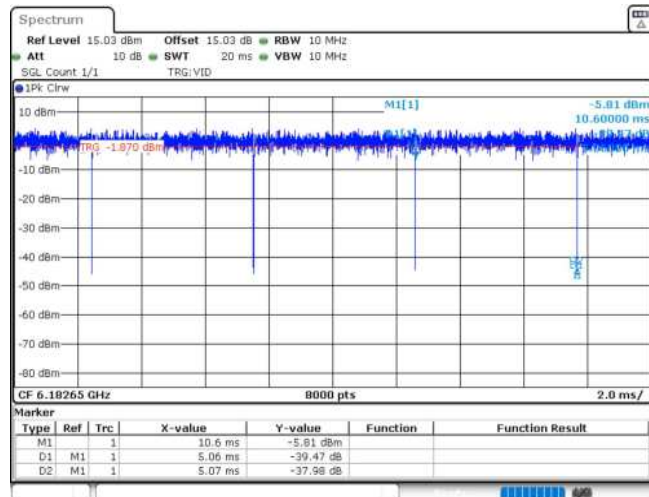
11AX20MIMO_Ant2_6175_52Tone_RU40
