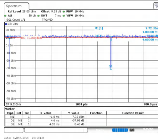
NTNV-11AX20MIMO-Ant2-5200
