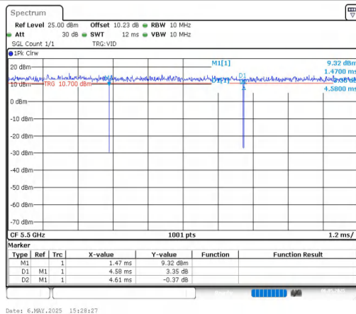
NTNV-11AX20MIMO-Ant1-5500
