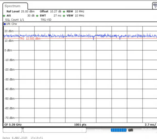
NTNV-11AX20MIMO-Ant1-5280
