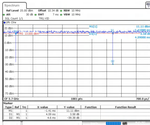
NTNV-11AX20MIMO-Ant1-5700
