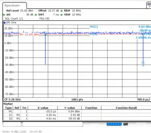
NTNV-11AX20MIMO-Ant1-5260
