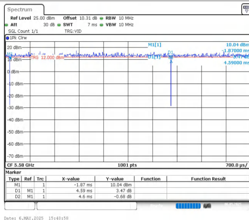
NTNV-11AX20MIMO-Ant1-5580
