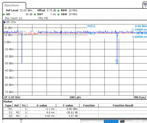
NTNV-11AX20MIMO-Ant1-5320
