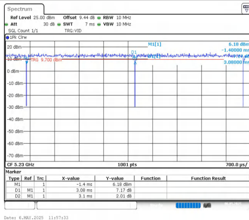
NTNV-11AC40MIMO-Ant1-5230
