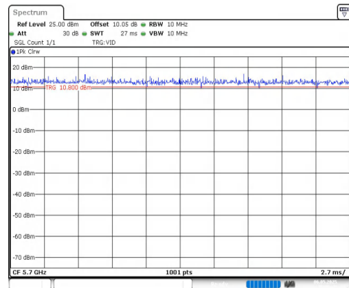
NTNV-11AX20MIMO-Ant2-5700
