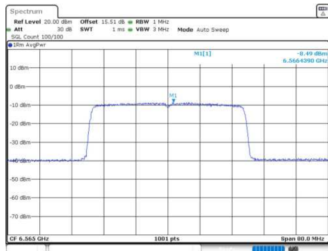
11AX40MIMO_Ant1_6565
