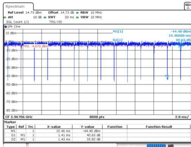
11AX80MIMO_Ant1_5985_484Tone_RU65
