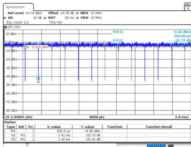
11AX80MIMO_Ant2_5985_484Tone_RU66
