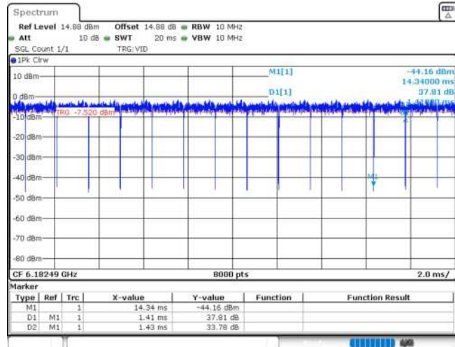
11AX80MIMO_Ant1_6145_484Tone_RU66
