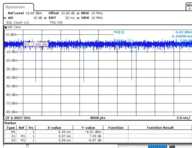
11AX20MIMO_Ant2_6895_26Tone_RU8
