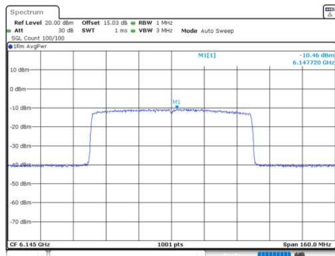
11AX80MIMO_Ant1_6145
