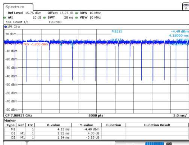
11AX40MIMO_Ant1_7085_242Tone_RU62
