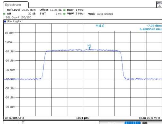
11AX40MIMO_Ant2_6485
