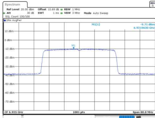
11AX40MIMO_Ant2_6925
