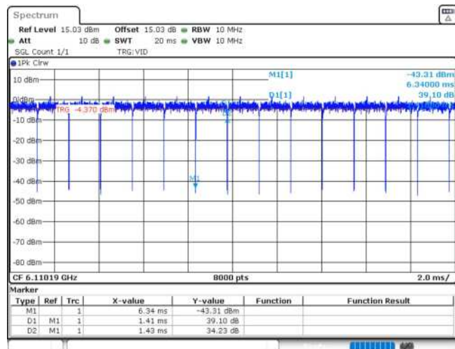
11AX80MIMO_Ant2_6145_484Tone_RU65
