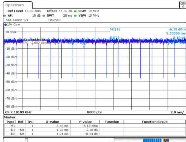
11AX40MIMO_Ant2_7085_242Tone_RU62
