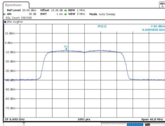
11AX20MIMO_Ant2_6695
