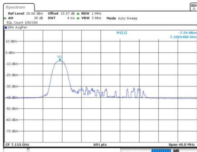
11AX20MIMO_Ant1_7115_26Tone_RU0
