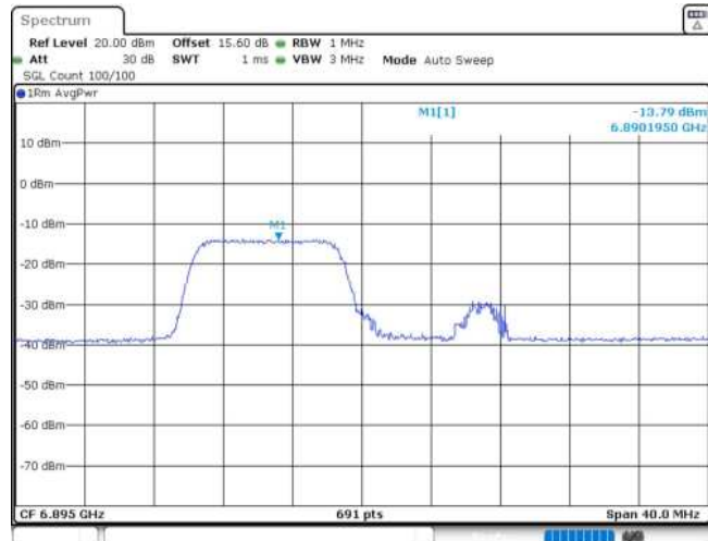
11AX20MIMO_Ant2_6895_106Tone_RU53
