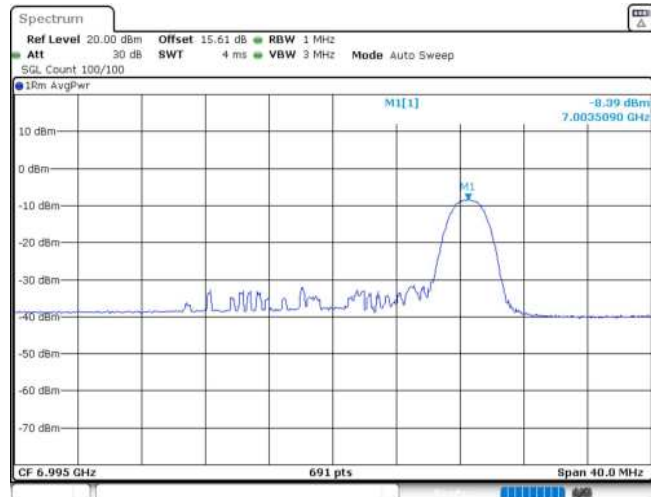
11AX20MIMO_Ant1_6995_26Tone_RU8
