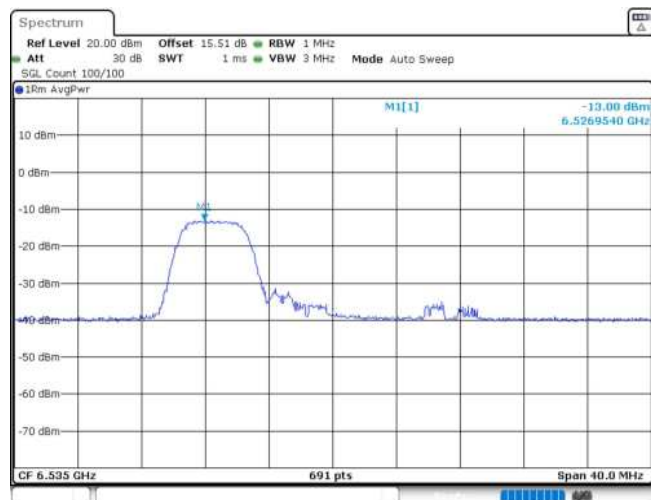
11AX20MIMO_Ant2_6535_26Tone_RU8
