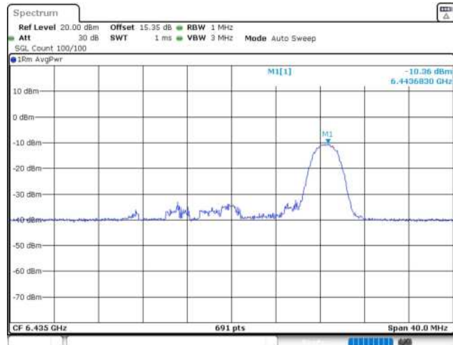
11AX20MIMO_Ant2_6435_26Tone_RU8
