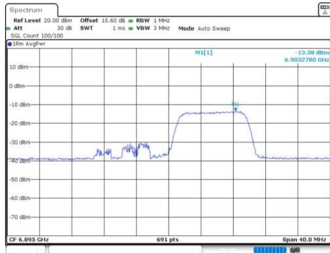
11AX20MIMO_Ant2_6895_106Tone_RU54
