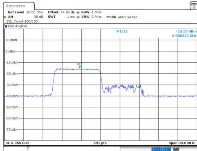
11AX40MIMO_Ant2_5965_242Tone_RU61
