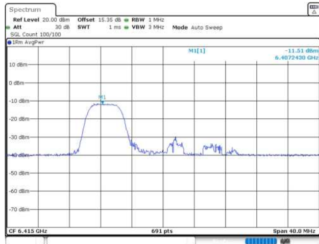
11AX20MIMO_Ant2_6415_52Tone_RU37
