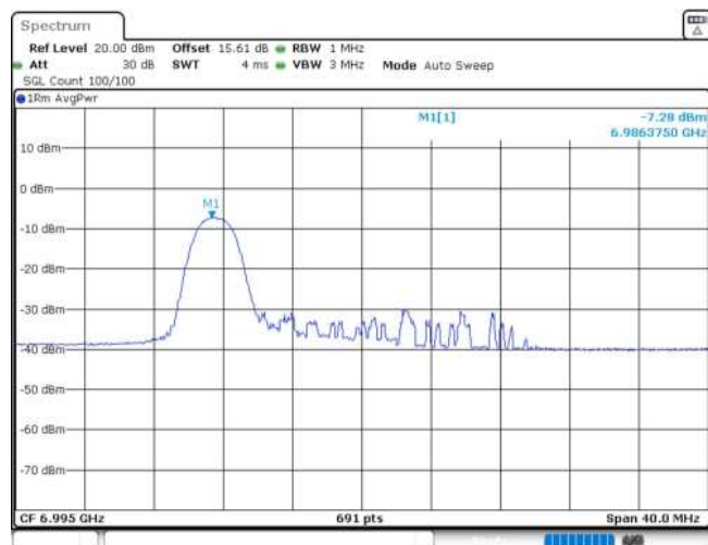
11AX20MIMO_Ant1_6995_26Tone_RU0
