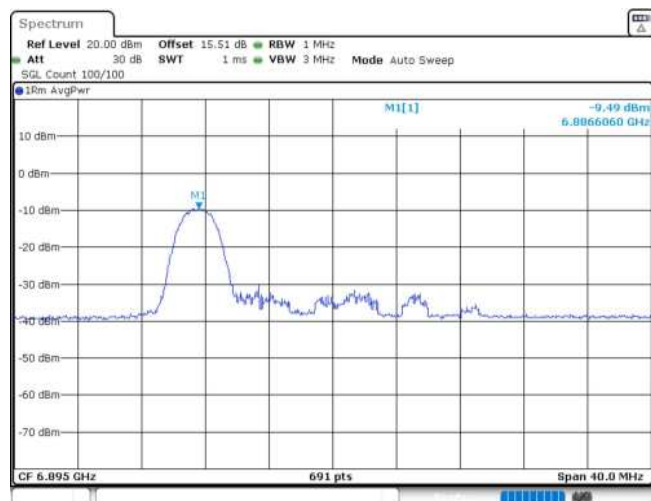
11AX20MIMO_Ant1_6895_26Tone_RU0
