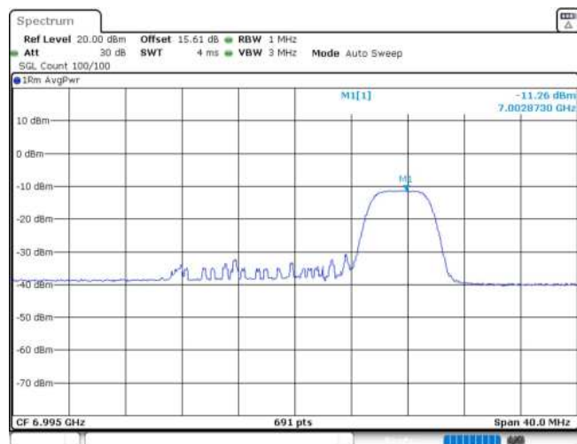
11AX20MIMO_Ant1_6995_52Tone_RU40
