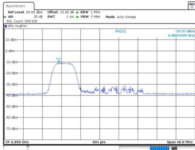
11AX20MIMO_Ant2_6895_52Tone_RU37
