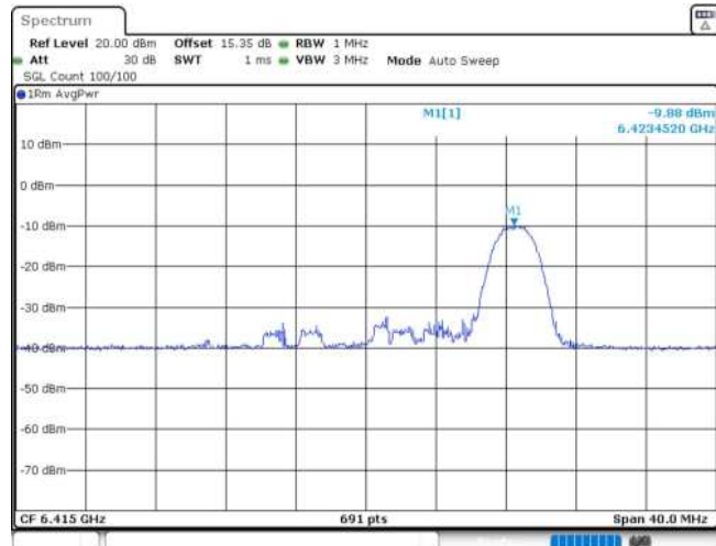
11AX20MIMO_Ant2_6415_26Tone_RU8
