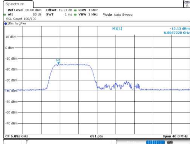
11AX20MIMO_Ant1_6895_106Tone_RU53
