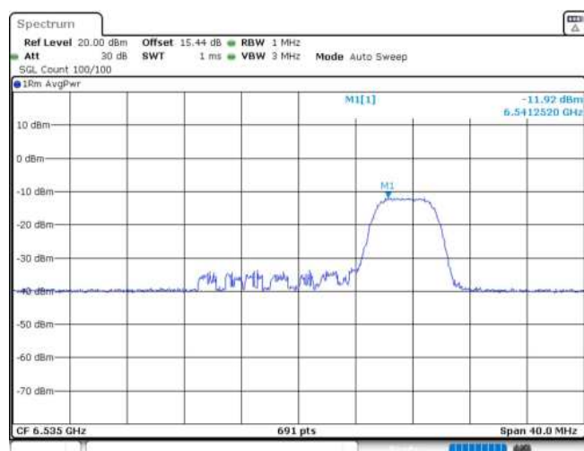
11AX20MIMO_Ant1_6535_52Tone_RU37
