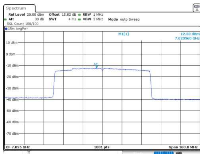
11AX80MIMO_Ant1_7025
