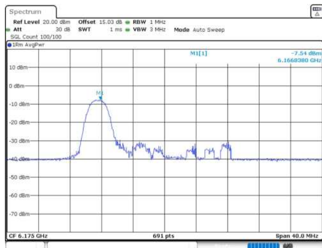
11AX20MIMO_Ant2_6175_26Tone_RU0
