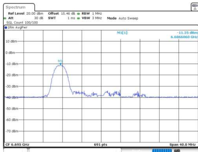
11AX20MIMO_Ant2_6695_26Tone_RU0
