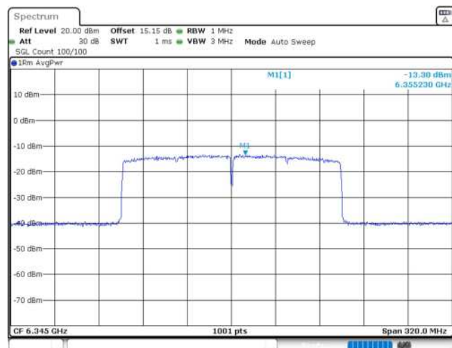
11AX160MIMO_Ant2_6345
