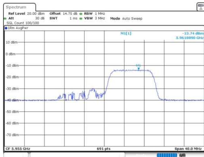
11AX20MIMO_Ant1_5955_106Tone_RU54
