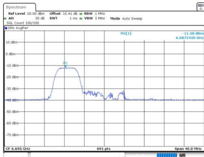
11AX20MIMO_Ant1_6695_52Tone_RU37
