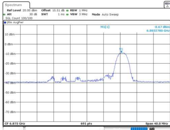
11AX20MIMO_Ant1_6875_26Tone_RU8
