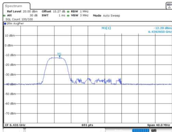
11AX20MIMO_Ant1_6435_52Tone_RU37
