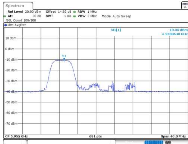
11AX20MIMO_Ant2_5955_52Tone_RU37
