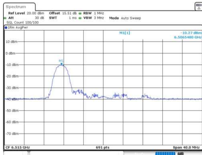
11AX20MIMO_Ant2_6515_26Tone_RU0
