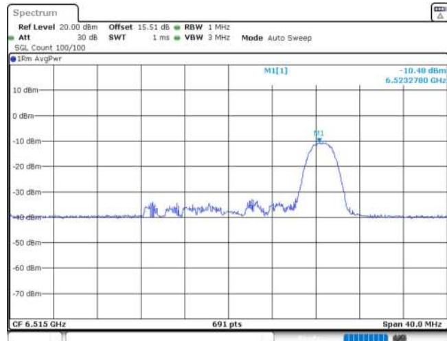
11AX20MIMO_Ant2_6515_26Tone_RU8
