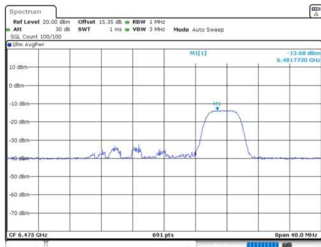
11AX20MIMO_Ant2_6475_52Tone_RU40
