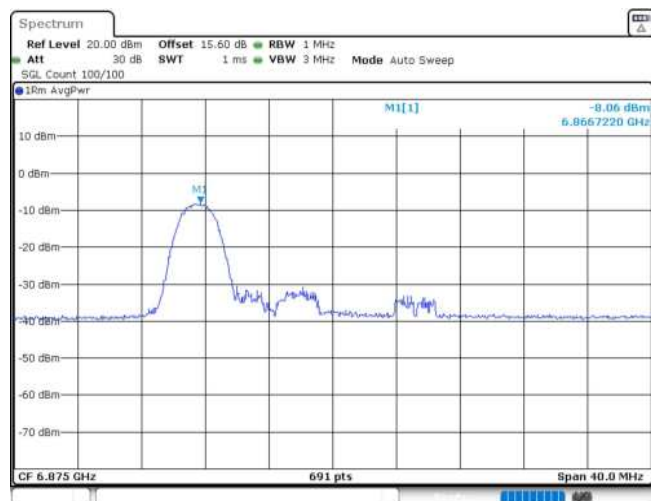
11AX20MIMO_Ant2_6875_26Tone_RU0
