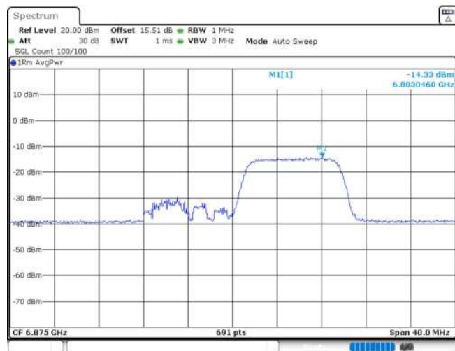
11AX20MIMO_Ant1_6875_106Tone_RU54
