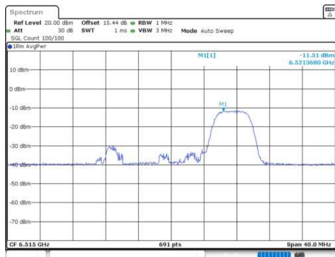
11AX20MIMO_Ant1_6515_52Tone_RU37
