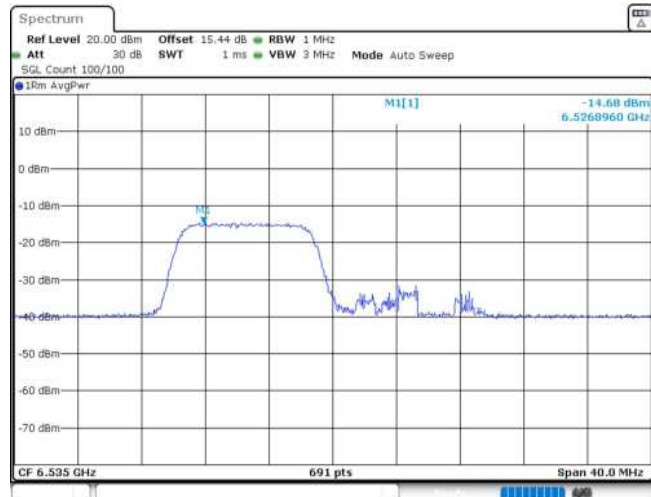
11AX20MIMO_Ant1_6535_106Tone_RU53
