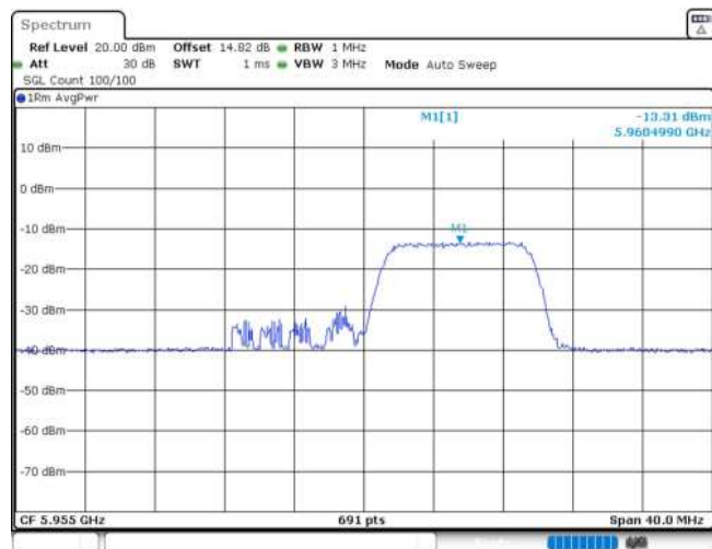
11AX20MIMO_Ant2_5955_106Tone_RU54
