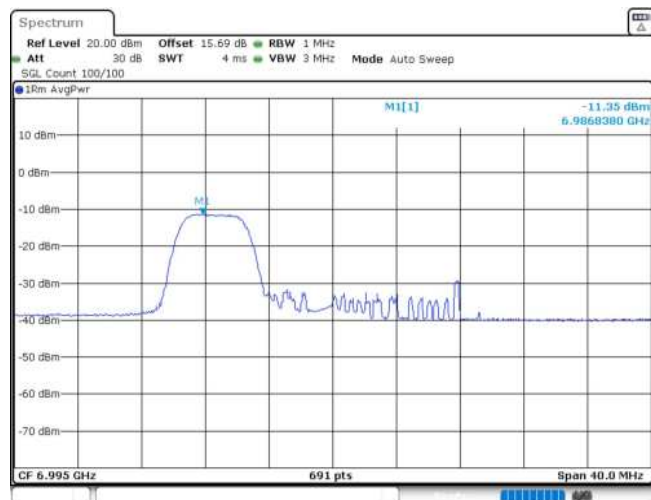
11AX20MIMO_Ant2_6995_26Tone_RU8
