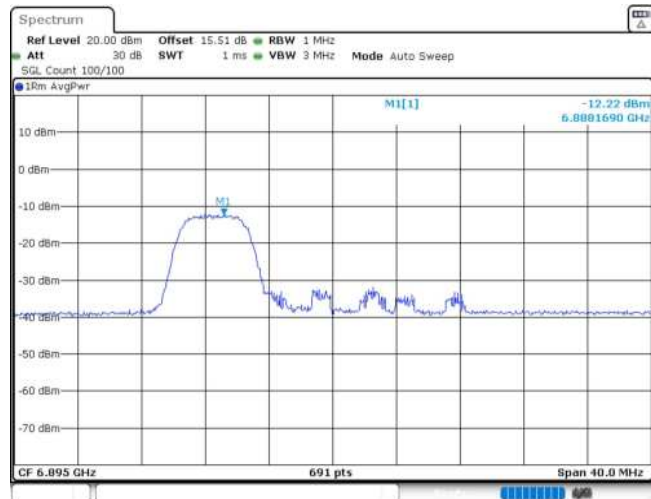
11AX20MIMO_Ant1_6895_52Tone_RU37
