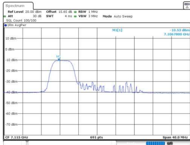
11AX20MIMO_Ant2_7115_52Tone_RU37
