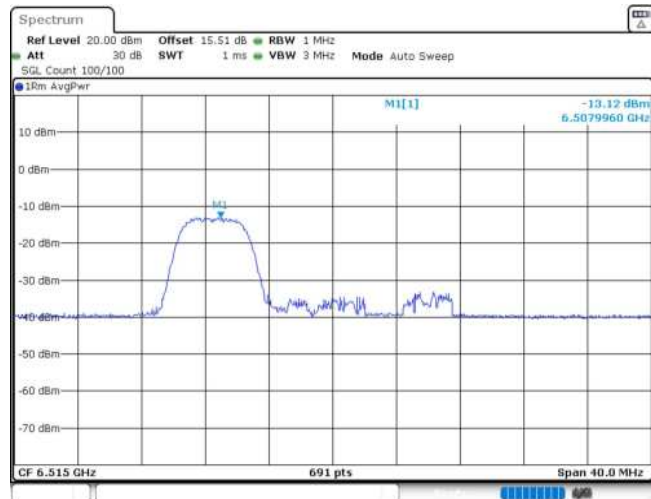
11AX20MIMO_Ant2_6515_52Tone_RU37
