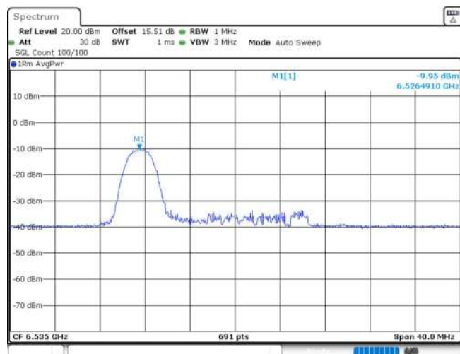
11AX20MIMO_Ant2_6535_26Tone_RU0
