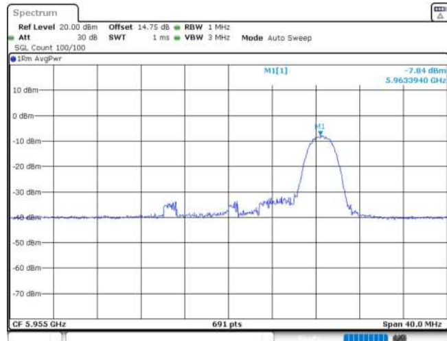
11AX20MIMO_Ant1_5955_26Tone_RU8
