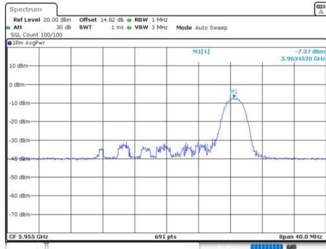
11AX20MIMO_Ant2_5955_26Tone_RU8
