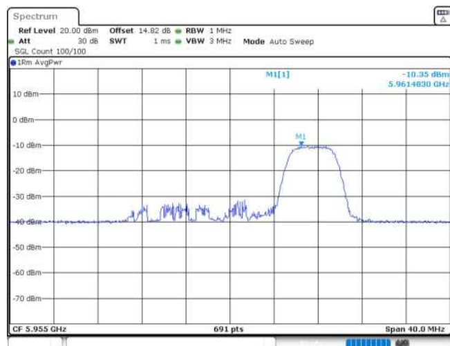
11AX20MIMO_Ant2_5955_52Tone_RU40
