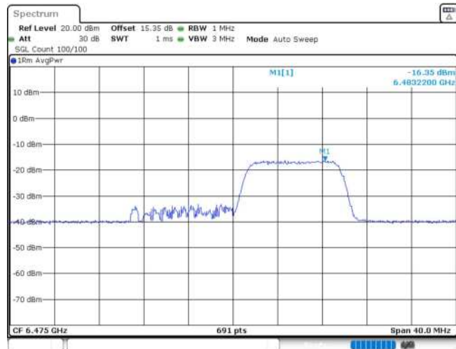
11AX20MIMO_Ant2_6475_106Tone_RU54
