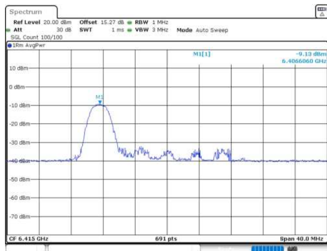
11AX20MIMO_Ant1_6415_26Tone_RU0
