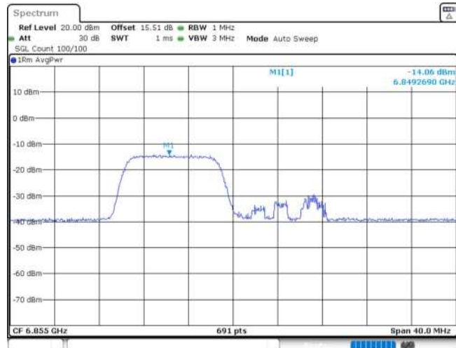
11AX20MIMO_Ant1_6855_106Tone_RU53
