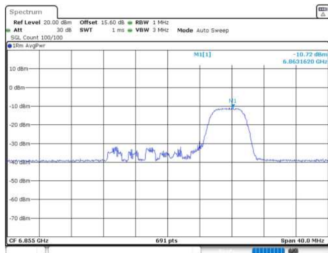
11AX20MIMO_Ant2_6855_52Tone_RU37
