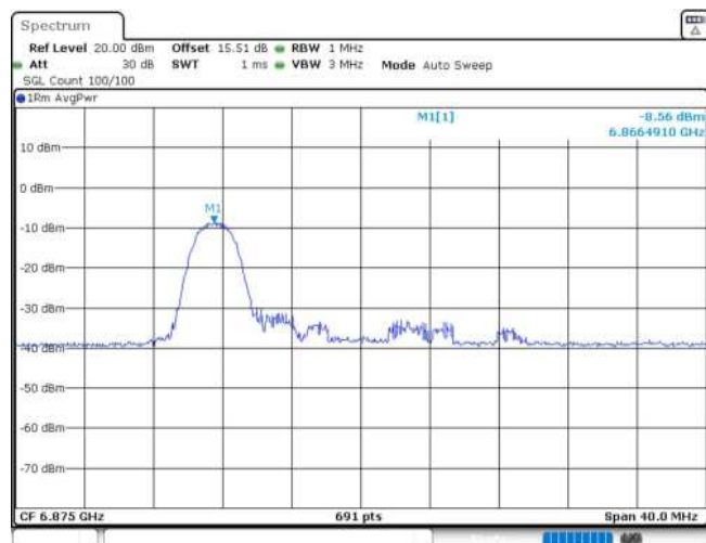
11AX20MIMO_Ant1_6875_26Tone_RU0
