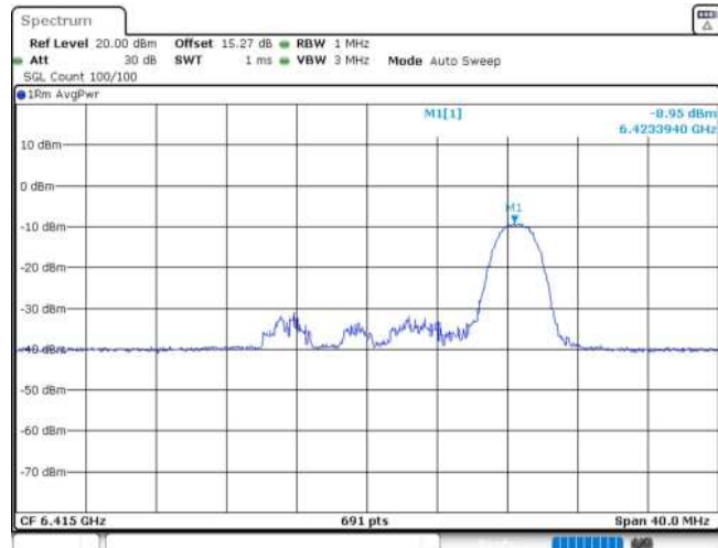
11AX20MIMO_Ant1_6415_26Tone_RU8
