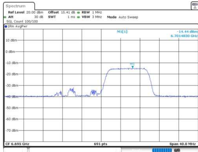
11AX20MIMO_Ant1_6695_106Tone_RU54
