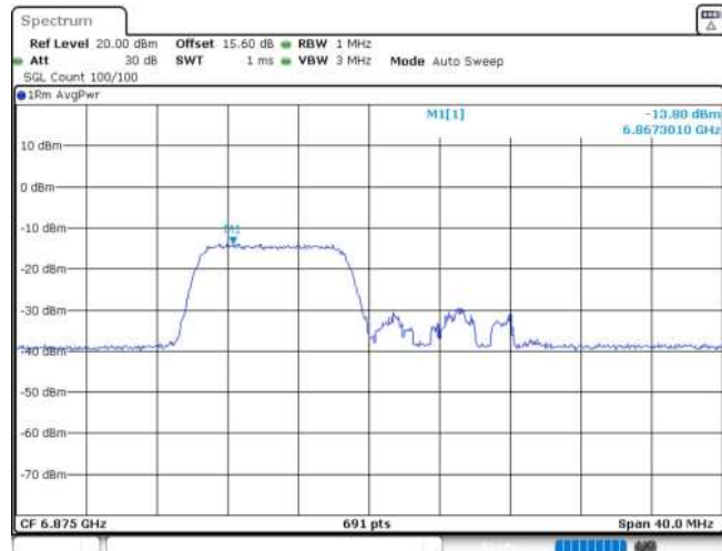
11AX20MIMO_Ant2_6875_106Tone_RU53
