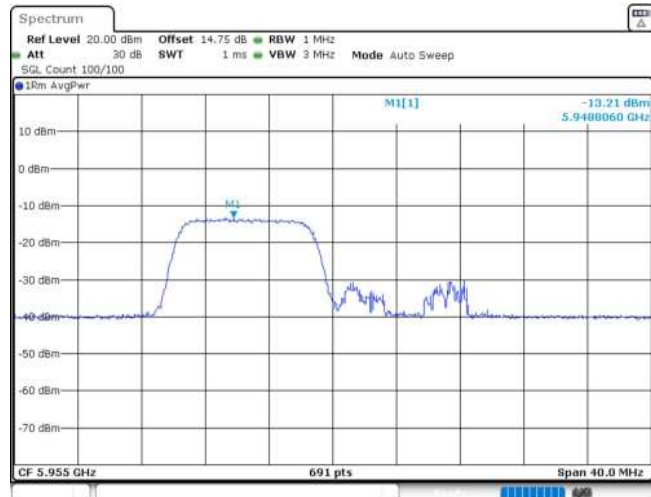
11AX20MIMO_Ant1_5955_106Tone_RU53
