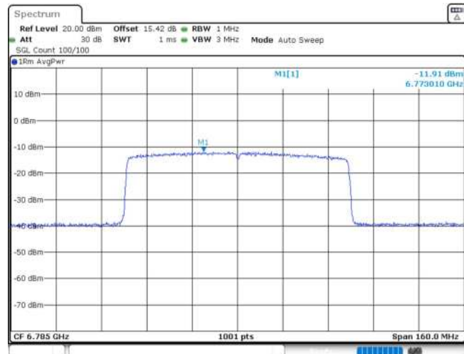
11AX80MIMO_Ant1_6785
