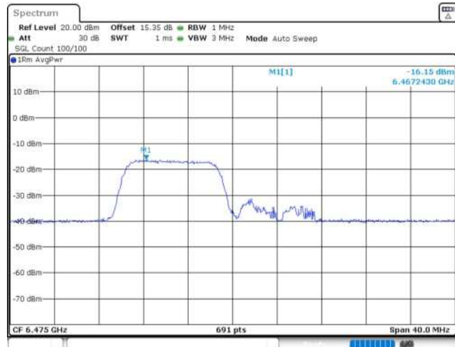
11AX20MIMO_Ant2_6475_106Tone_RU53
