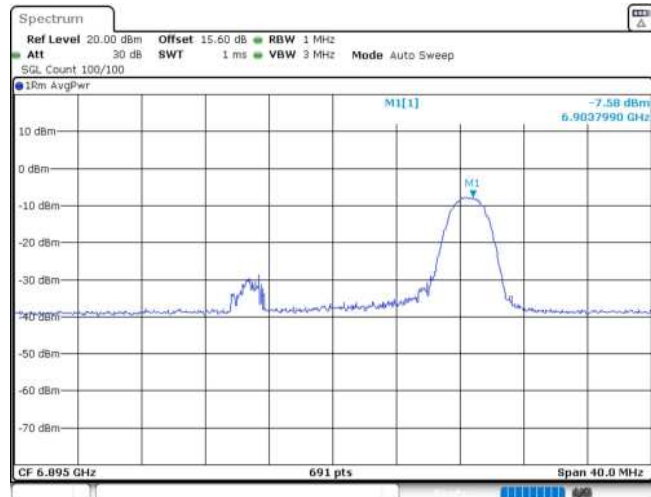
11AX20MIMO_Ant2_6895_26Tone_RU8
