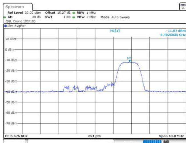
11AX20MIMO_Ant1_6475_52Tone_RU40
