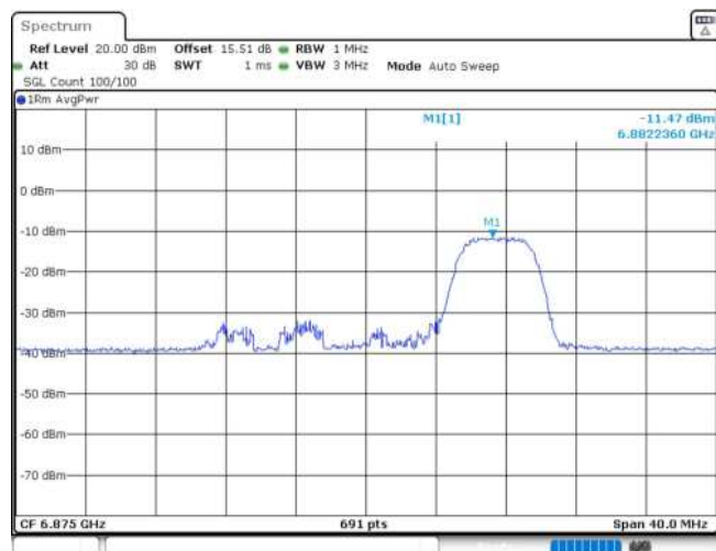
11AX20MIMO_Ant1_6875_52Tone_RU37
