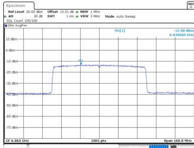
11AX80MIMO_Ant1_6865
