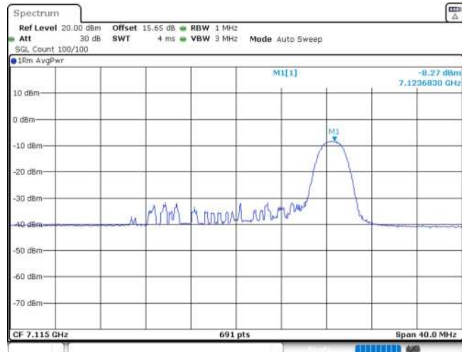
11AX20MIMO_Ant2_7115_26Tone_RU8
