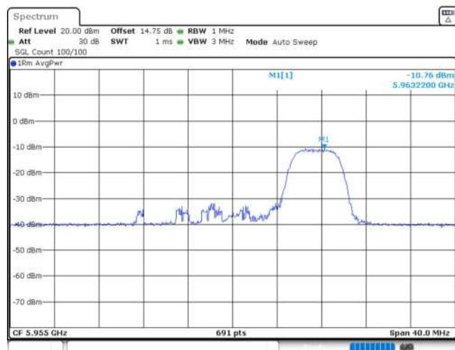
11AX20MIMO_Ant1_5955_52Tone_RU40
