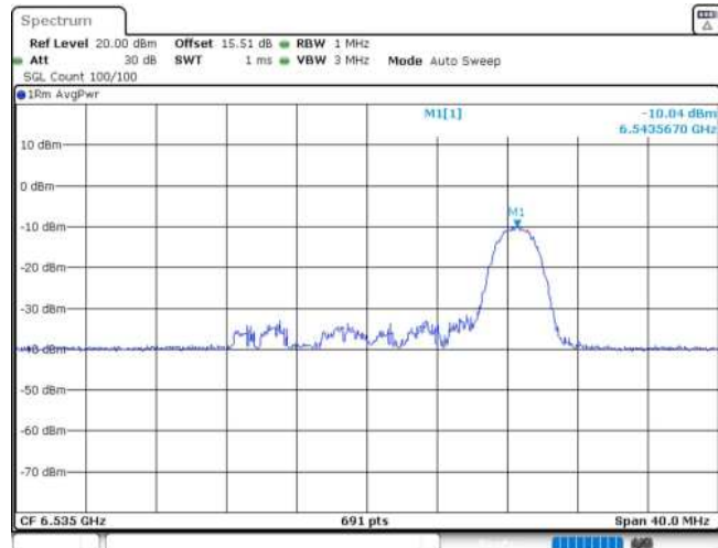
11AX20MIMO_Ant2_6535_26Tone_RU8
