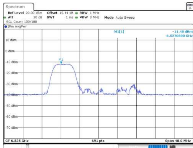
11AX20MIMO_Ant1_6535_52Tone_RU37
