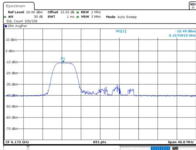
11AX20MIMO_Ant2_6175_52Tone_RU37
