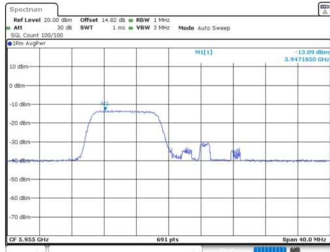
11AX20MIMO_Ant2_5955_106Tone_RU53
