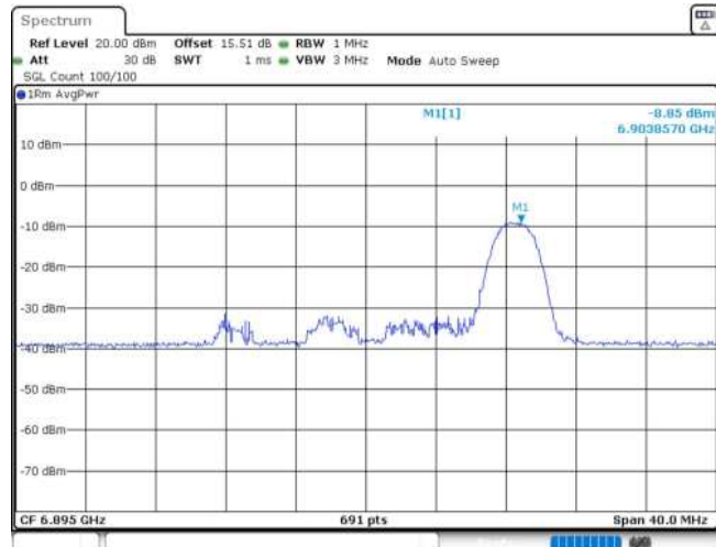
11AX20MIMO_Ant1_6895_26Tone_RU8
