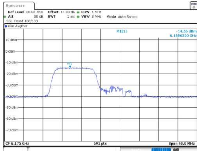
11AX20MIMO_Ant1_6175_106Tone_RU53
