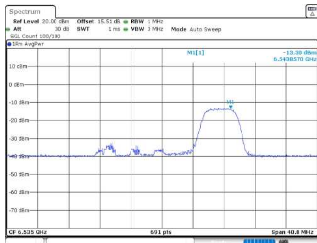
11AX20MIMO_Ant2_6535_52Tone_RU37
