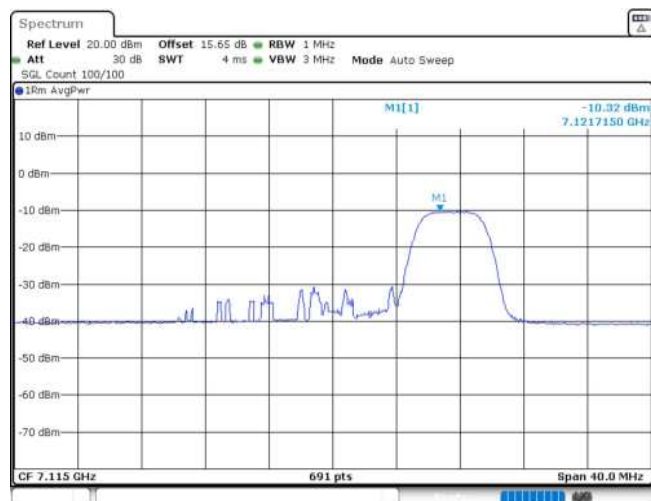
11AX20MIMO_Ant2_7115_52Tone_RU40
