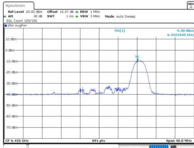
11AX20MIMO_Ant1_6435_26Tone_RU8
