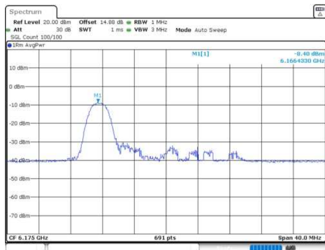
11AX20MIMO_Ant1_6175_26Tone_RU0
