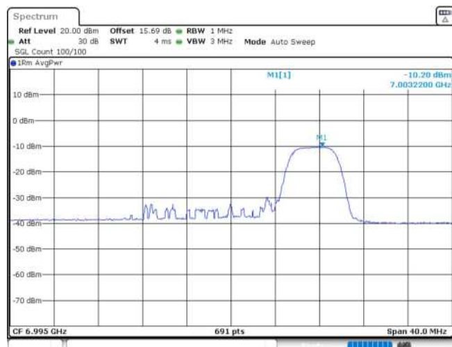
11AX20MIMO_Ant2_6995_52Tone_RU37
