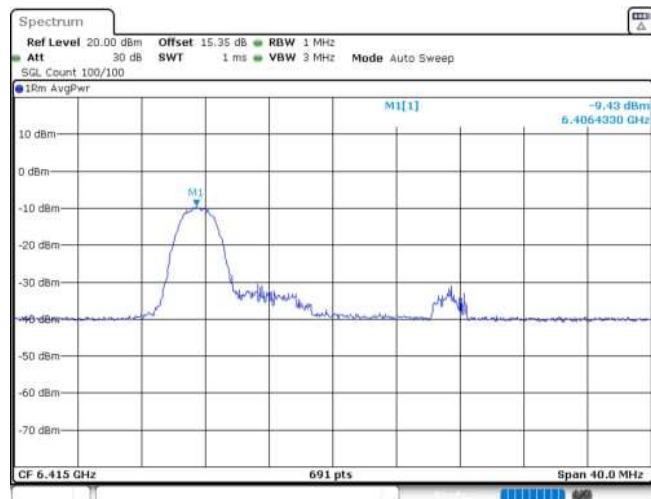
11AX20MIMO_Ant1_6415_106Tone_RU54
