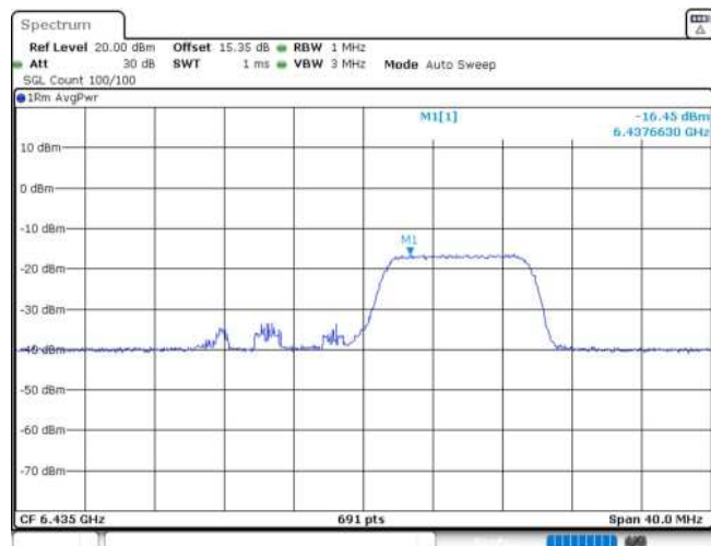
11AX20MIMO_Ant2_6435_106Tone_RU53
