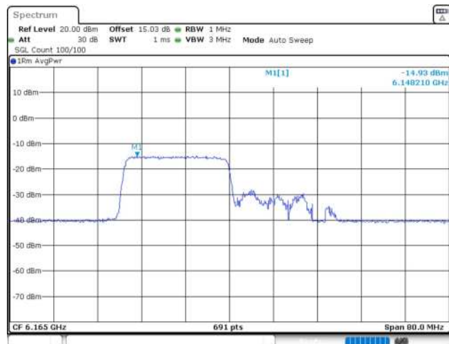
11AX40MIMO_Ant1_6165_242Tone_RU62
