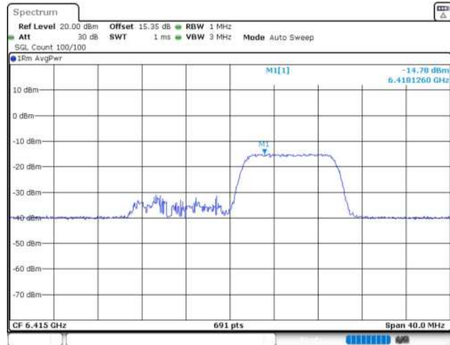
11AX20MIMO_Ant2_6415_106Tone_RU54
