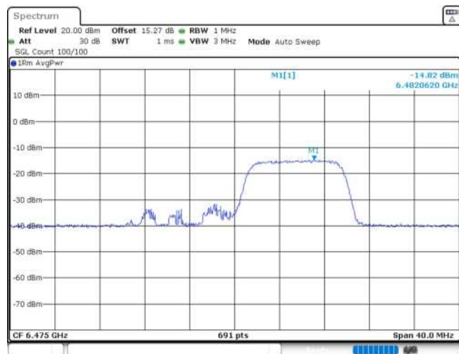
11AX20MIMO_Ant1_6475_106Tone_RU53
