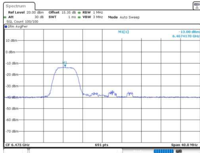
11AX20MIMO_Ant2_6475_52Tone_RU37
