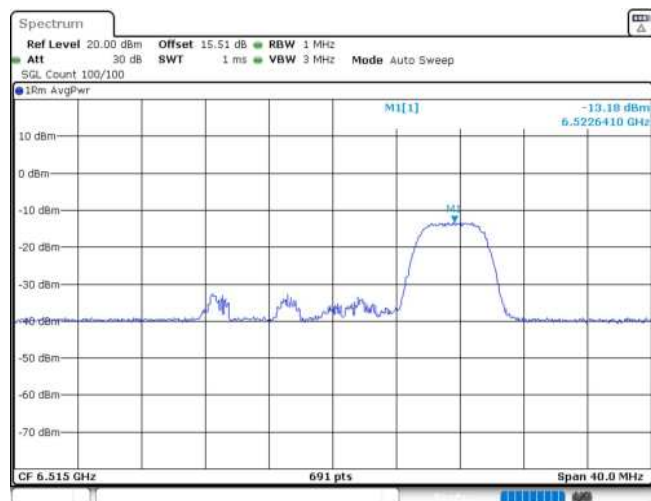
11AX20MIMO_Ant2_6515_52Tone_RU40
