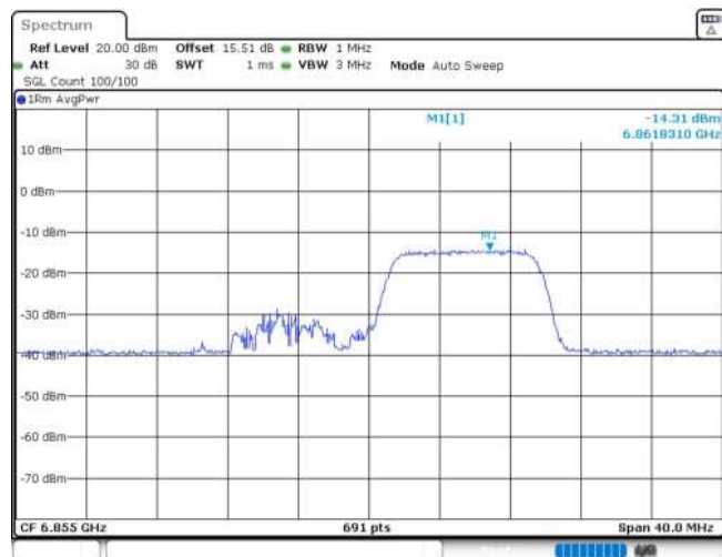
11AX20MIMO_Ant1_6855_106Tone_RU54
