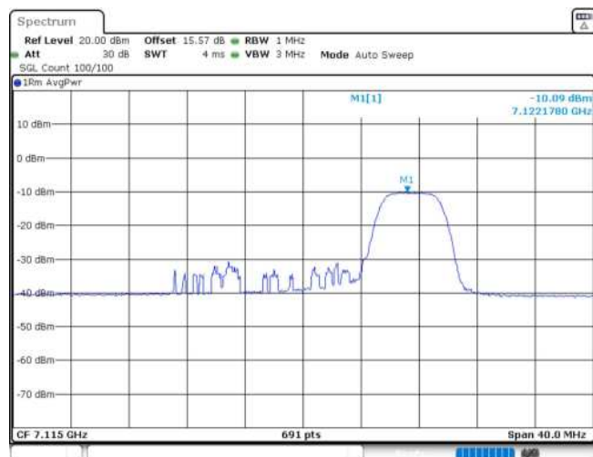
11AX20MIMO_Ant1_7115_52Tone_RU37
