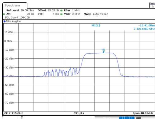
11AX20MIMO_Ant2_7115_106Tone_RU53
