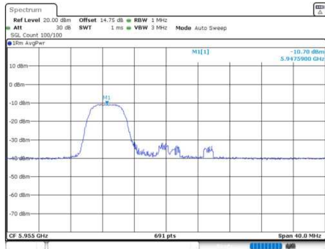
11AX20MIMO_Ant1_5955_52Tone_RU37
