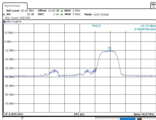
11AX20MIMO_Ant2_6895_52Tone_RU40
