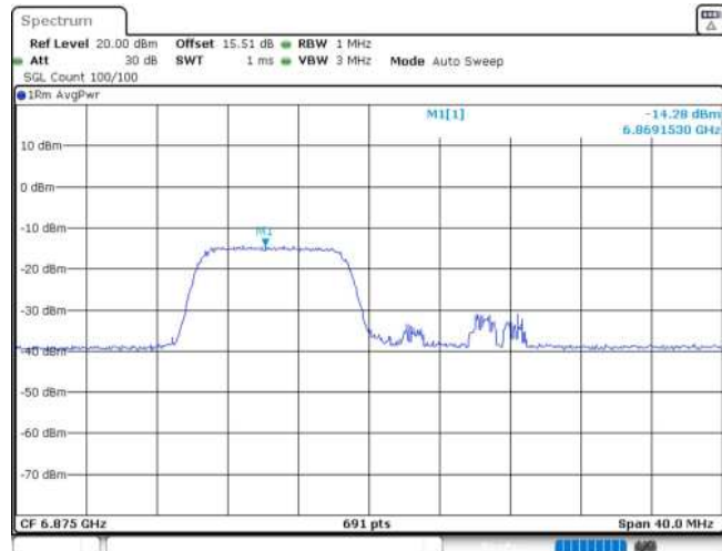
11AX20MIMO_Ant1_6875_106Tone_RU53
