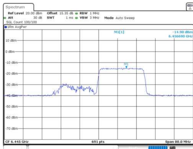
11AX40MIMO_Ant2_6445_242Tone_RU62
