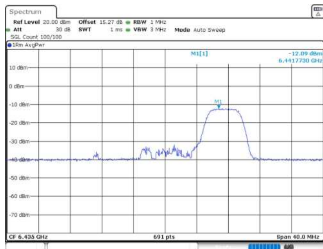
11AX20MIMO_Ant1_6435_52Tone_RU40
