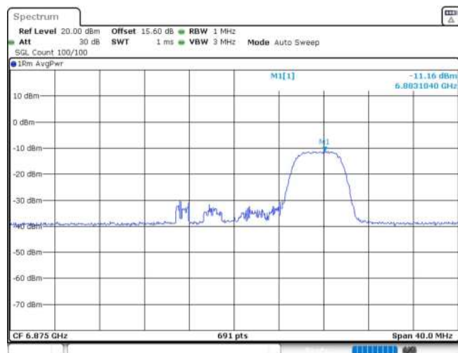
11AX20MIMO_Ant2_6875_52Tone_RU37
