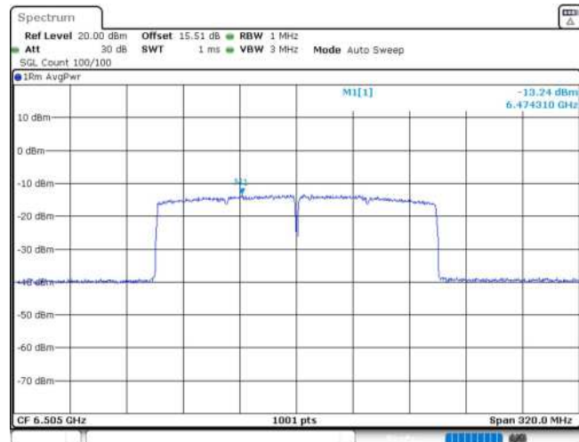
11AX160MIMO_Ant2_6505
