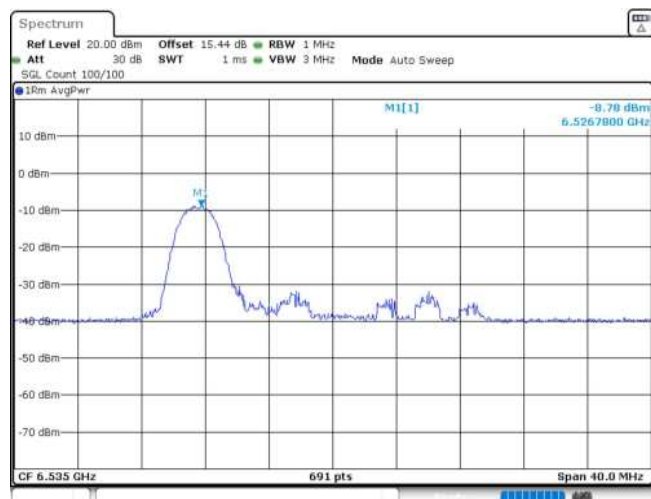
11AX20MIMO_Ant2_6515_106Tone_RU54
