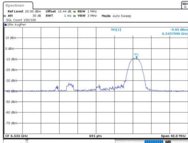
11AX20MIMO_Ant1_6535_26Tone_RU8
