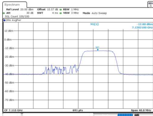
11AX20MIMO_Ant1_7115_106Tone_RU54
