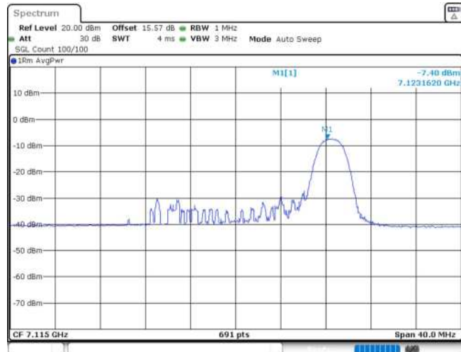
11AX20MIMO_Ant1_7115_26Tone_RU8
