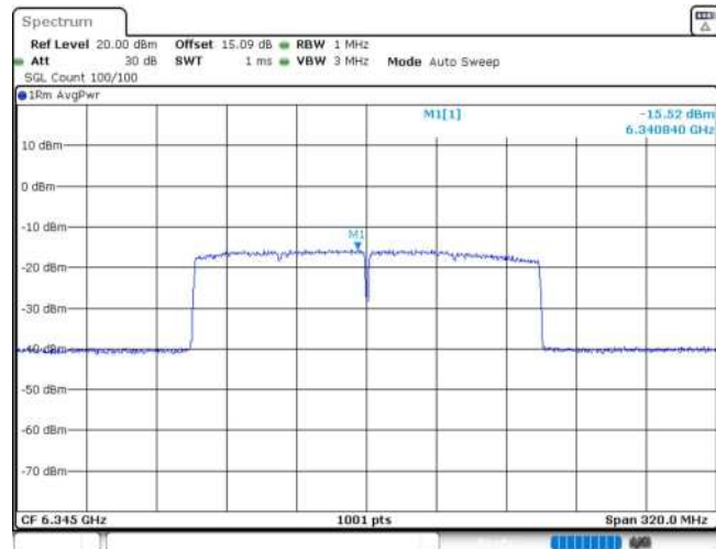
11AX160MIMO_Ant1_6345
