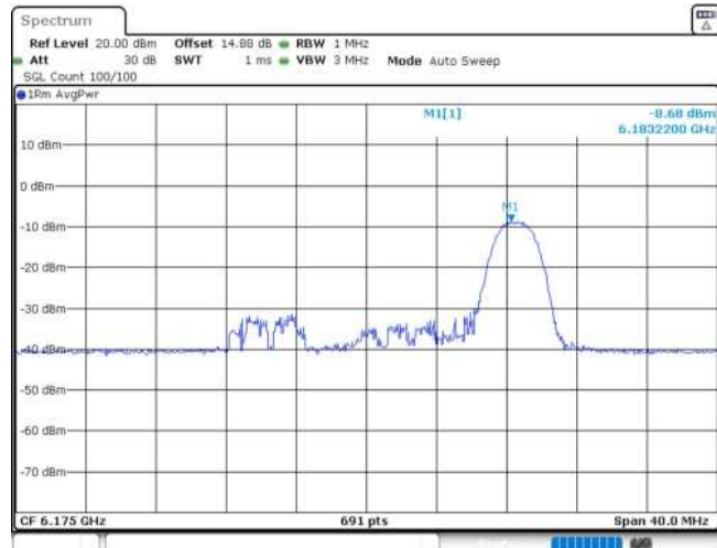
11AX20MIMO_Ant1_6175_26Tone_RU8
