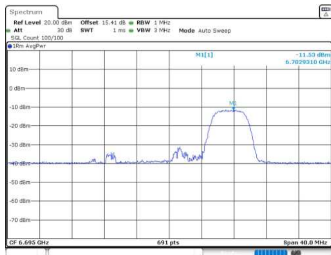
11AX20MIMO_Ant1_6695_52Tone_RU40
