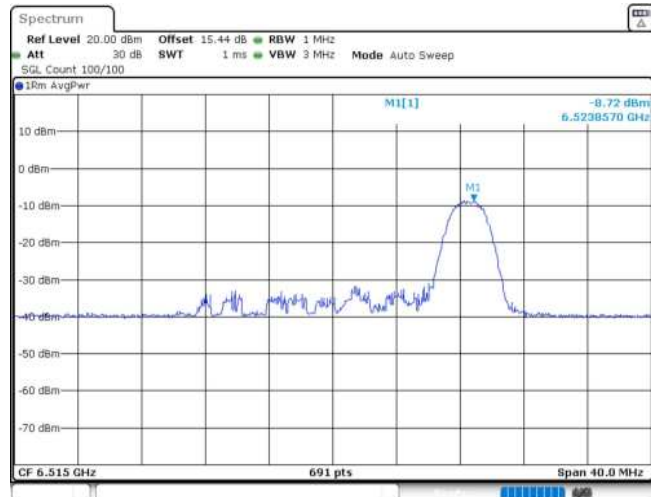
11AX20MIMO_Ant1_6515_26Tone_RU8
