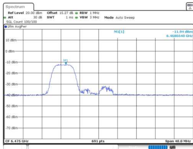
11AX20MIMO_Ant1_6475_52Tone_RU37
