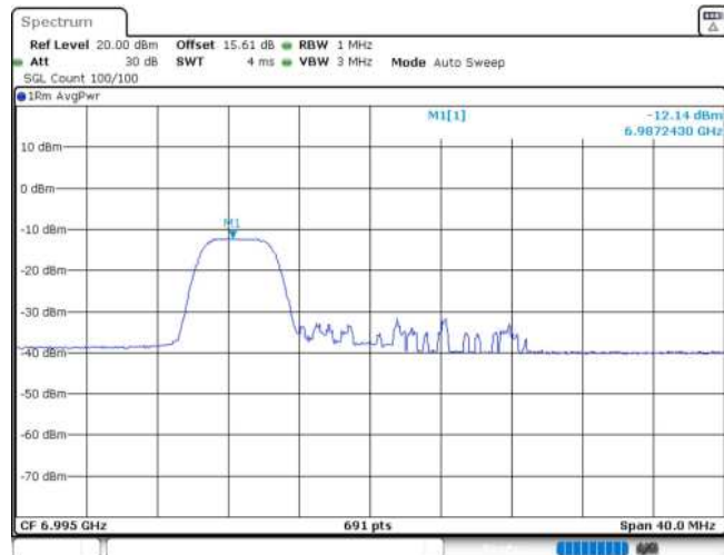
11AX20MIMO_Ant1_6995_52Tone_RU37
