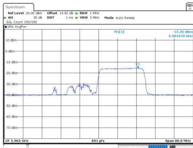
11AX40MIMO_Ant2_5965_242Tone_RU62
