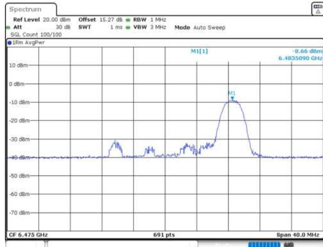
11AX20MIMO_Ant1_6475_26Tone_RU8
