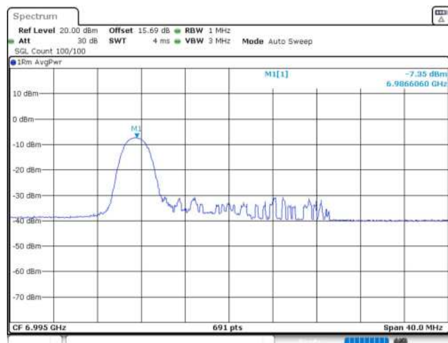
11AX20MIMO_Ant1_6995_106Tone_RU54
