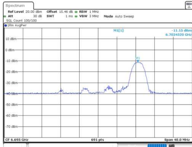
11AX20MIMO_Ant2_6695_26Tone_RU8
