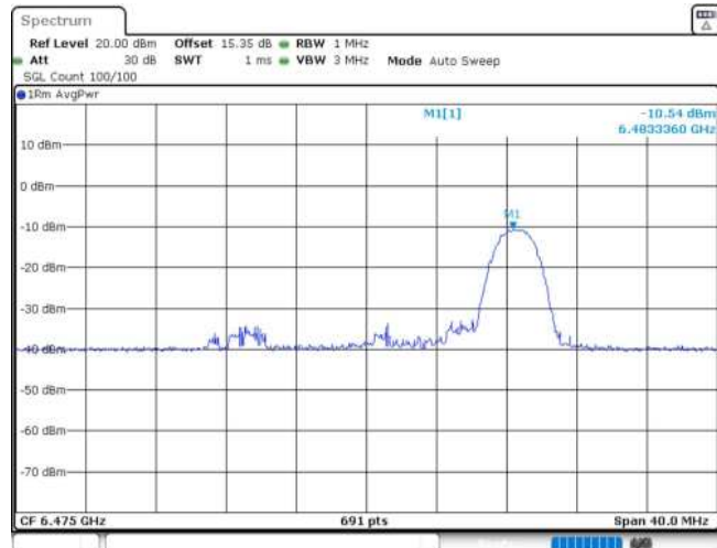
11AX20MIMO_Ant2_6475_26Tone_RU8
