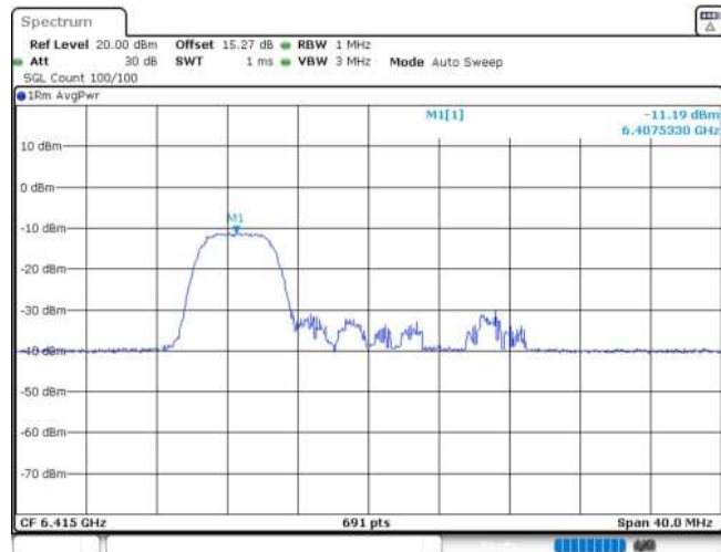
11AX20MIMO_Ant1_6415_52Tone_RU37
