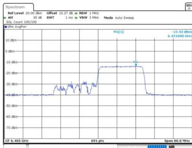
11AX40MIMO_Ant1_6405_242Tone_RU62
