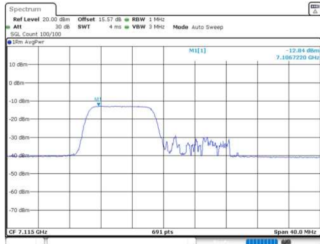
11AX20MIMO_Ant1_7115_106Tone_RU53
