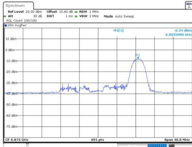
11AX20MIMO_Ant2_6875_26Tone_RU8
