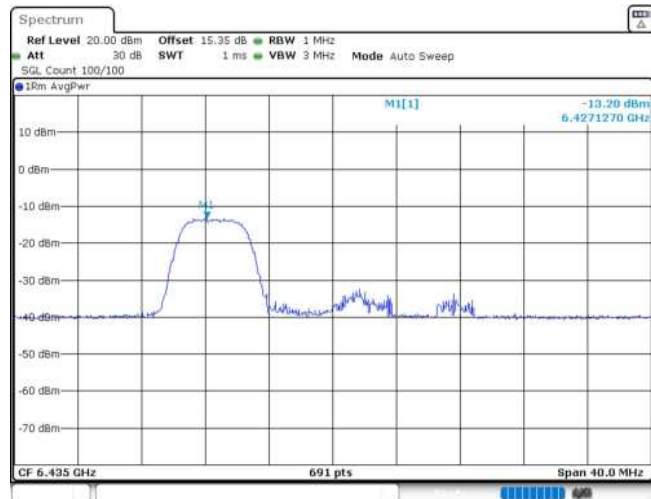
11AX20MIMO_Ant2_6435_52Tone_RU37
