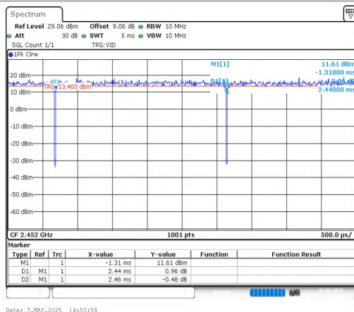
NTNV-11AX40MIMO-Ant1-2452
