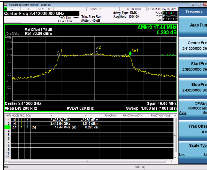
11N/AC 20MIMO_Ant2_2412
