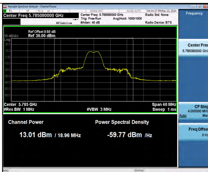
11AX20MIMO Ant1 5785 52Tone RU38
