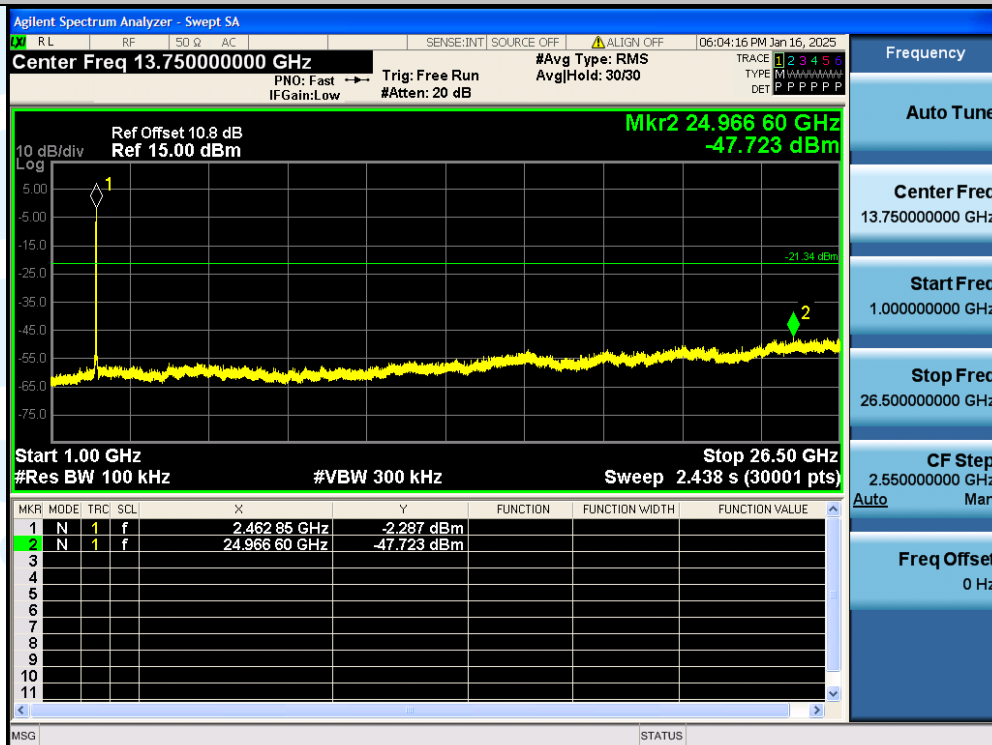
11G-Ant1-2462MHz-1000~26500MHz-PASS
