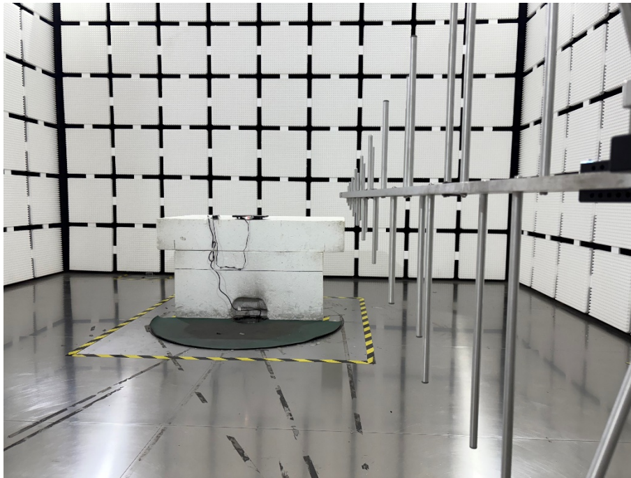
30MHz-1GHz-BT/WIFI
