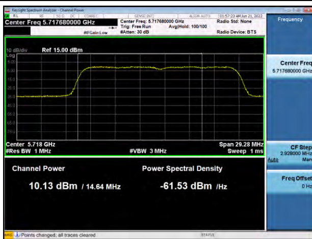
5720 MHz : Chain 2
