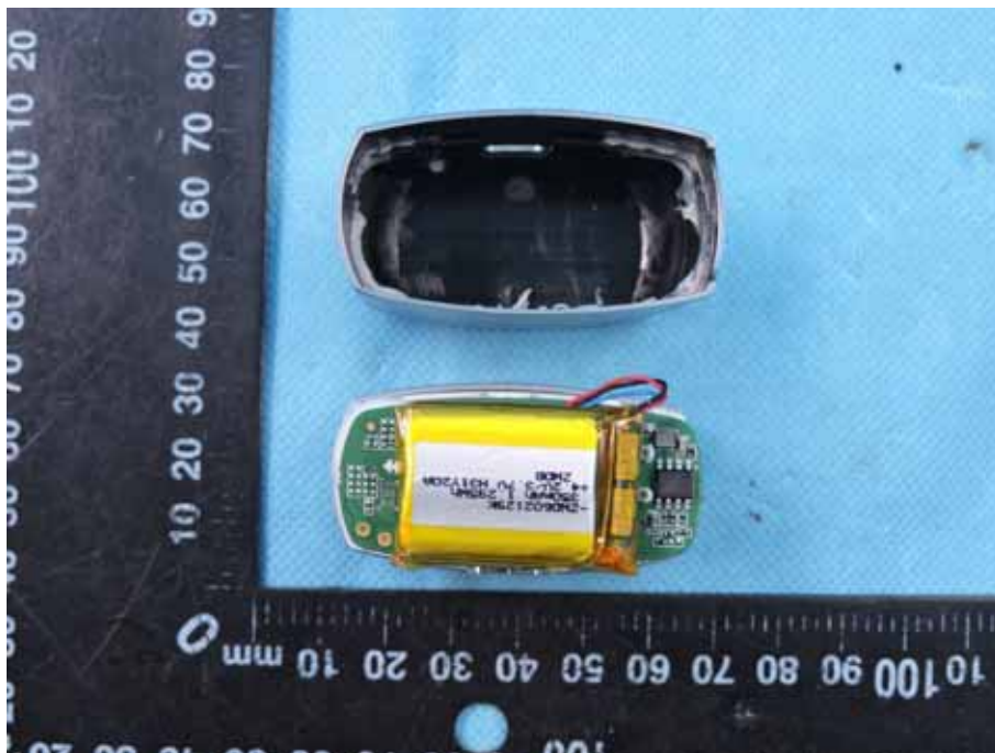
Model: Klipsch T5 II True Wireless
