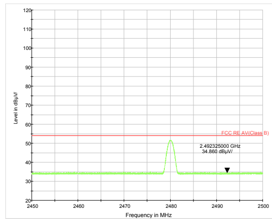
BLE Channel 39 Average
