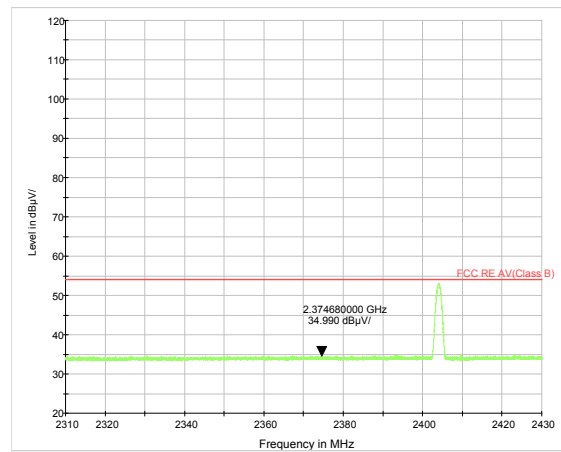
BLE Channel 0 Average
