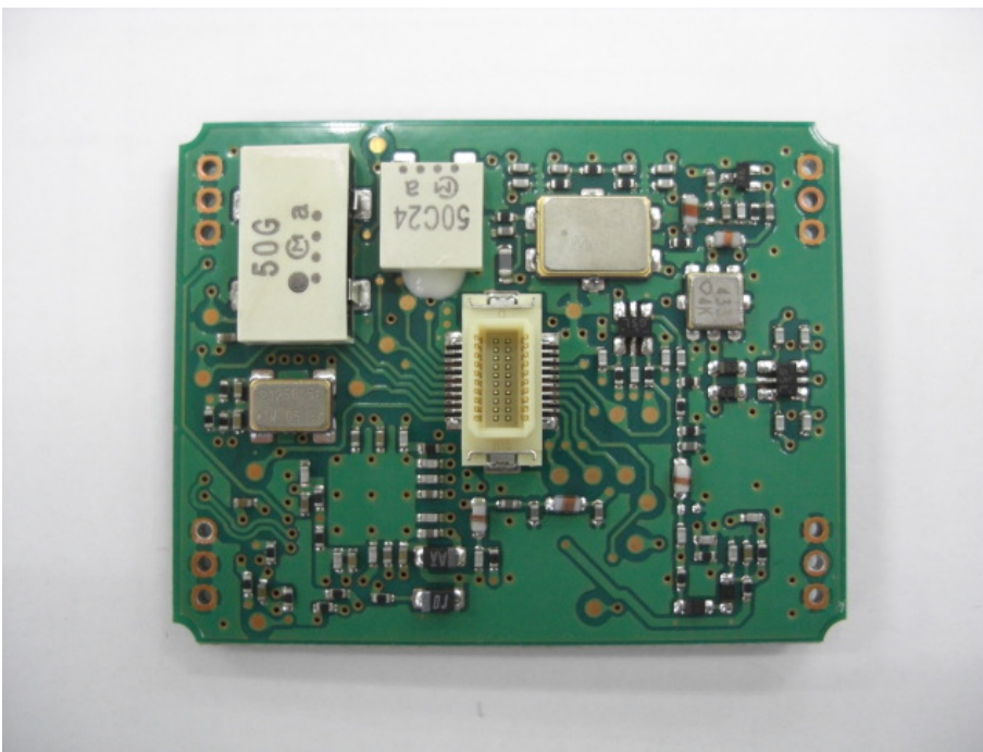
RF-module side-C
