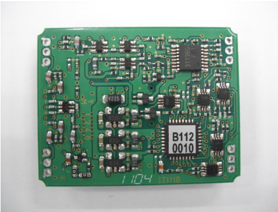
RF-module side-S
