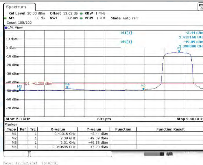
11N20MIMO_Ant1_Low_2412_AV
