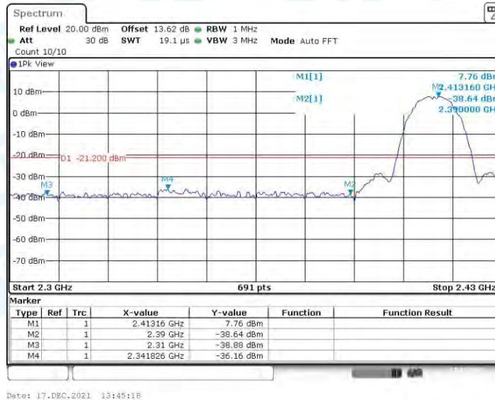
11B-CDD_Ant1_Low_2412_Peak
