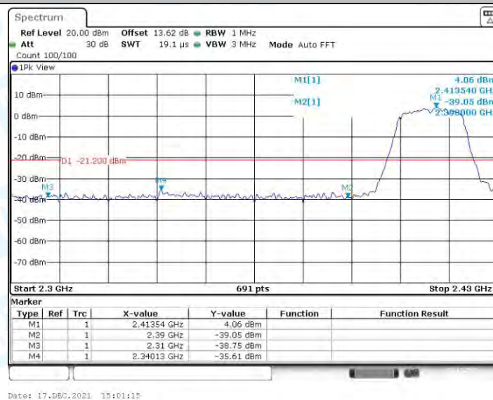
11N20MIMO_Ant1_Low_2412_Peak
