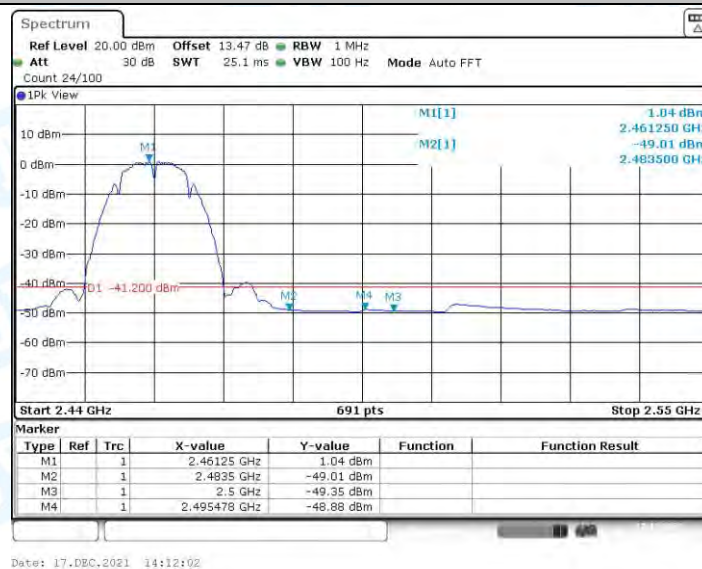
11B-CDD_Ant1_High_2462_AV
