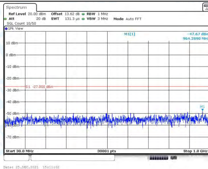
11AC80MIMO_Ant2_5210_30~1000
