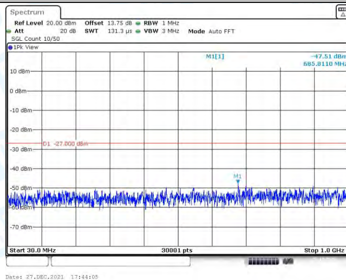
11AC40MIMO_Ant2_5310_30~1000
