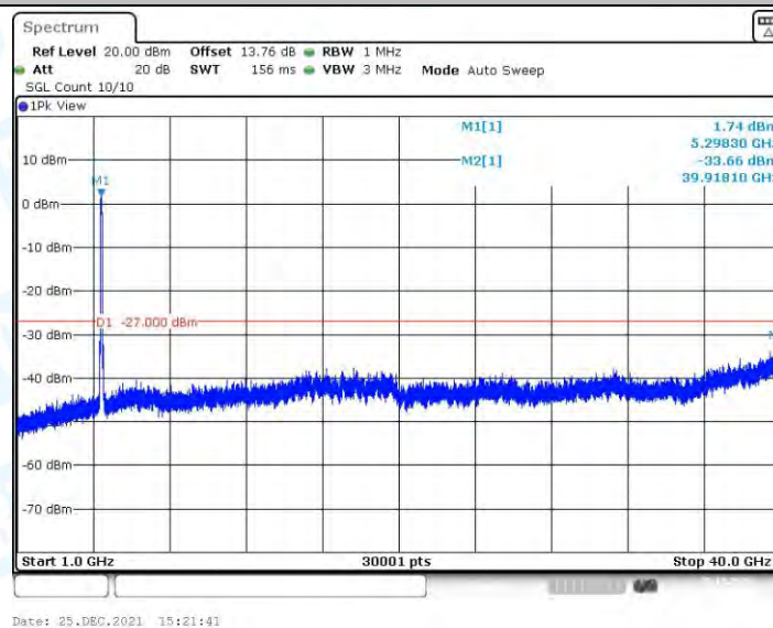
11AC80MIMO_Ant1_5290_1000~40000
