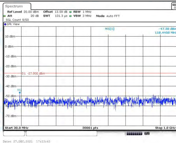
11AC40MIMO_Ant2_5190_30~1000
