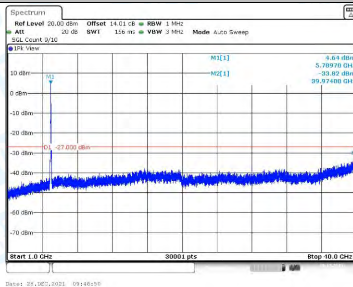
11AC40MIMO_Ant2_5795_1000~40000
