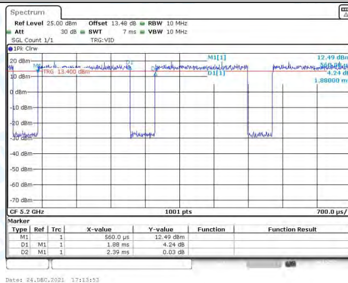
11N20MIMO_Ant1_5200
