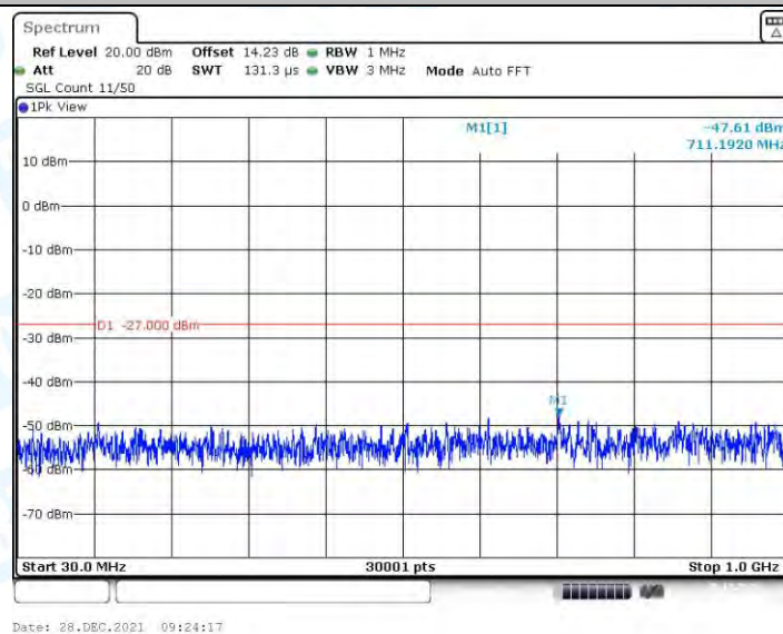
11AC40MIMO_Ant2_5670_30~1000
