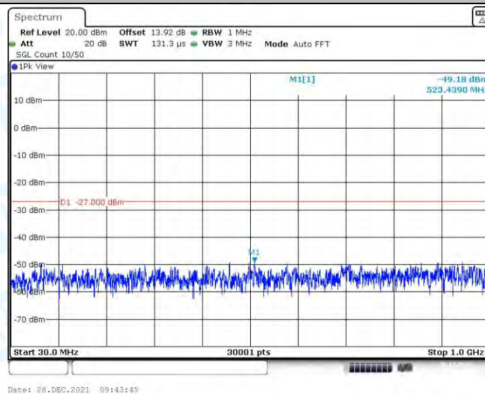
11AC40MIMO_Ant1_5795_30~1000
