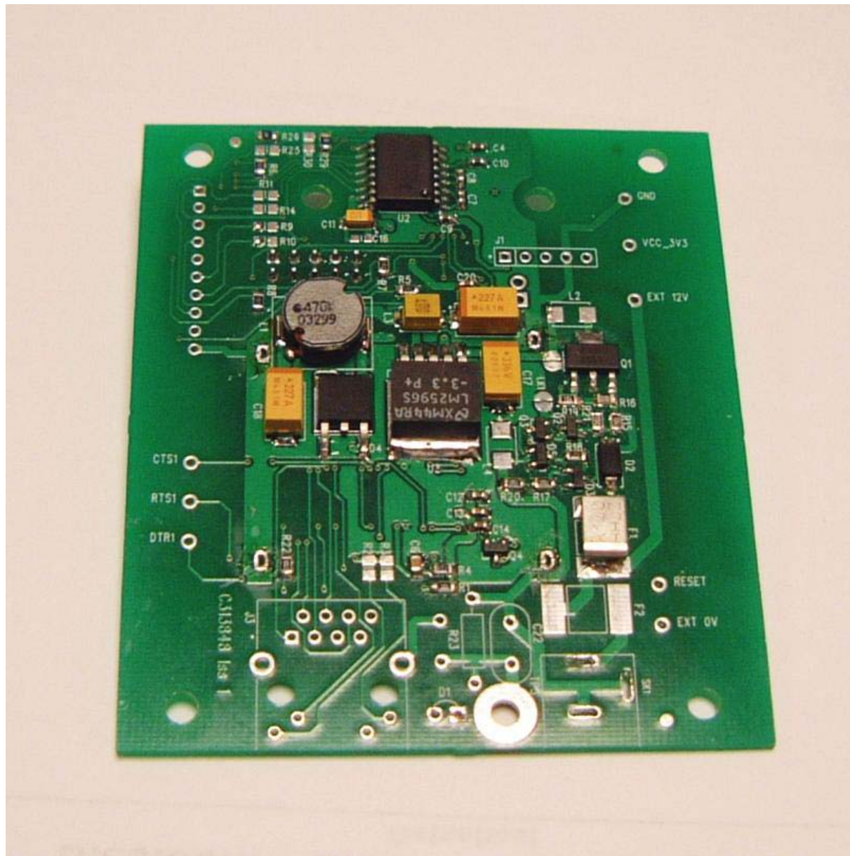
Fig. 3 Wi-Fi Module PCB – Bottom
