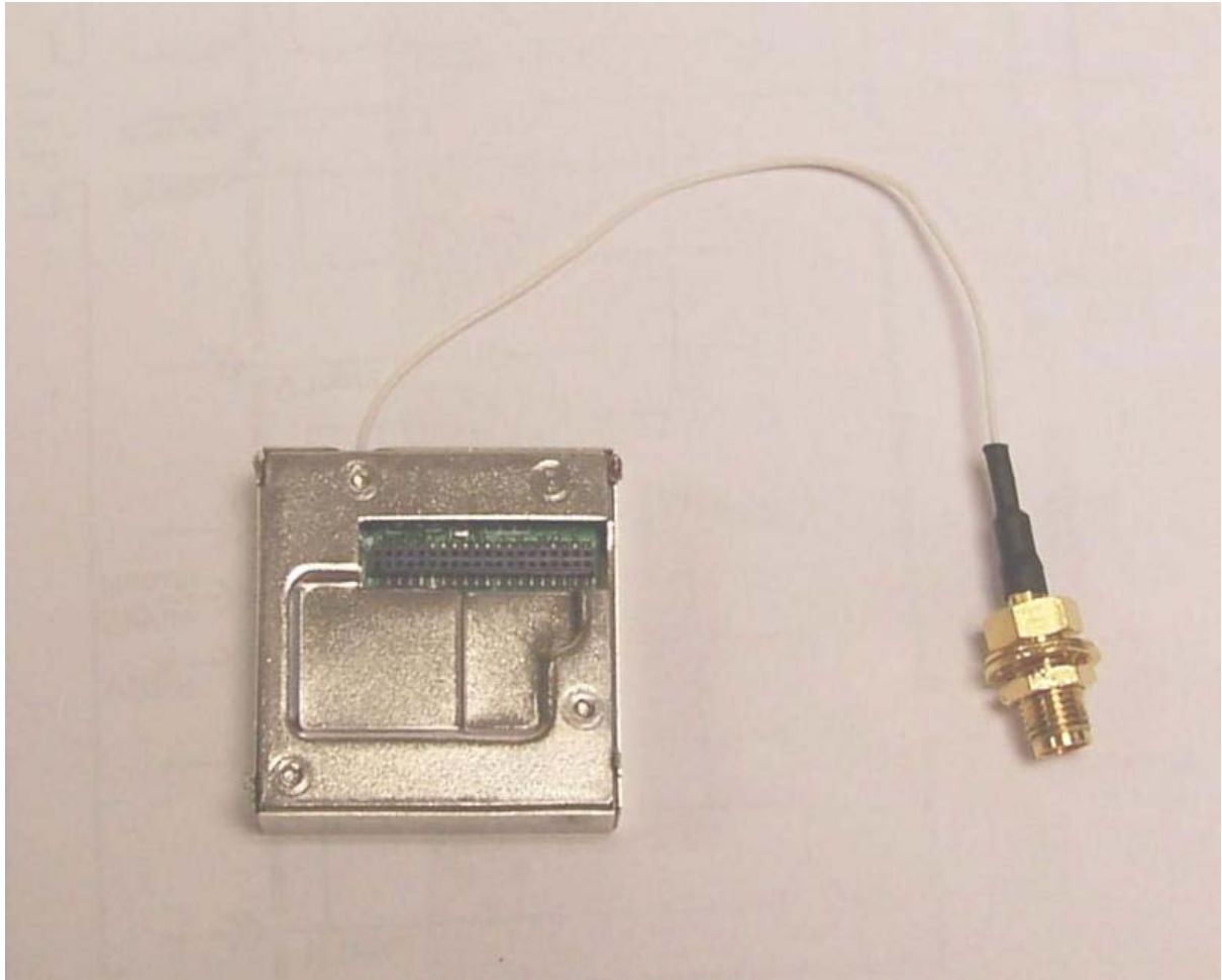
Fig. 5 RF Module - Bottom
