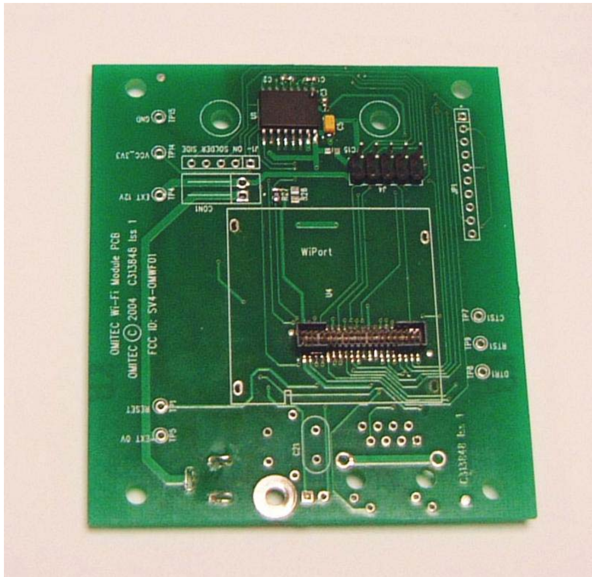
Fig. 2 Wi-Fi Module PCB – Top – RF module removed
