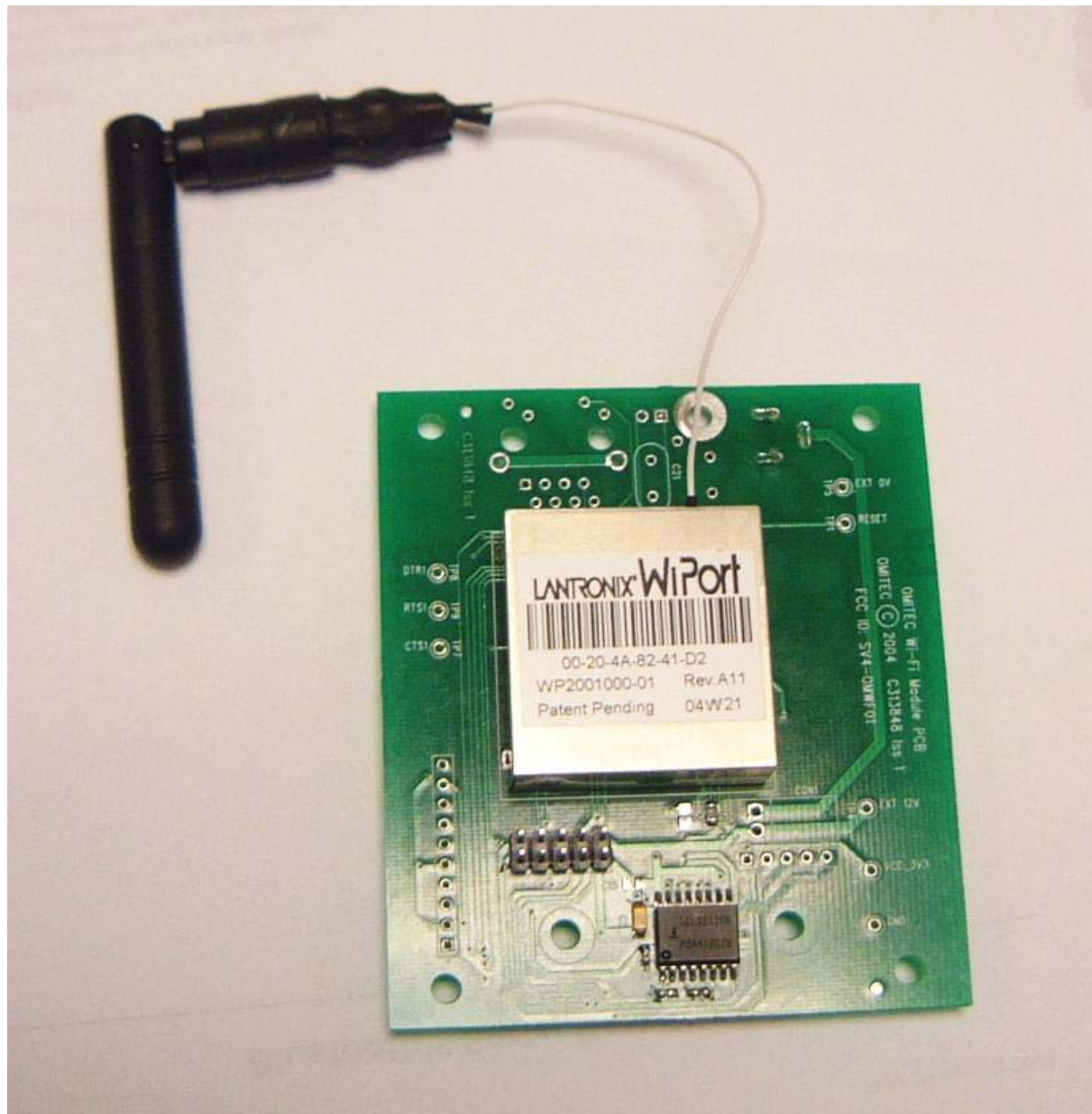
Fig. 1 Wi-Fi Module PCB – Top
