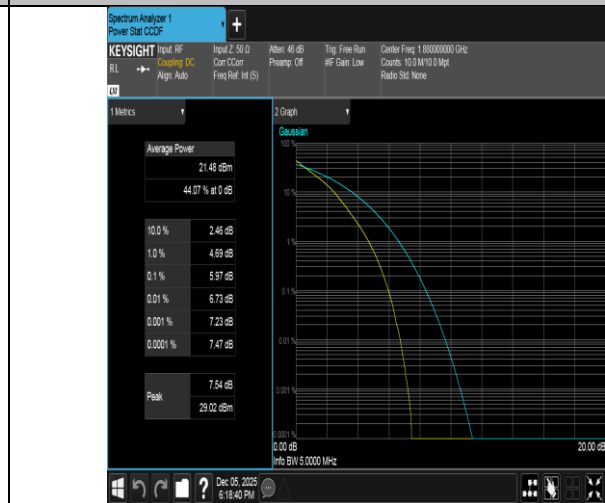
Band2-5MHz-QPSK-18900-25RB#0-PASS
