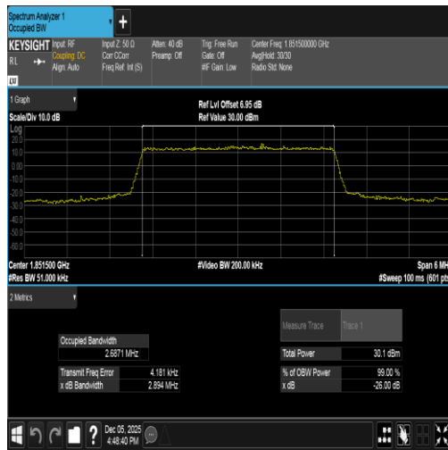
Band2-3MHz-QPSK-18615-15RB#0-PASS
