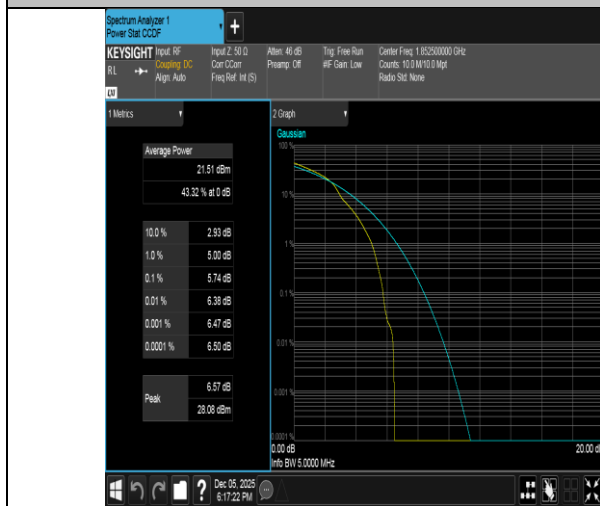
Band2-5MHz-16QAM-18625-1RB#0-PASS
