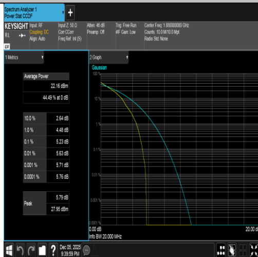
Band2-20MHz-QPSK-18900-1RB#0-PASS
