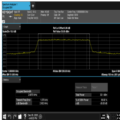
Band2-3MHz-QPSK-18900-15RB#0-PASS
