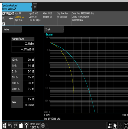
Band2-10MHz-QPSK-18900-1RB#0-PASS
