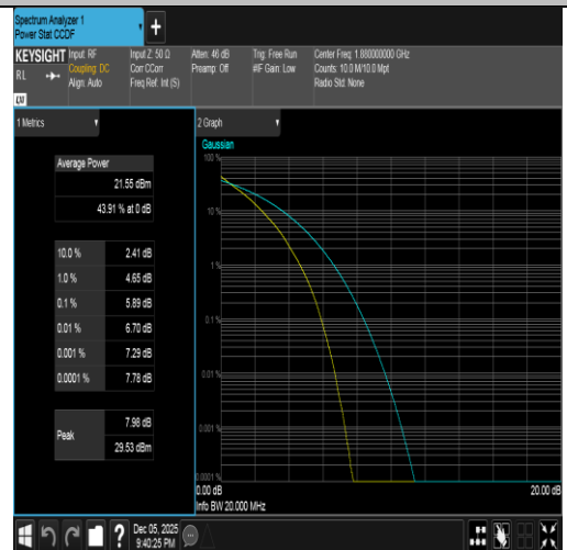
Band2-20MHz-QPSK-18900-100RB#0-PASS
