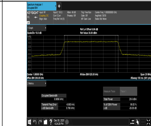
Band2-10MHz-16QAM-18900-50RB#0-PASS
