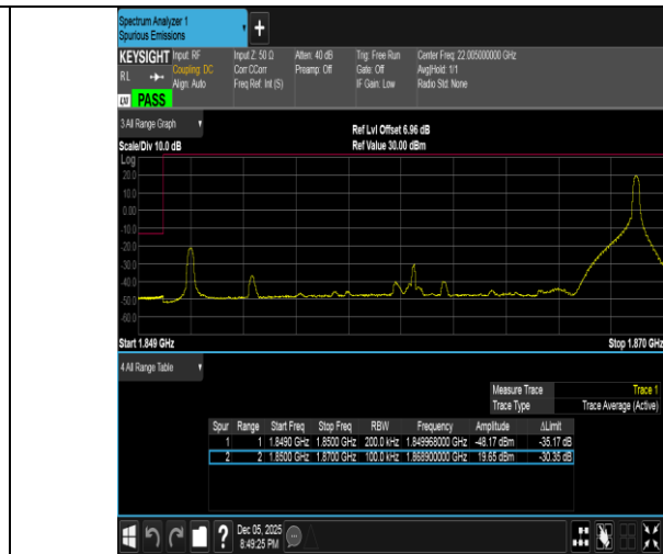
Band2-20MHz-QPSK-18700-1RB#99-PASS
