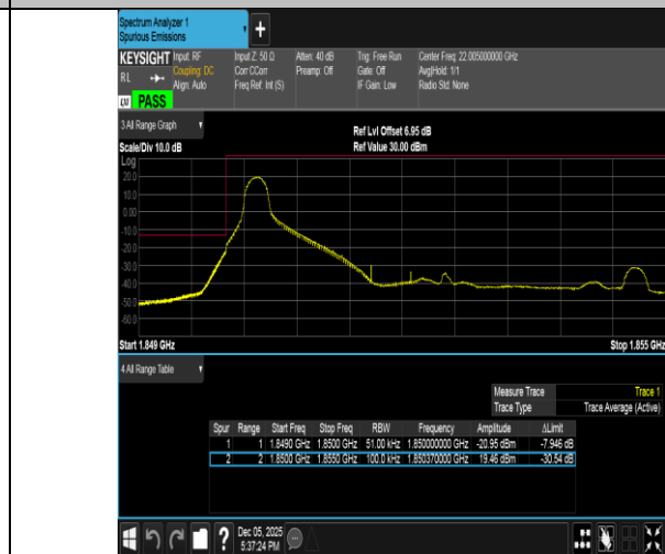
Band2-5MHz-16QAM-18625-1RB#0-PASS
