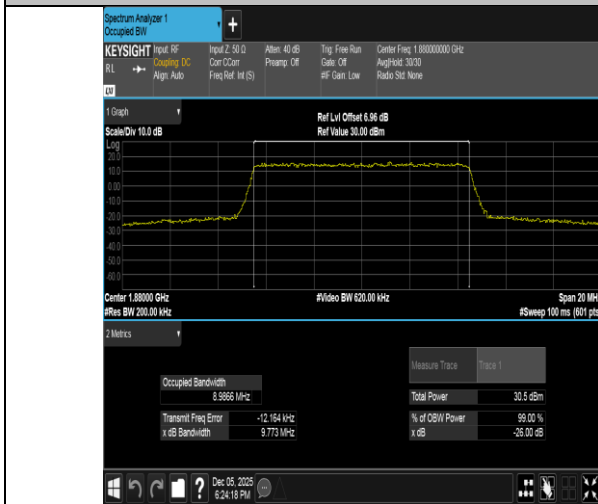
Band2-10MHz-QPSK-18900-50RB#0-PASS
